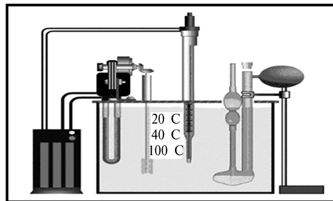
5.5- rasm. Moylarning qovushqoqligini aniqlash asbobi
