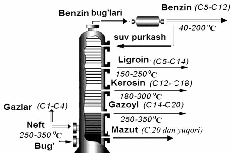
1.3 -rasm. Rektifikatsiyalash kolonnasi qurilmasining sxemasi.
