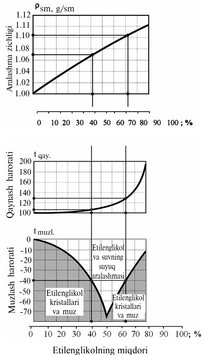
8.2-rasm. Etillenglikol va suvning muzlash, qaynash harorati.
