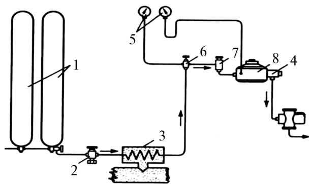
4.2-rasm. Siqilgan gaz uzatish sistemasining sxemasi:
