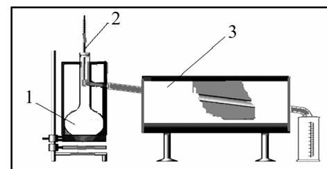
2.5- rasm. Yonilg'ilarni fraksion tarkibini aniqlaydigan qurilma.
