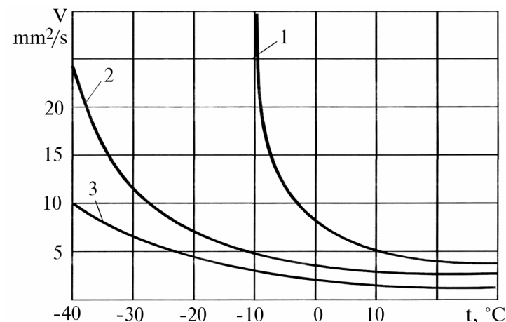
3.1-rasm. Dizel yonilg'isi qovushqoqligi(v)ning, harorat (t°C)ga bog'liqligi: 1-yozgi; 2-qishki; 3-shimoliy.
