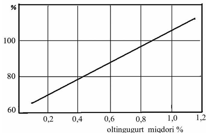
rasm. Yonilg'i tarkibidagi oltinugurt miqdorini porshen 1.1 halqalari yeyilishiga ta'siri
