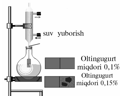
3.4- rasm. Yonilg'i tarkibidagi oltingugurt miqdorini aniqlash asbobi.
