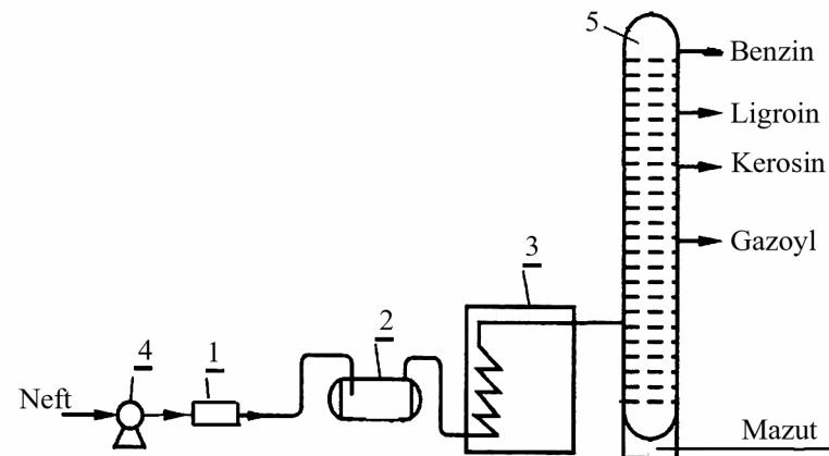
1.4-rasm. Bir marta bug'latishli neftni haydash qurilmasi: 1-issiqlik almashtirgich; 2- suv va loy ajratgich; 3-pech; 4- nasos; 5- rektifikatsion kolonna (minora).
