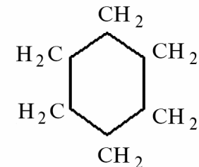
siklogeksan
