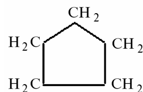
siklopentan
