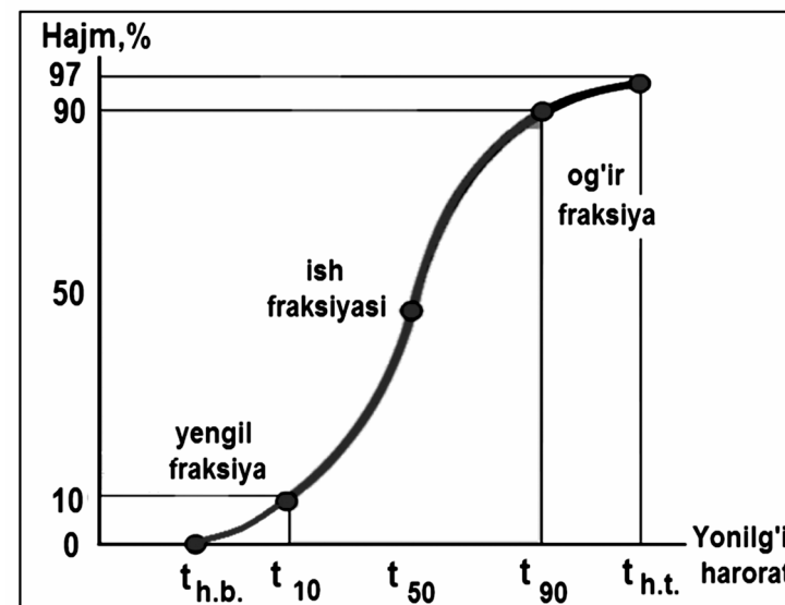
2.6-rasm. Benzinning fraksion tarkibi egri chiziq'i
