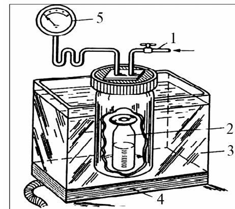
2.13 -rasm. Benzinning induksion davrini aniqlash asbobi:
