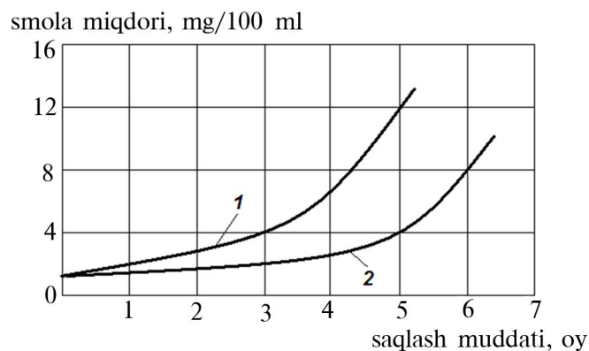
2.14 rasm. Benzinni saqlash mobaynida smolali birikmalarning hosil bo'lishi: 1- to'la to'ldirilgan idish, 2- 50% to'ldirilgan idish.
