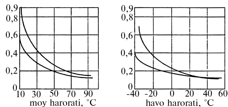
6.1-rasm. Moy harorati va havo haroratining tishli ilashmalar yeyilishga ta'siri.
