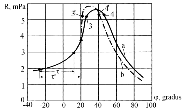
3.6.-rasm. Dizel yonilg'ilarining yoyilgan indikator diagrammasi: a-yumshoq ishlash; v-qattiq ishlash.
