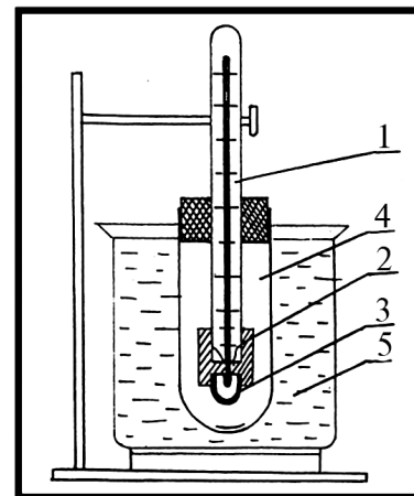
7.1.-rasm. Tomchilash haroratsini aniqlash asbobi.
