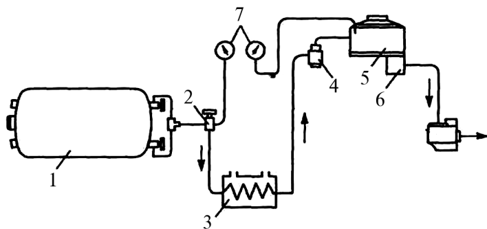
4.1-rasm. Suyultirilgan gaz uzatish sistemasining sxemasi:
