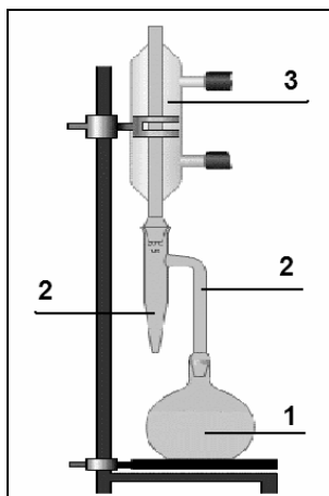
3.5- rasm. Yonilg'i tarkibidagi suvning miqdorini aniqlash asbobi. 1-kolba, 2-suv yig'gich, 3-sovutgich.
