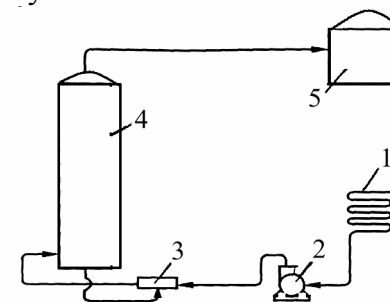
1.6-rasm. Benzinni ishqor bilan tozalash sxemasi:
