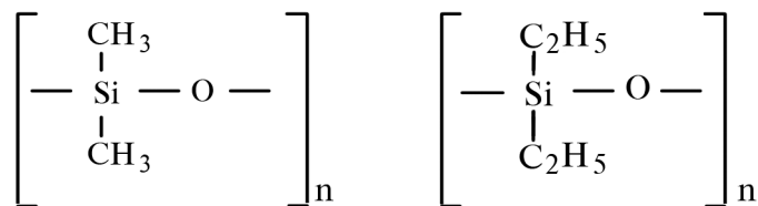
Metilpolisiloksan
