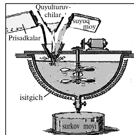
7.1. rasm. Plastik surkov moylarini tayorlash jarayoni.
