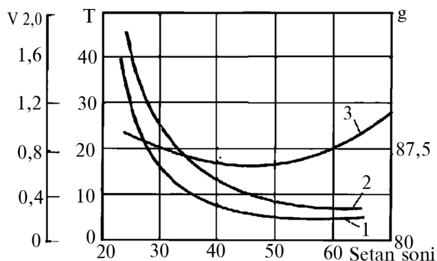
3.9-rasm. Setan sonini o'zgarishini dizel dvigateling parametralariga bog'liqlik grafiqi:
