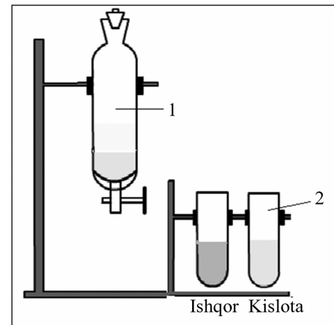
2.2- rasm. Yonilg'i tarkibidagi kislota va ishqorlarni aniqlash asbobi 1-ajratish asbobi. 2-probirkalar.
