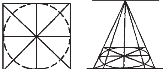
4- a rasm. Aylana perspektivasi.
