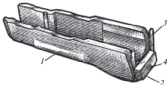
91-rasm. Stvol osti qoplamasi (dastasi): 1—barmoqlar uchun joy; 2—boʻrtma; 3—yassi prujina; 4—shompol uchun teshik.
