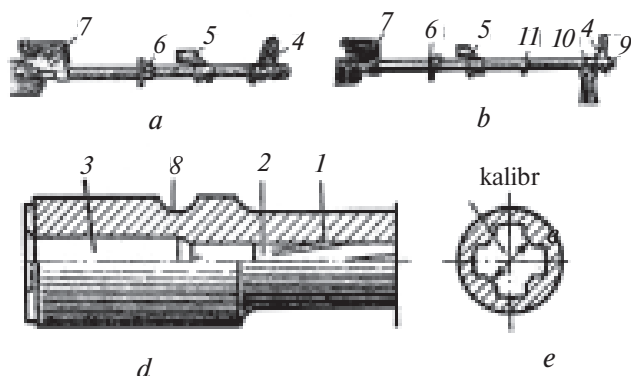
81-rasm. Stvol:
