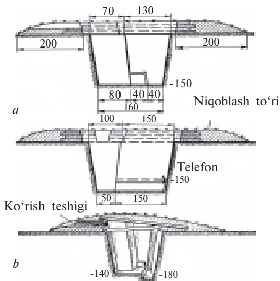
51-rasm. Kuzatuv punkti:
