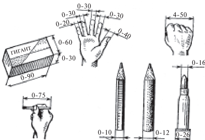
59-rasm. Qo'l ostidagi predmetlardan burchakning minglar kattaligini o'lchashda foydalanish.
