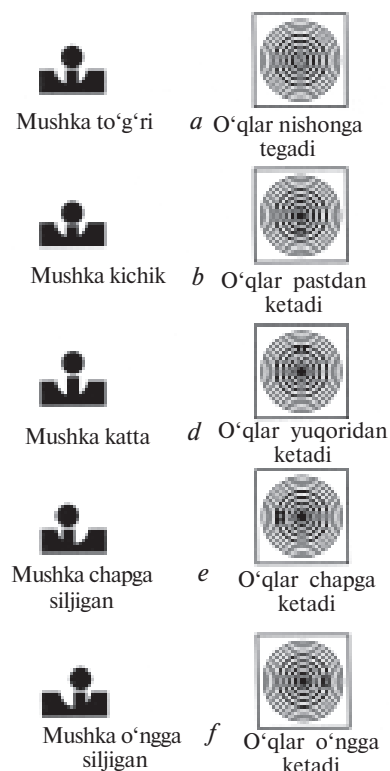
124-rasm. Toʻgʻri moʻljallash va moʻljallash vaqtidagi xatoliklar: a—mushkani toʻgʻri olib, moʻljallangan nuqtaga toʻgʻrilash; b—mushka kichik; d—mushka katta; e—mushka chapga siljigan; f—mushka oʻngga siljigan.
