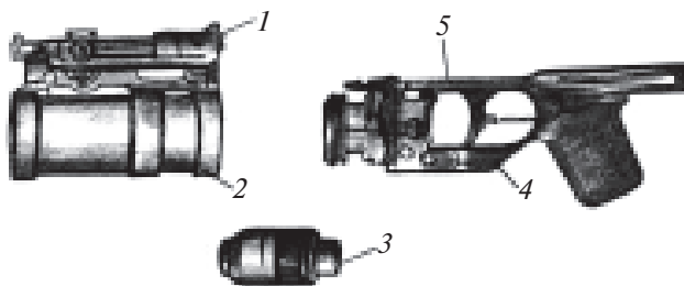
109-rasm. Stvol ostidagi granatomyotning qismlarga ajratilgan holatdagi koʻrinishi:
