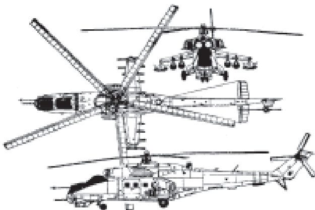
21-rasm. MI-24 B jangovar vertolyoti.
