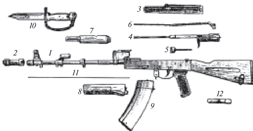
79-rasm. Avtomatning asosiy qism va mexanizmlari:
