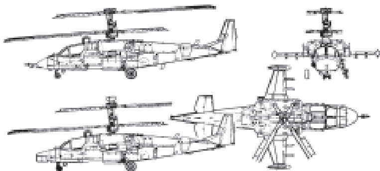
22-rasm. Ka-52 «ALLIGATOR» jangovar vertolyoti.
