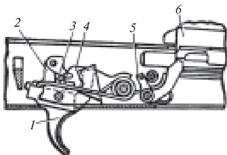
107-rasm. Zarbdor-tepki mexanizmi qismlarining o't ochilgandan so'nggi, o'tkazgich yakka tarzda o't ochish holatida:
