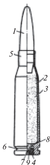
103-rasm. Jangovar patron:
