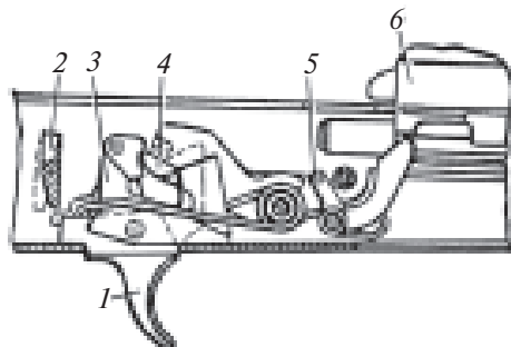
106-rasm. Zarbdor-tepki mexanizmi qismlarining o't ochishgacha bo'lgan holati:
