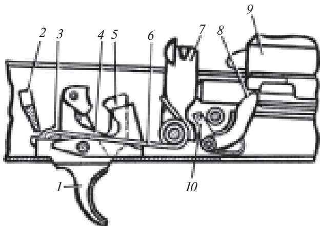
105-rasm. Zarbdor-tepki mexanizm qismlarini o'qlashgacha qo'riqlagichdan tushirilib, tepkning qo'yib yuborilgan holati:
