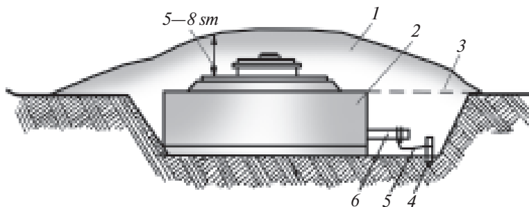
66-rasm. Tankka qarshi minaning yaydoq yerlarda o'rnatilishi:
