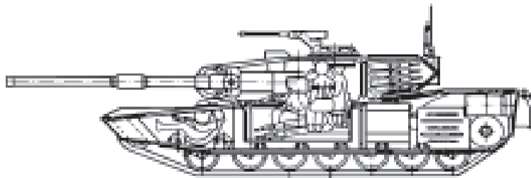
16-rasm. M1 «Abrams» tankining klassik joylashuv chizmasi.
