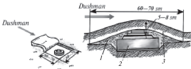
65-rasm. Tankka qarshi minalarni chim bilan qoplangan joylarga o'rnatish:
