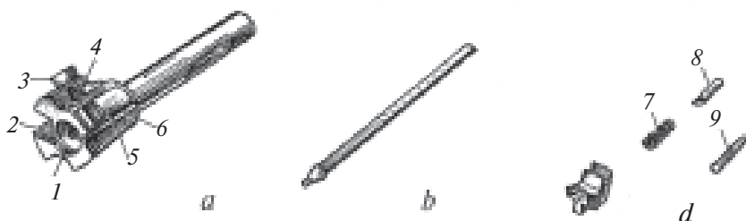
87-rasm. Zatvor:
