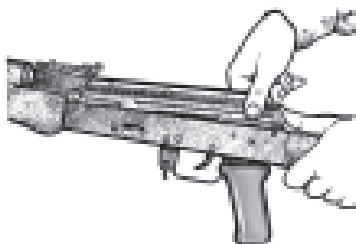
98-rasm. Stvol qutisining qopqog'ini ajratish.
