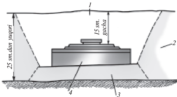
70-rasm. Qish (qor yoqqan) sharoitda tankka qarshi minaning oʻrnatilishi:
