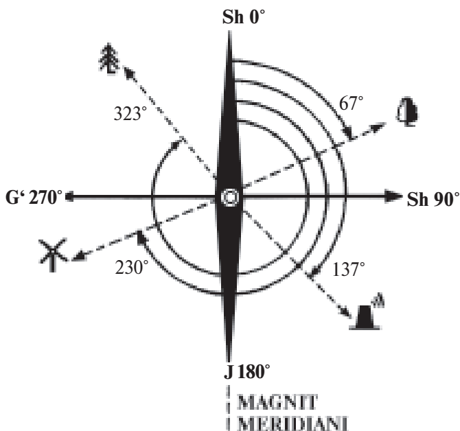
76-rasm. Magnit azimutlari:
