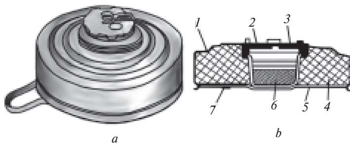
67-rasm. Tankka qarshi TM-62 M mina:
