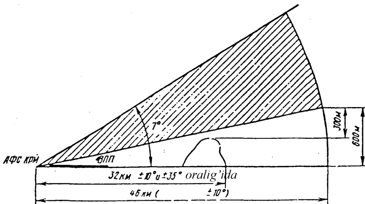
3.11-rasm. Gorizontal tekislikdagi KRM kuch hududi.
