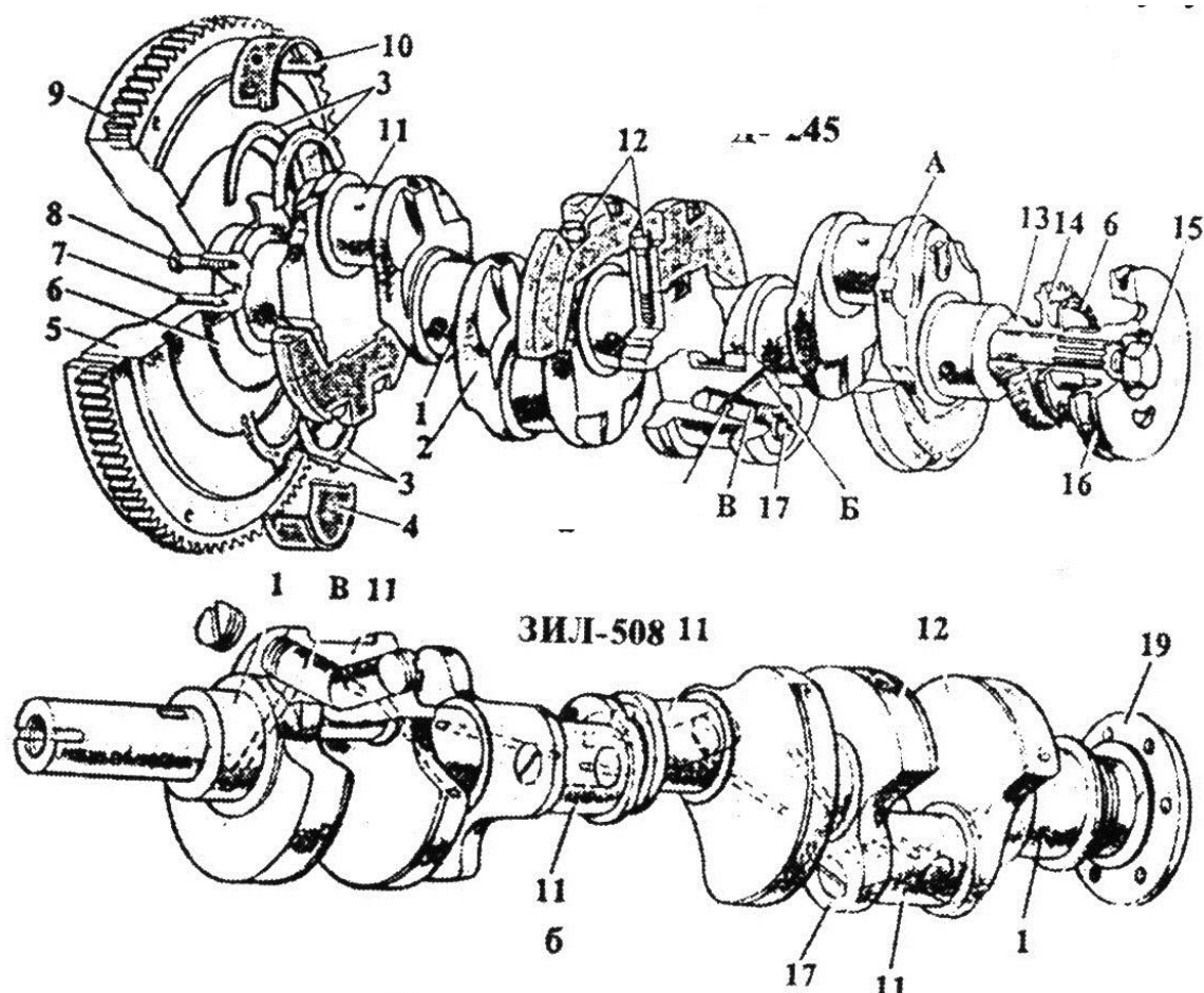
5.10-rasm. Tirsakli vallar: a - bir qatorli dizelniki, b - U-simon dizelniki,
