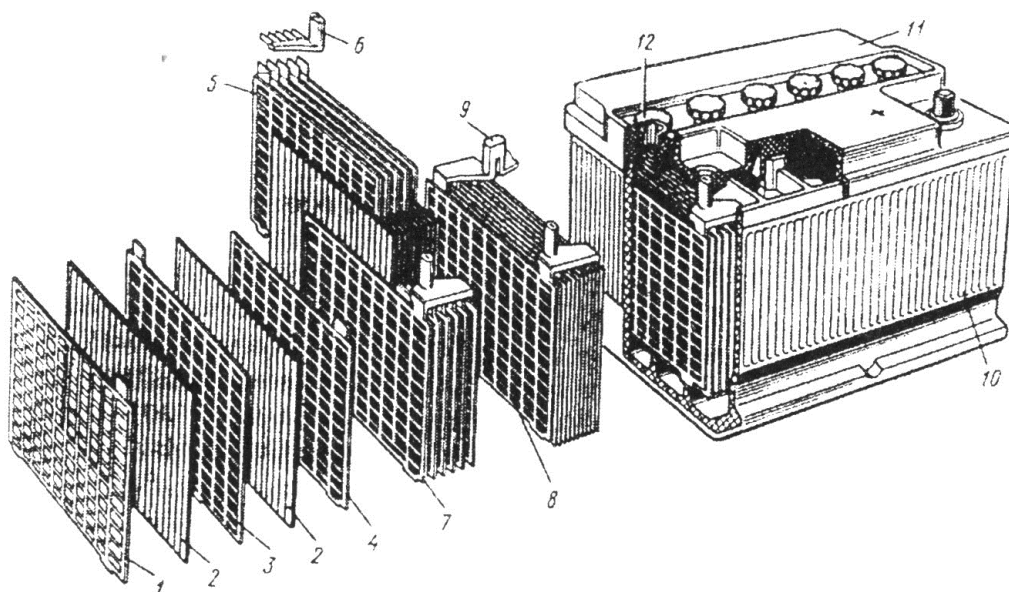
121-rasm. Umumiy qopqogi bolgan qo'rg'oshin-kislotali starterbor akkumulator batareyasining tuzilishi.
