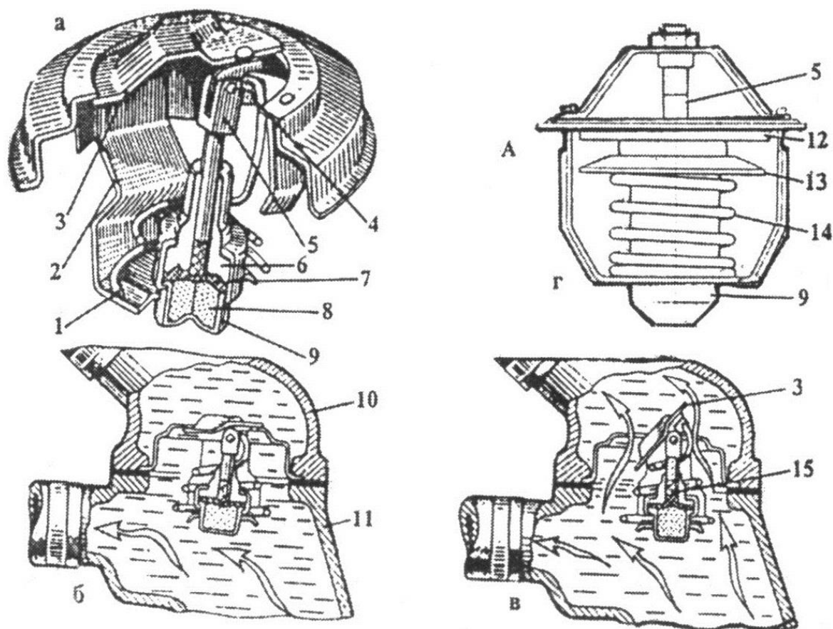
4.4-rasm. Buriladigan va oddiy klapanli termostat:
