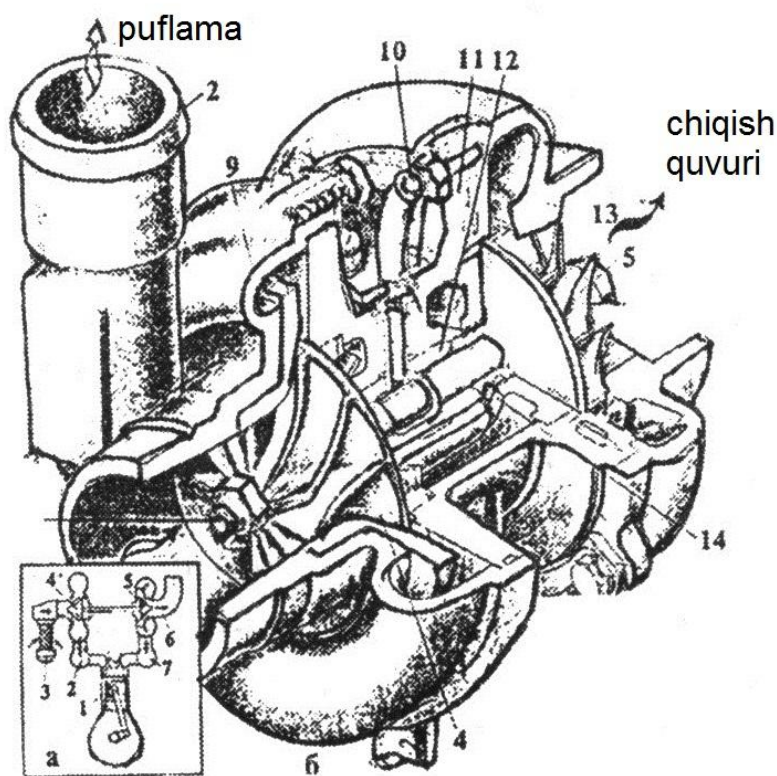
4.19-rasm. D-245 dizelining turbokompressor: a - ishlash shakli, b - tuzilishi.
