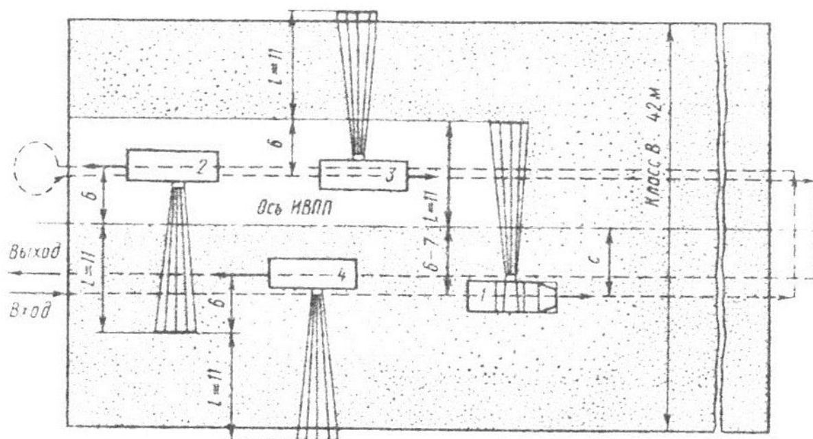
3.6-rasm. . «V» klass aerodromning SUQMini bitta shamol mashina yordamida tozalashda harakat sxemasi (yon Jama shamol 3 m/s, qor qalinligi 4 sm, qamrov kengligi 11 m):
