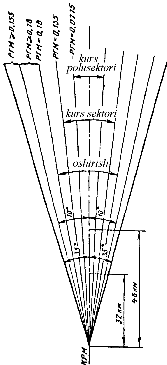
3.10-rasm. Gorizont tekislikdagi KRM kuch hududi.
