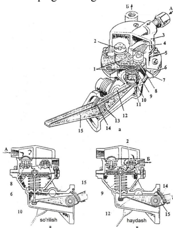
4.17-rasm. Benzin nasosi: a - tuzilishi; b va v - nasosni so'rilish va haydash vaqtidagi ishchi chizmasi.
