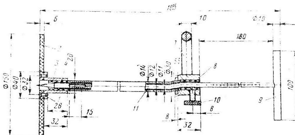
3.1-rasm. Qor, shilta va suv uchun chiqurlik o'lchagich, GM-1
