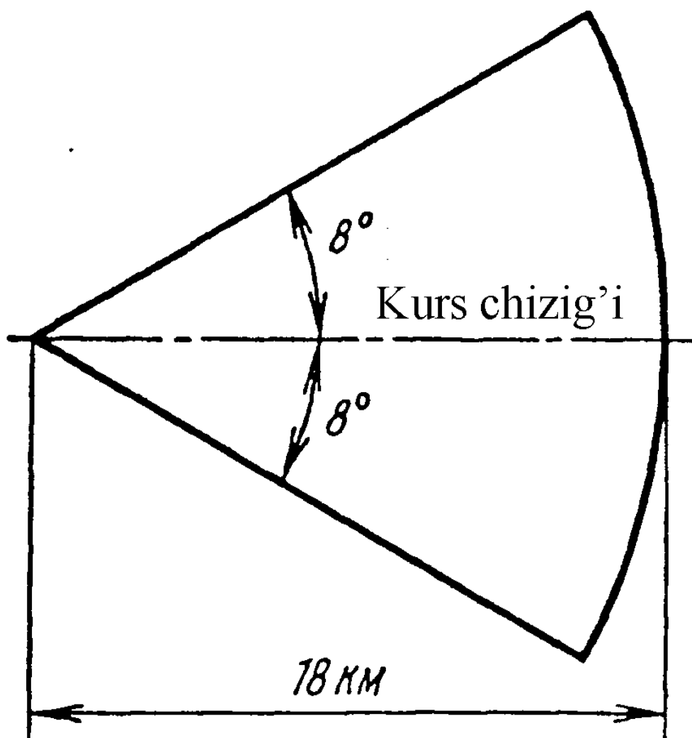
3.12-rasm. Gorizontal tekislikdagi GRM kuch hududi.
