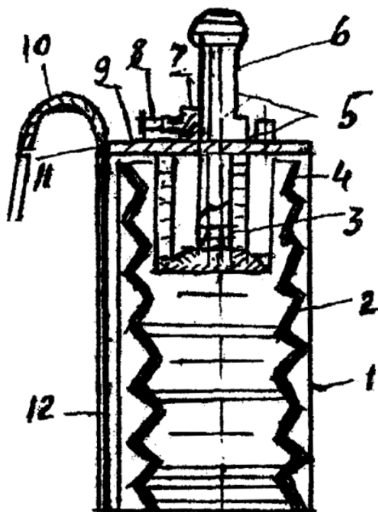
2 - rasm. Havo yutuvchi va gaz o'lchagich moslama VT-2.
