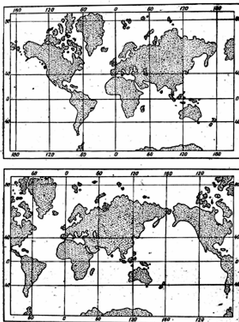
38-rasm. Dunyo kartasini 2 xil komponovkada ko‘rinishi.
