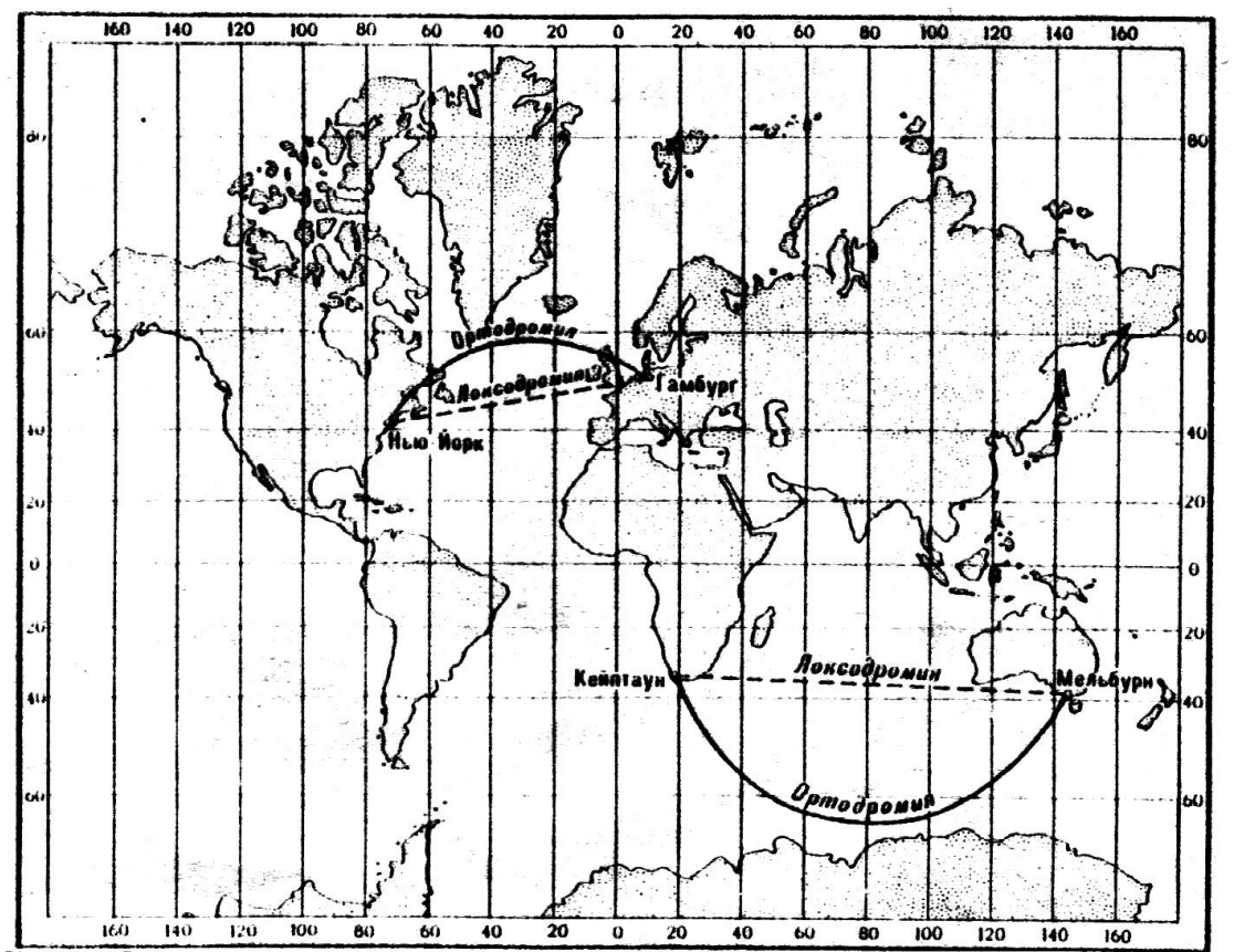
27-rasm. Merkator proektsiyasida kartografik to'ring ko'rinishi. Shimoliy va Janubiy yarim sharlarda loksodromiya va ortodromiyalarning tasvirlanishi.
