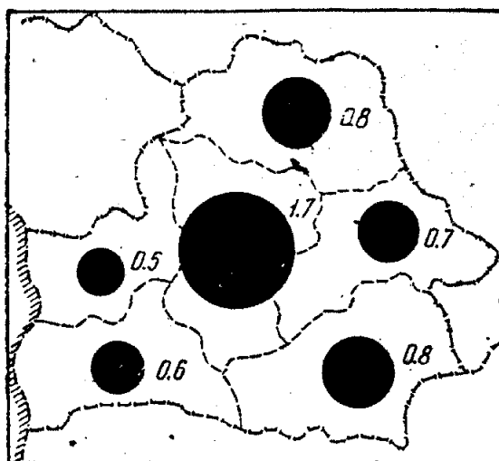
51-rasm. Doiraviy kartodiagramma (raqamlar bilan Belarus viloyatlaridagi shahar aholisining soni mln. kishi hisobida koʻrsatilgan).
