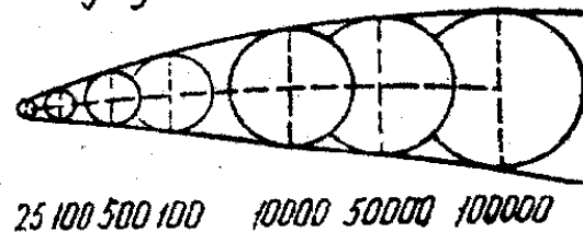
Шартли узлуksиз шкала
