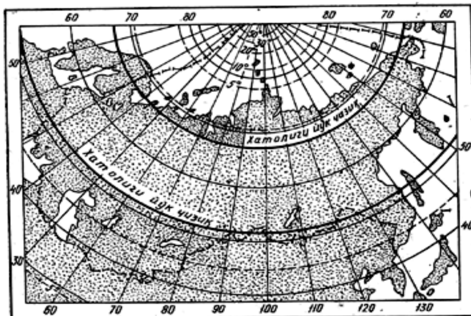
Бұрчак (ω) изоколлари
