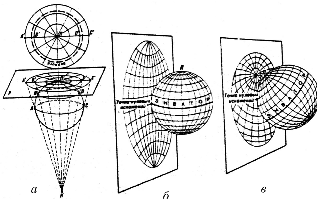
21- рasm. Азимутал проeксийанинг турлари. a -то'g'ри, b -ко'ndalang, v -qiyshiq.
