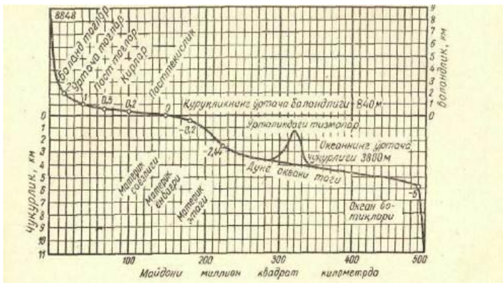
Куруқликнинг гипсографик ва океан тағининг батиграфик эгри чизиғи
