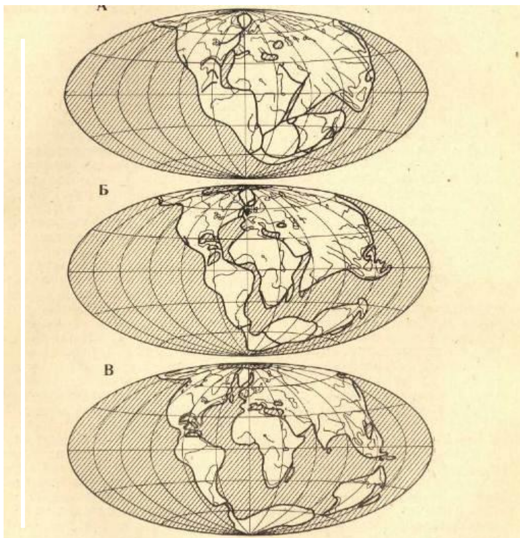
А. Вегенер гипотезасига кўра материкларнинг вужудга келиши: Л — палеозой, Б — мезозей, В — кайнозой
