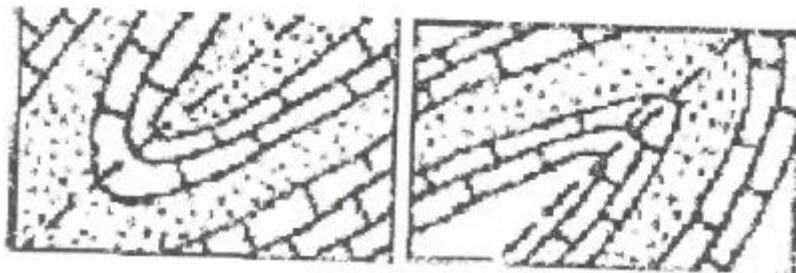
Қийшиқ бурма.
