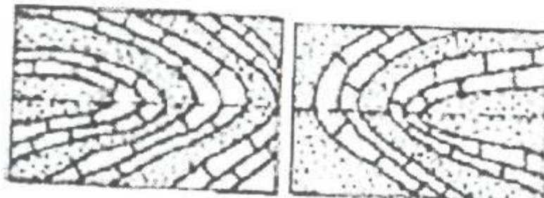
Ётиқ бурма
