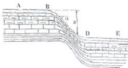
Флексура элементлари.
