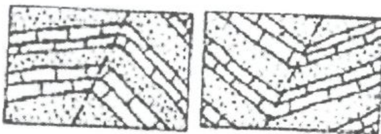
Ағдарма бурма.
