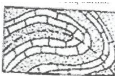
Тўнқарилган бурма.
