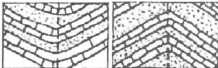
Тўғри бурма.
