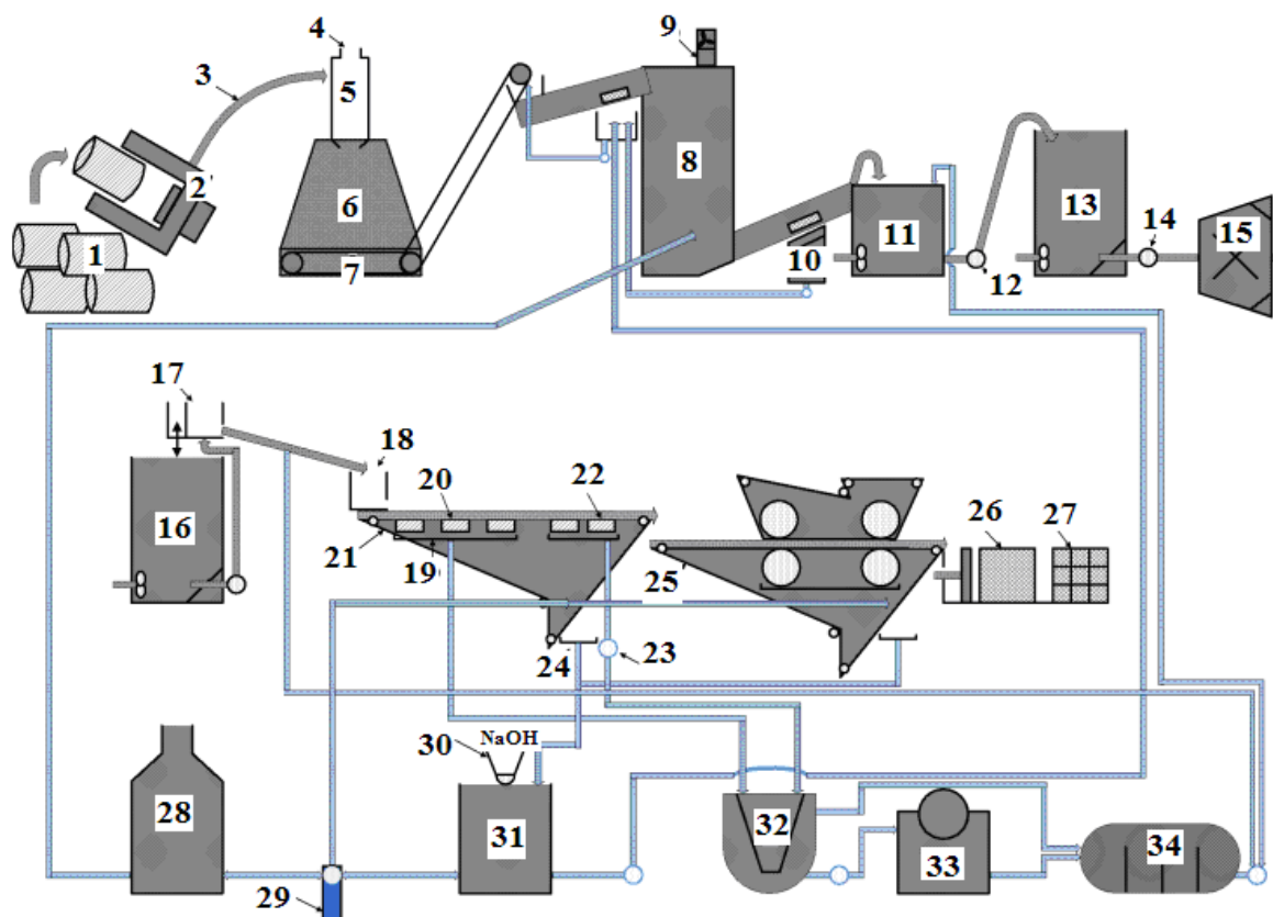
7.10-rasm. Uzlusiz usulda somondan yarim tayyor selluloza olish texnologik sxemasi:
