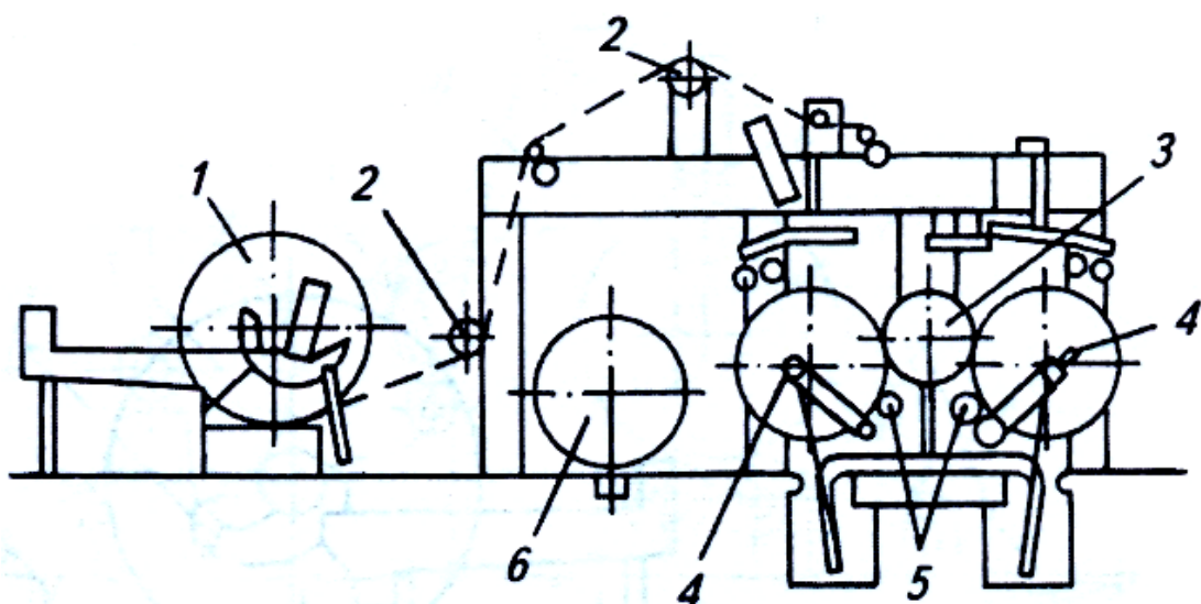
8.6-rasm. Ikkilangan uzinasiga qirqish dastgoh sxemasi: 1 – o‘raladigan rulon; 2 – qog‘oz uzatuvchi valiklar; 3 – o‘tkazuvchi silindr; 4 – o‘tkazuvchi vallar; 5 – qirqish qurilmasi; 6 – tayyor rulon.
