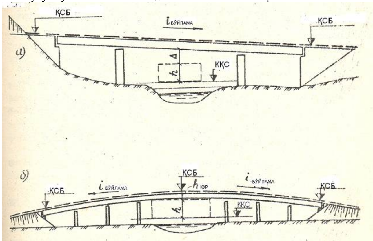
Расм 3.8. Кўприк ҳаракат қисмининг бўйлама профили:
