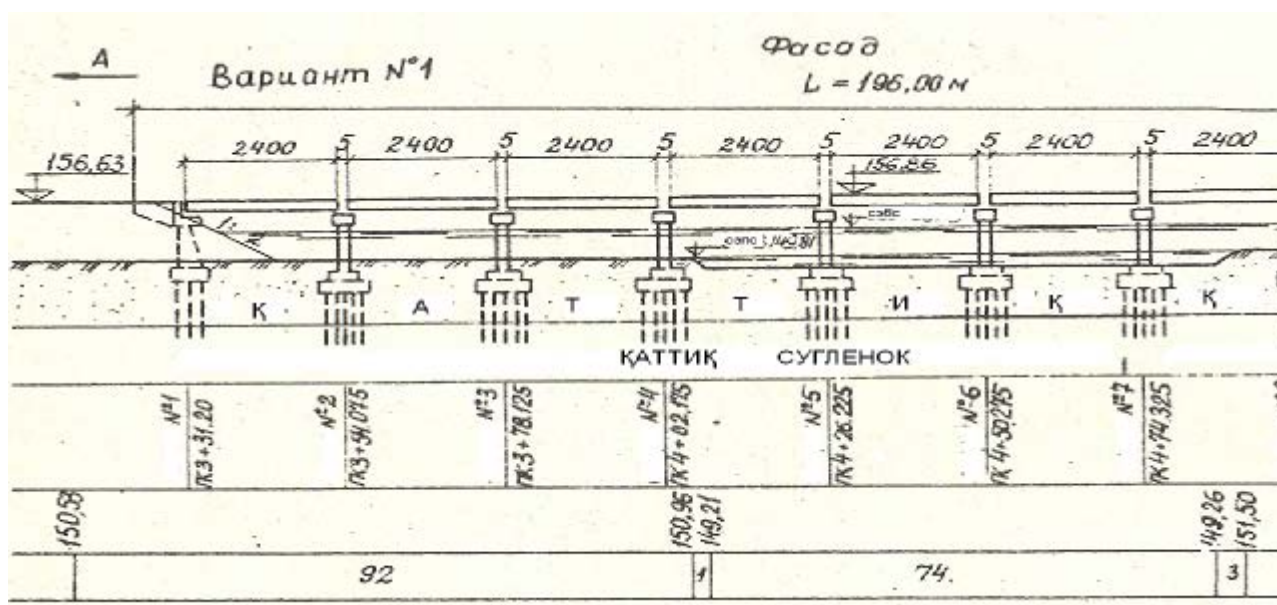
Расм.7.1.Биринчи вариант бўйича кўприк схемаси.
