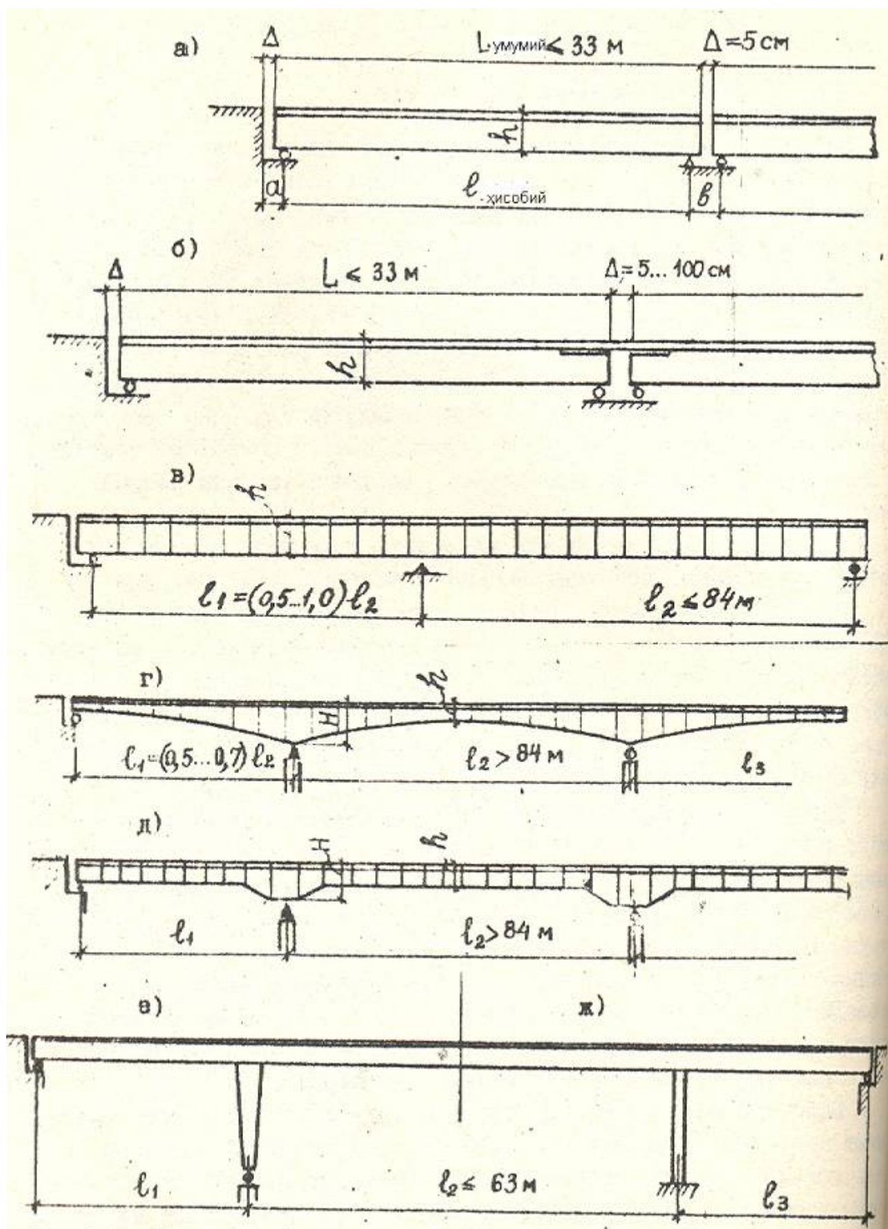
Расм 4.1. Йиғма темир бетон кўприклар системалари: а- узлукли-тўсинли ;
