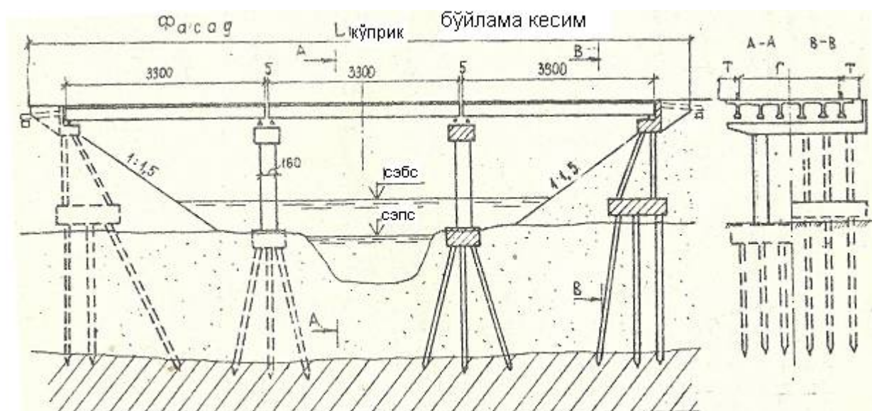
см 4 13.Тўсинли темирбетон кўприк схемаси.
