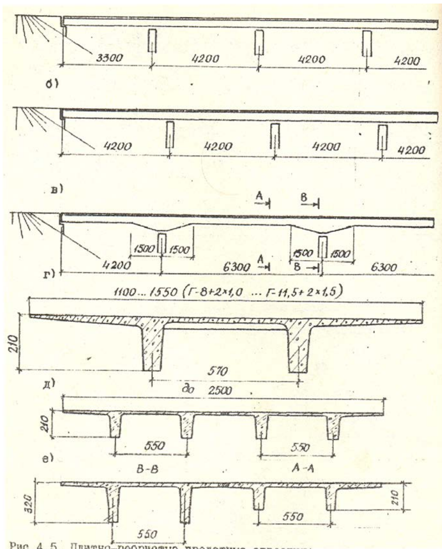
Рис. 4.5. Плита қовурғали оралиқ қурилмалар
