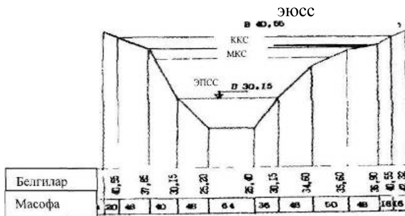
Расм 3.1. Кўприк ўтиш ўқи бўйича бўйлама кесими (М1: 100... 1: 500): ЭЮСС сувнинг энг юқори сатҳи, ЭПСС энг паст сув сатҳи, ККС кема қатнови сатҳи, МКС муз қатлами сатҳи.
