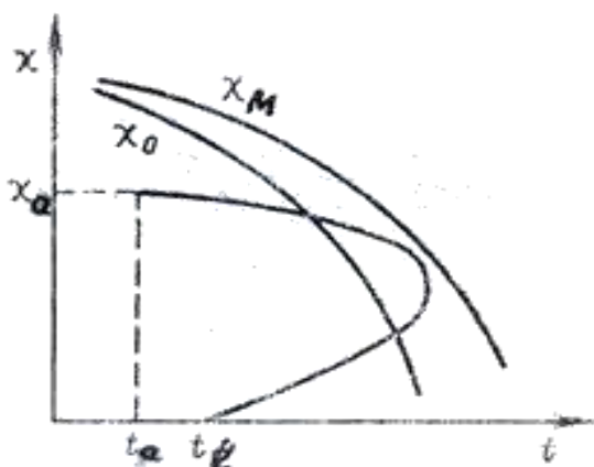
33-rasm. Ekzotermik reaksiyalar uchun quvirsimon kontakt apparatlarida mahsulotga aylanish darajasining o'zgarishi.
