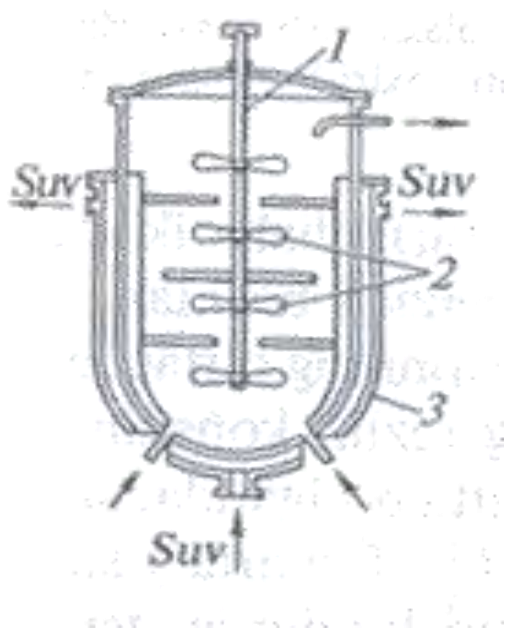
11-rasm. Izotermik rejimli to'liq aralashtirgichi aralashtiruvchi reaktor-aralashtirgichli qaynovchi qavatli katalitik apparat. ko'ylagi(g'ilofi)
