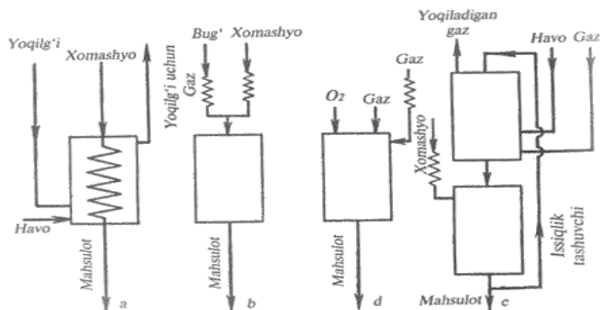
92-rasm. Issiqlik berishning asosiy usullari.
