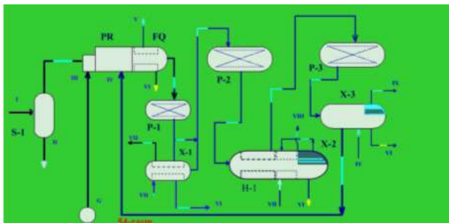
54-rasm. Muborak gazni qayta ishlash zavodi oltingugurt ishlab chiqarish qurilmasining sxemasi. C- 1-kiritish separatori; PR-pech-reaktor; fq-foydalanish qozoni; p-1,p-2,p-3-reaktorlar; K-1, K-2, K-3-kondensatorlar; I-issiqlik almashtirgich; Q-qizdirgich, f-filtr; G-gazpurkagich; I-nordon gaz, II-suyuqlik tomchilari;III-havo,IV-yuqori bosimli havo,V-yuqori bosimli suv bug'lari, VI- gaz oltingugurti, VII- past bosimli suv, VIII-past bosimli suv bug'I,IX-chiqib ketuvchi gazlar.
