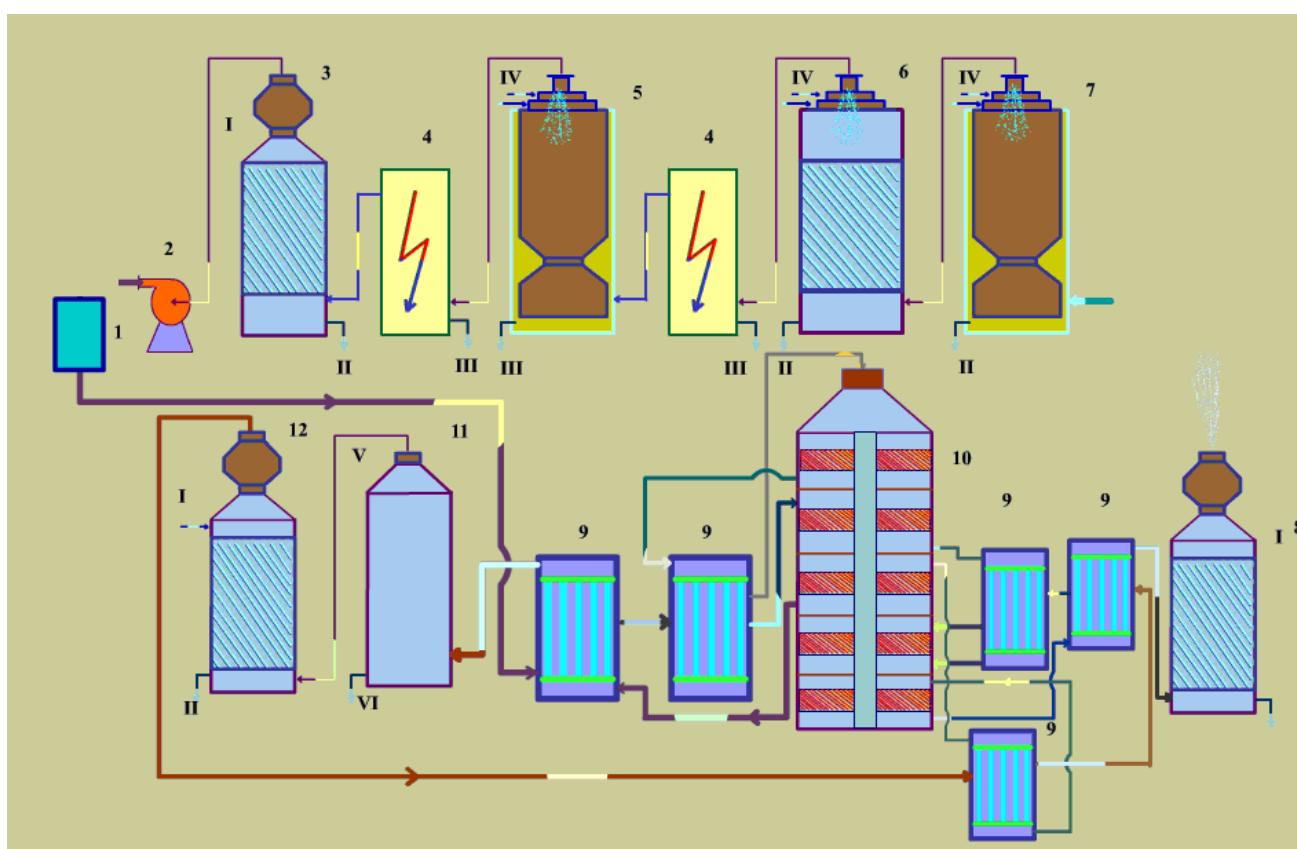
63-rasm. Kolchedanni kuydirib olingan gazdan ( SO_2 ) sulfat kislota ishlab chiqarishnin IK/IA sxemasi.
