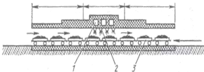
81-rasm. Tunnel pechi(ko'ndalang kesimi) 1-havo kiradigan kanallar; 2-gorelkalar; 3-kuydiriladigan material ortilgan vagonchalar.
