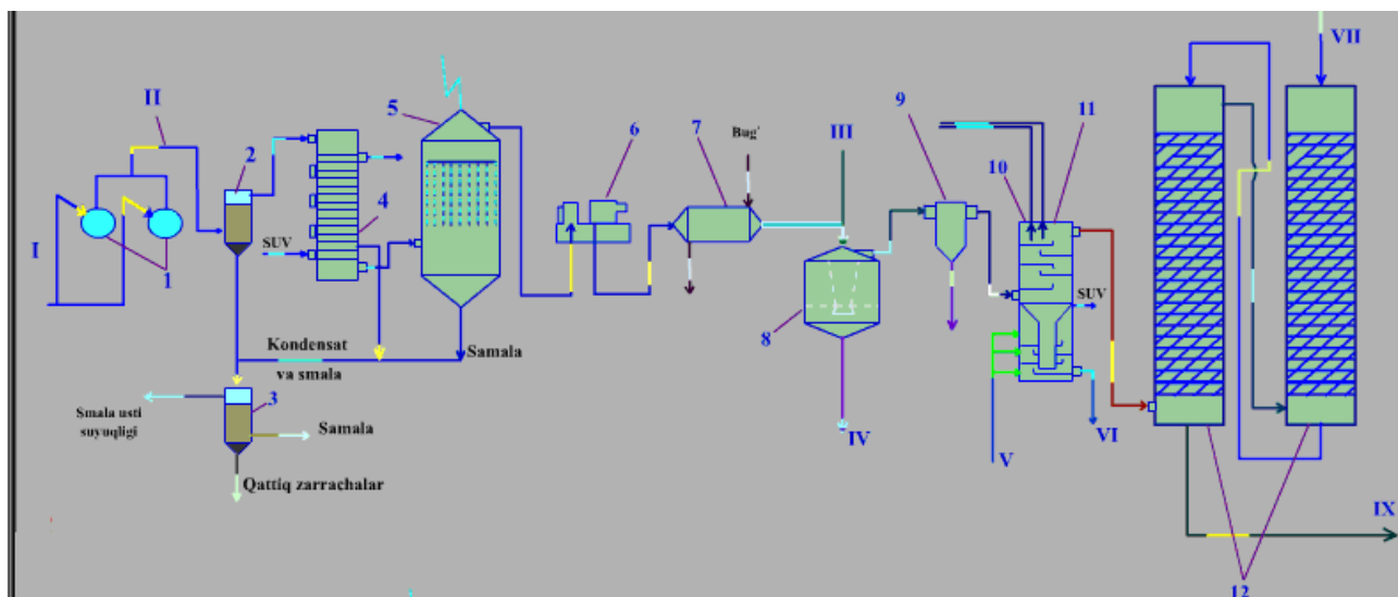
90-rasm. To'g'ri koks gazlarini qayta ishlash sxemasi.
