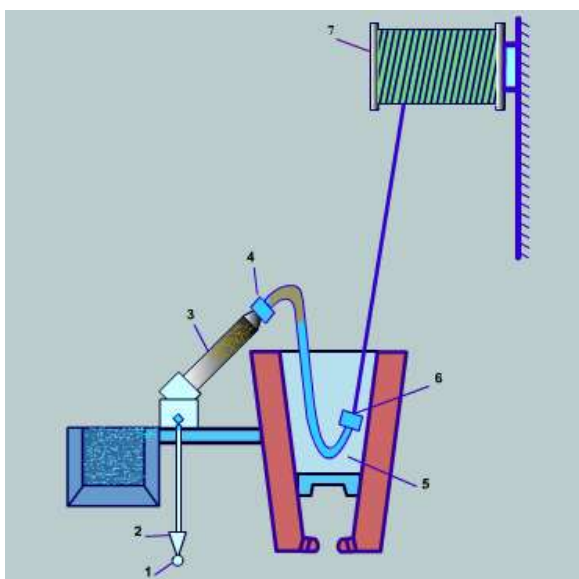
131-rasm. Eritmadan “Ho’l” yigirish orqali tolagashakl berish sxemasi.
