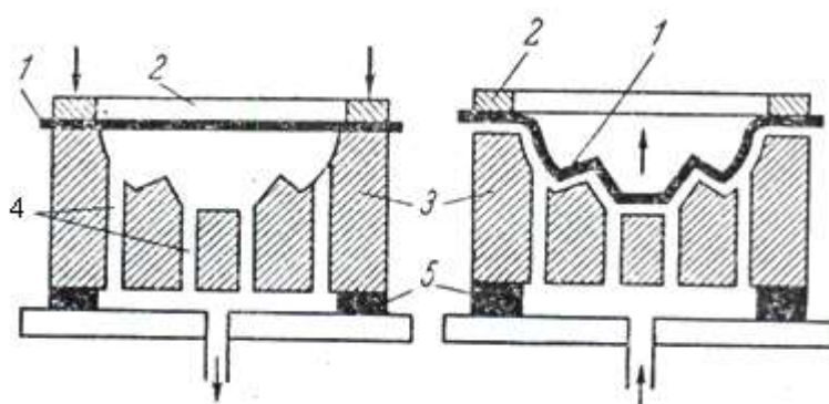
136-rasm. Plastmassadan vakuumda buyum tayyorlash apparati. 1- plastmassa varaqlari; 2-qisuvchi halqa; 3- shakl' 4- so'rib chiqarish va siqilgan havoni kiritish tuynugi; 5-qistirma.
