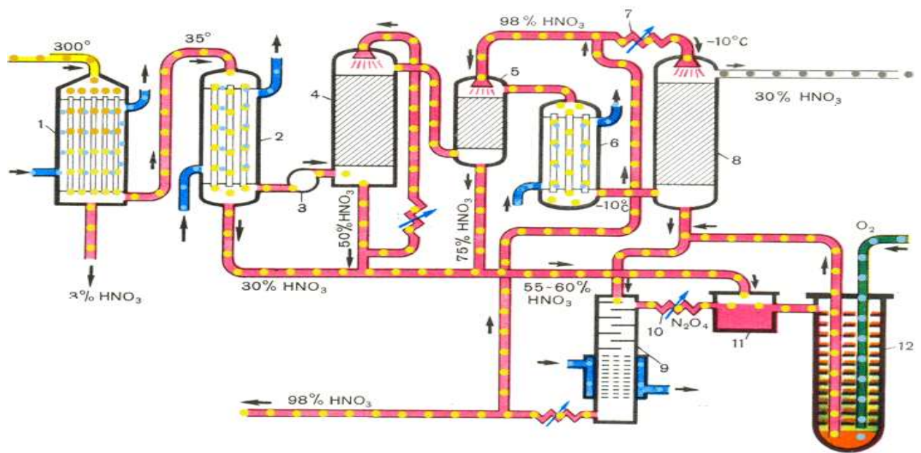
71-rasm. Konsentratlangan nitrat kislota sintezining soddalashtirilgan sxemasi. 1-tez sovutgich; 2-suvkli sovutgich; 3-ventilyator; 4-oksidlovchi minora; 5-to'liq oksidlash; 6,7,10-shurabali sovutgichlar; 8-yuttiruvchi minora; 9-tokchali oqartiruvchi colonna va uning bug' uchun kuylagi; 11-aralashtirgich; 12-elaksimon tarelkali avtoklav.
