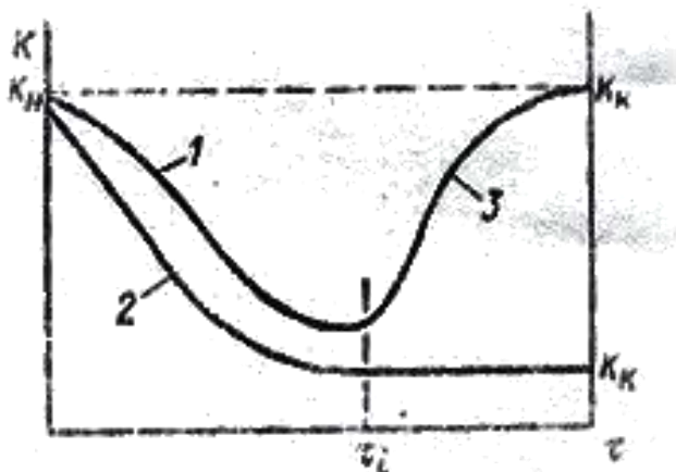
26-rasm. Katalizatorning qaytar (1) va qaytmas(2) zaxarlanganida katalitik reaksiyaning boshlanishidan K_b to oxirigacha K_a tezlik konstantasining o'zgarishi.(3)-chi egri chiziq reaksiya aralashmadan zaxar yo'qotilgach, aktivlikning qayta tiklanishi.
