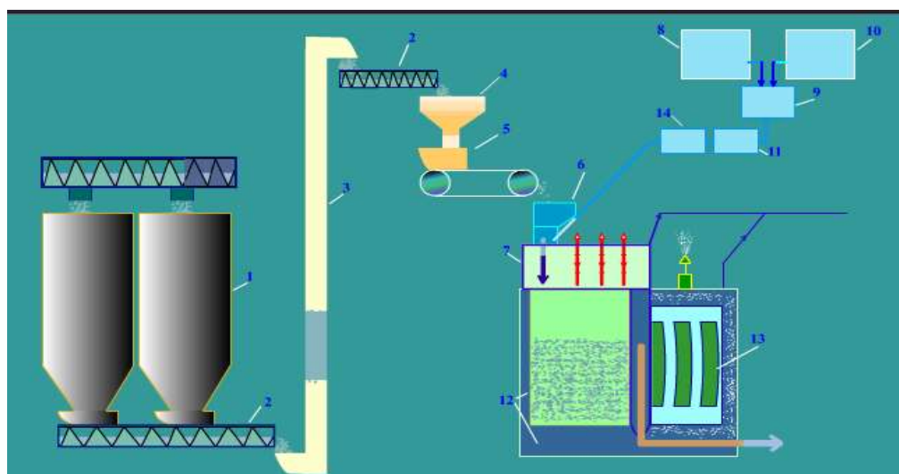
76-rasm. Uzlüksiz usulda superfosfat ishlab chiqarish sxemasi.
