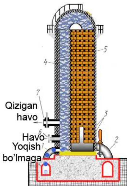
49-rasm. Kauper(havo qizdirgich). 1,6,7-gaz kirib-chiqish tuynuklari; 2-tutun chiqish joyi; 3-sovuq havo kirish tuynugi; 4- yoqish bo'limi; 5-nasadkali bo'limi.
