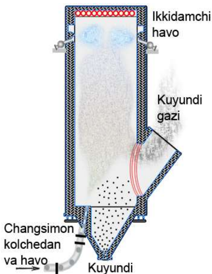
58-rasm. Kolchedanni changitib kuydirish pechi. 1-silindrsimon g'ilof; 2-futrovka(qoplamasi); 3-kuyundi uchun bunker; 4-kolchedanva havo aralashmasini kirituvchi forsunka; 5-sovutuvchi ekran.
