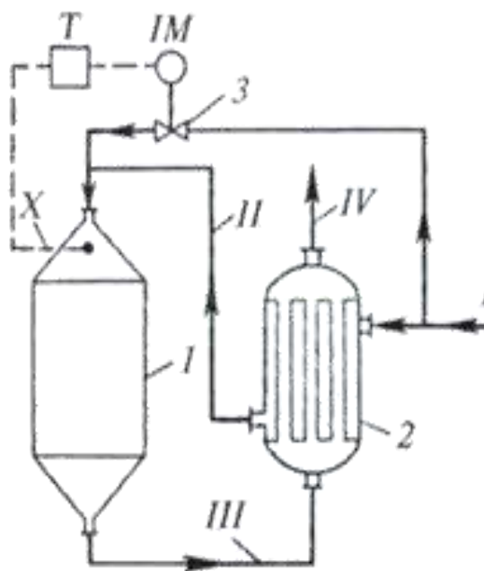
1-rasm Reaktorlarning harorat rejimini oddiy avtomatlashtirish sxemasi
