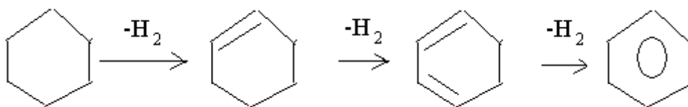
Siklogeksan siklogeksen siklogeksadien benzol
