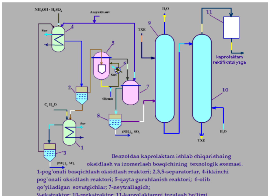
102-rasm. Benzoldan kaprolaktam ishlab chiqarishning oksidlash va izomerlash bosqichining texnologik sxemasi.
