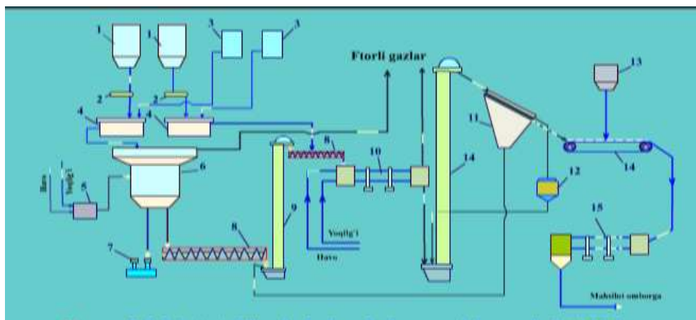
80-rasm. Uzluksiz(patokli) oqimda donadorlangan qo'sh superfosfat ishlab chiqarish sxemasi.
