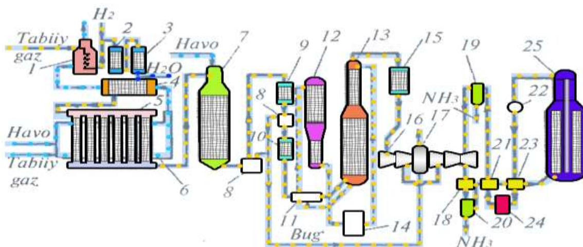
66-rasm. Metan konversiyasi bilan birga ammiak sintezini qo'shib amalga oshiruvchi qurilmaning sxemasi. 1-tabiiy gaz qizdirgichi; 2-organik oltingugurtni gidrogenlash reaktori; 3-vodorod sulfid adsorberi; 4-issiqlik almashtirgich; 5-quvursimon pech metan konvertori; 6-yoqish pechi; 7-
