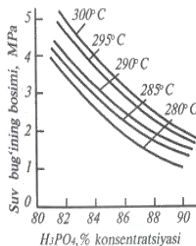
107-rasm. Turli haroratda suv bosimining fosfat kislota konsentratsiyasiga bog'liqligi
