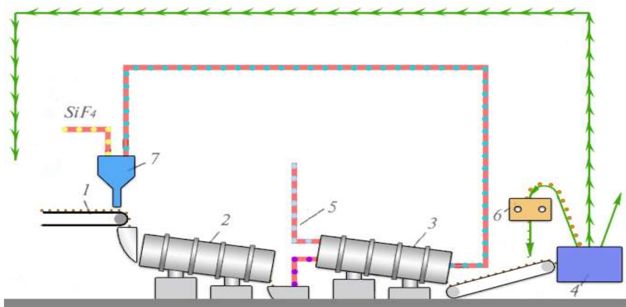
78-rasm. Superfosfatni donadorlash qurilmasi sxemasi.
