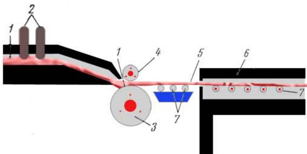
86-rasm. Uzluksiz prokatlash orqali sayqallangan shisha listini tayyorlash sxemasi. 1-shisha massa; 2-to'siq(qopqoq)' 3,4-valklar; 5-shisha lenta; 6-yumshatish pechi; 7-shisha lentani harakatlantirish uchun g'ildiraklar.
