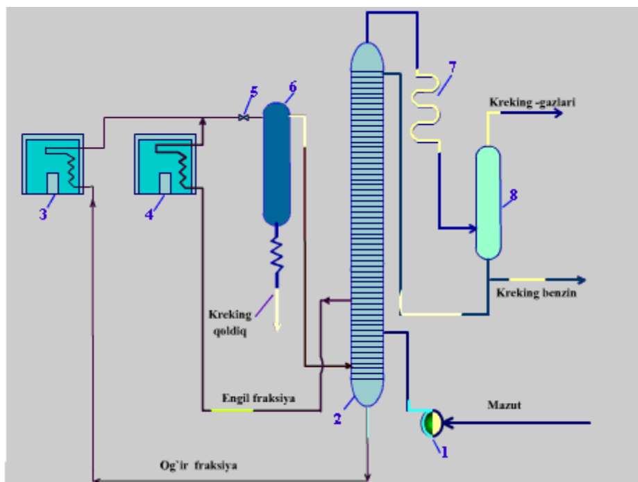
97-rasm. Mazutni termik krekingi.
