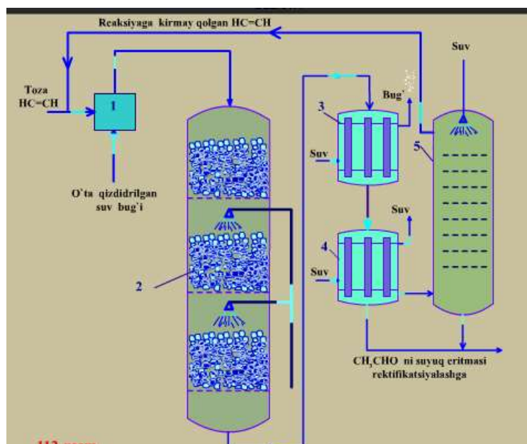
110-rasm.. Atselinni bug' fazali gidratlash yo'li bilan sirka aldegid olish sxemasi.
