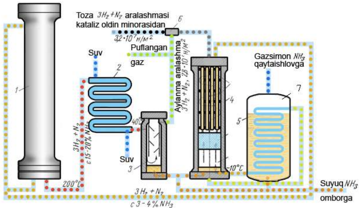
64-rasm. O'rta bosimda ammiak ishlab chiqarish sxemasi. 1-sintez kolonnasi; 2-bug' qozoni suvini qizdirgichi; 3-suvli sovutgich' 4- kondensator; 5-sirkulyatsiyalovchi(aylantiruvchi) turbokompressor; 6- kondensatsiya kolonasi; 7-bug'lantirgich
