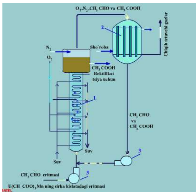
111- rasm. Sirka aldegidni oksidlab sirka kislota olish sxemasi. 1-oksidlash minorasi; 2-kondensator; 3-nasoslar.
