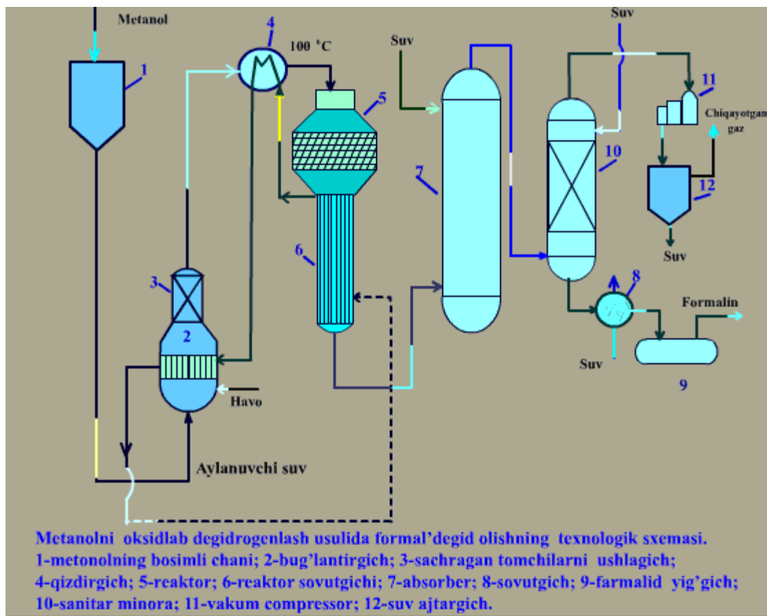
109-rasm. Metanolni oksidlab degidrogenlash usulida formaldegid olishning texnologik sxemasi.
