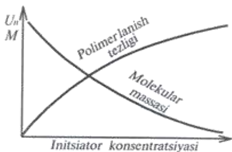
116-rasm. Polimer molekulyar massasining va polimerlanish tezligining katalizator konsentratsiyasiga bog'liqligi.
