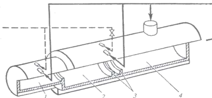
60-rasm. Oltingugurtning yoqish uchun ishlatiladigan siklon pech. 1-oltingugurt va havo berish uchun forsunkali forkamera; 2- yoqish bo'limi; 3-gazni girdobli harakatga keltiruvchi halqalar.
