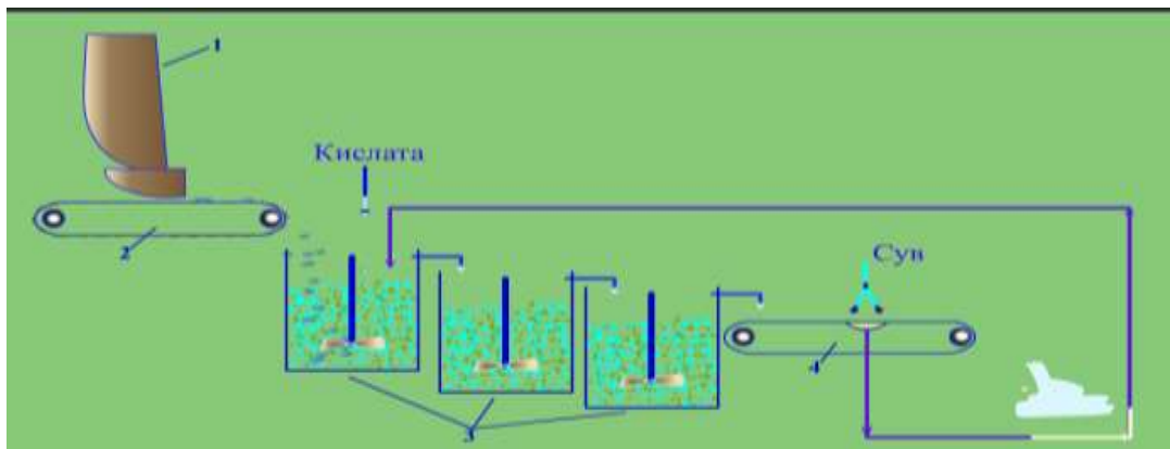
79-rasm. Ekstraksiya usuli bilan fosfat kislota ishlab chiqarish sxemasi. 1-bunker; 2-tasmali dozalogich; 3-ekstraktorlar; 4-tasmali vakuumfiltr.
