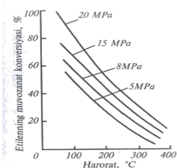
106-rasm. Etilenni etalonga aylanishdagi bug'i muvozanat konversiyasining harorat va bosimga bog'liqligi.
