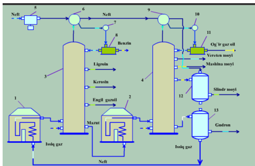
94-rasm. Atmosfera vakuumli qurilmada neftni haydash. 1,2-quvirsimon pechlar; 3,4-rektifikatsiya kanallari; 5-nasoos; 6,9,12,13- issiqlik almashtirgichlar; 7,10-kondensatorlar; 8-benzin qabul qilish qurilmasi; 11-gazoyl qabul qilish qurilmasi.
