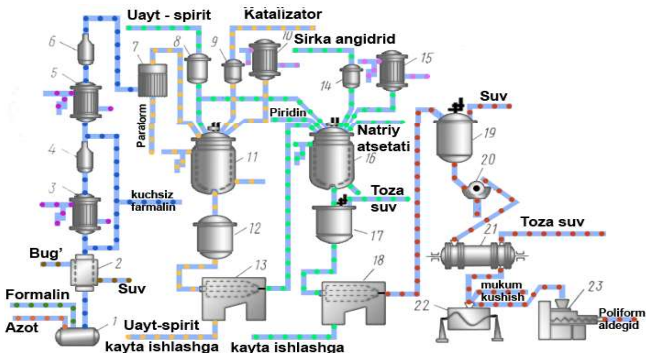
120-rasm. Poliformaldegid ishlab chiqarish qurilmasining sxemasi.
