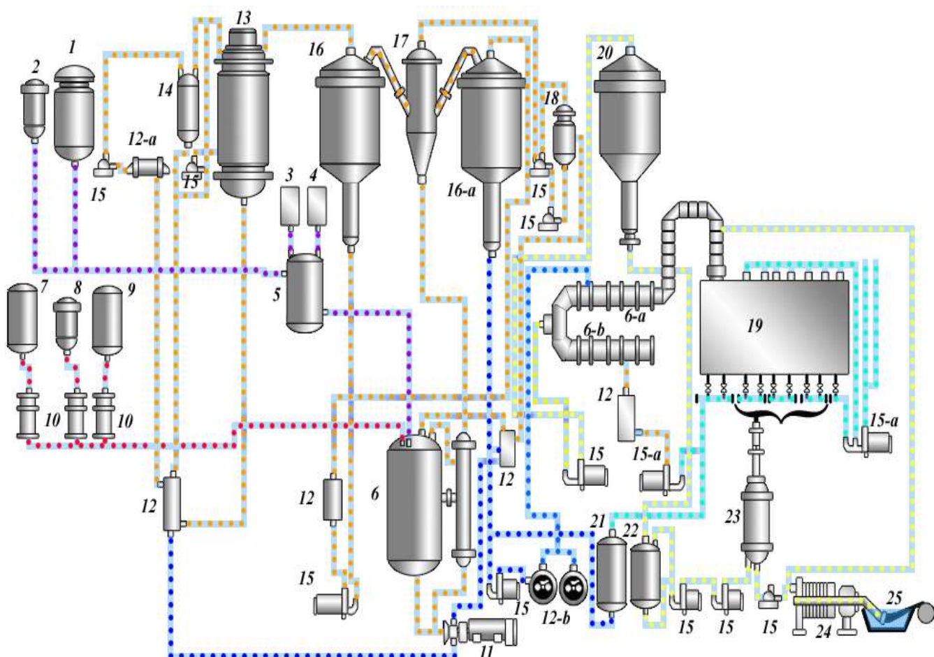
133-rasm. Nitron ishlab chiqarish sxemasi.
