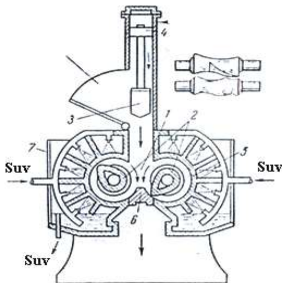
138-rasm. Yopiq rezina aralashtirgich. 1-aralashtirgichning bo'lmasi(kamerasi); 2-rotor(apparat ichida aylanuvchi qism); 3-yuqori zatvor(ochib yopuvchi mexanizm,tamba); 4-porshen; 5-bo'lma korpusi; 6-pastki zatvor; 7-chiqib ketuvchi suv ko'lagi(g'ilof).
