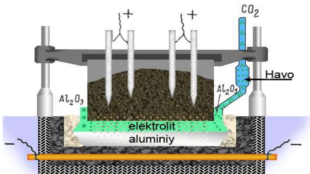
53-rasm. Anodga yuqoridan tok beruvchi uzluksiz o'zi quyuvchi anodli alyuminiy suyuqlantirish uchun elektrolizyor. 1-anod g'ilofi; 2-anod ramasi; 3-ko'targichlar; 4-gaz yig'gich; 5-uglerod (11)oksidini yoqish uchun gorelka; 6-yarim suyuq anod massasi; 7-qattiq anod massasi; 8-po'lat mixlar; 9-komir blok va plitalar; 10-o'tga chidamli g'isht; 11-elektrolizyor g'ilofi; 12-po'lat sterjin; 13-elektrolitning qotgan po'stlog'i.
