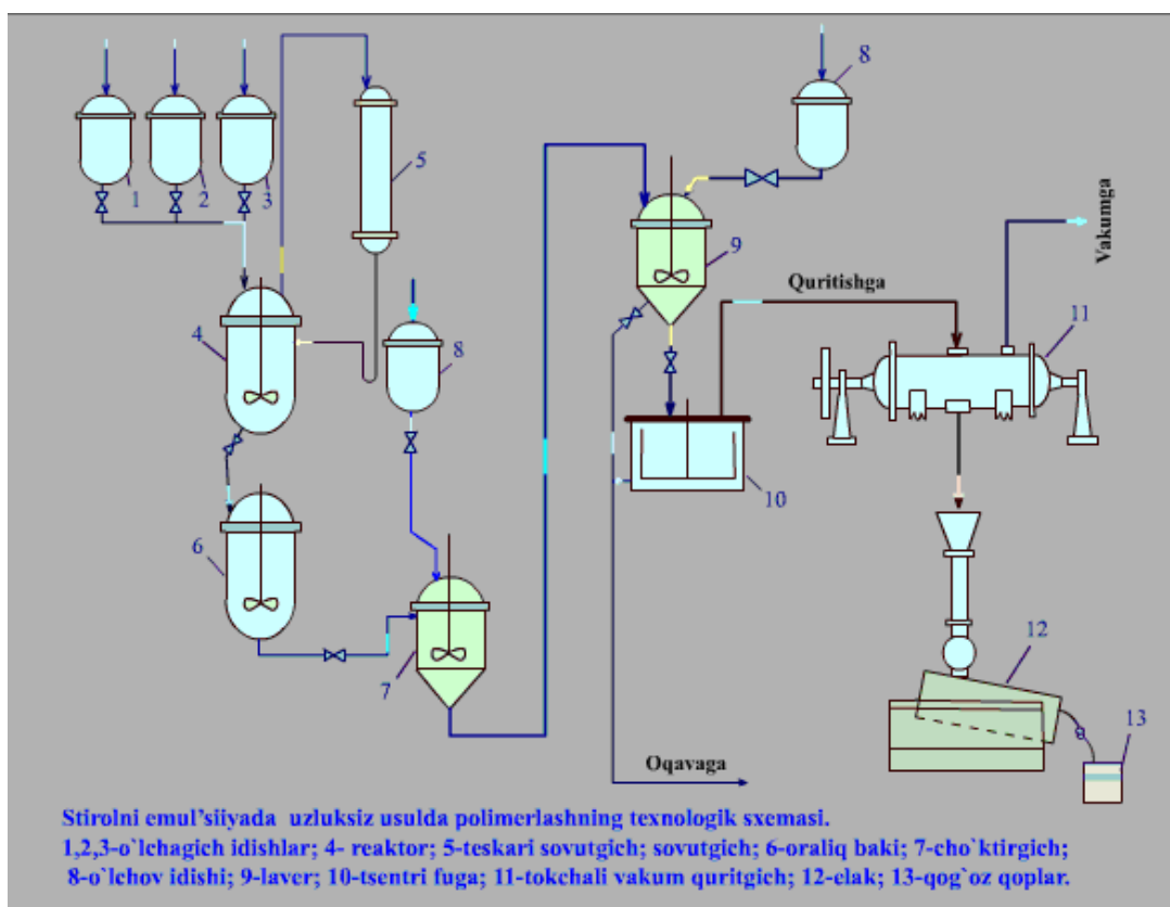
125-rasm.Stirolni emulsiyada uzluksiz usulda polimerlashning texnologik sxemasi
