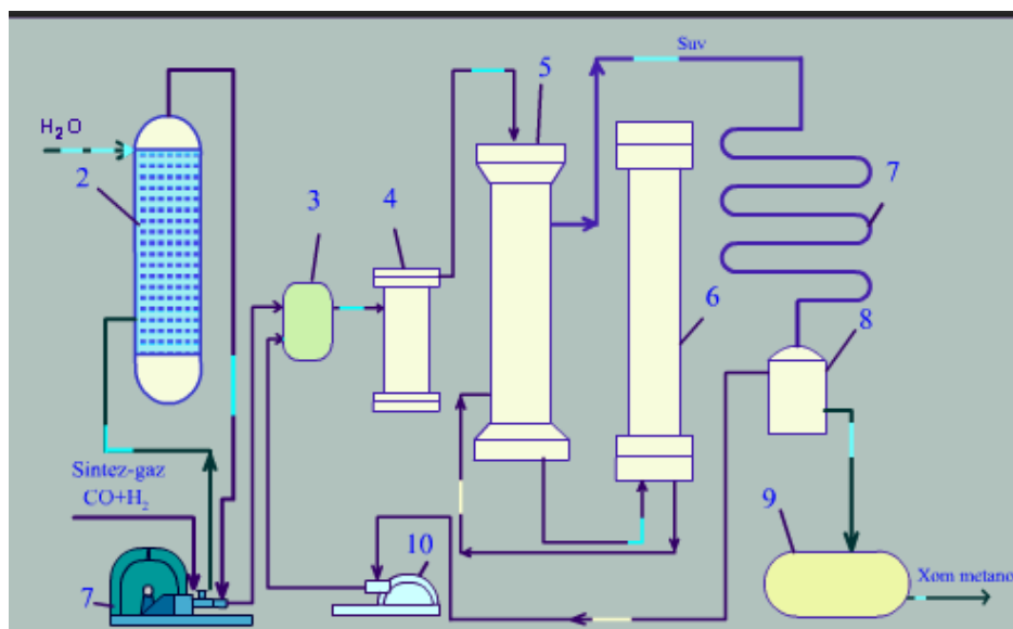
104-rasm. Uglerod(II) oksidi va vodoroddan metanol sintezi qurilmasining sxemasi. 1-kompressor; 2-skrubber; 3-aralashtirgich; 4-filtr; 5-issiqlik almashtirgich; 6-sintez kolonnasi; 7-kondensator; 8-separator; 9-xom spirt yig'gichi; 10-serkulyatsiya kompressor.
