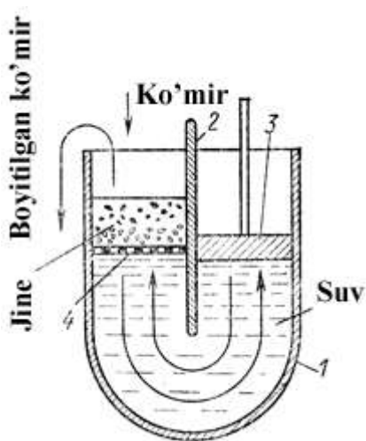
39-rasm. Ho'l usulda boyituvchi cho'ktirish mashinasining sxemasi
