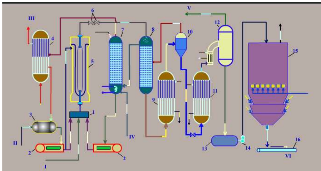
74-rasm. Karbamid ishlab chiqarishning soddalashtirilgan sxemasi. 1-aralashtirgich; 2,14-nasoslar; 3-suyuq ammiak yig'gichi; 4-kondensator; 5-sintez kolonnasi; 6-drossel jumrak; 7-yuvish kolonnasi; 8-1 pog'onali rektifikatsiya kolonnasi; 9,11-qizdirgichlar; 10-separator; 12-vakuum bulantirgich apparat; 13-karbamid suyuqlanmasini yig'gichi; 15-donadorlash minorasi; 16-transportyor.
