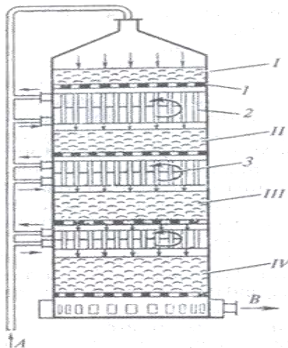
30-rasm. Qavatlar orasida issiqlik almashtirgichi bo'lgan tokchali kontakt apparati. 1-panjara; Ichki issiq almashtirgich; 3-to'siq; I,II,III,IV-katalizator qavatlar.
