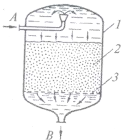
47-rasm. Kationit filtrining tuzilishi. 1-korpus; 2-kationit qavati; 3-qalpoqchali panjara; A – suv yoki regeneratsiyalanadigan eritmaning chiqishi. B – suv regeneratsiyalangan eritmaning chiqishi.
