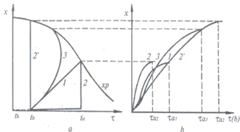
15-rasm Adiabatik va politermik siqib chiqarish reaktorlarining tartiblarini izotermik to'liq aralashtirish reaktori tartiblari bilan taqqoslash (a)/ turlireaktor tiplarida dastlabki moddaning mahsulotga aylanish darajasining vaqtga bog'liqligi (b). 1 – siqib chiqish adiabatik reaktori; 2 – izotermik aralashtirish reaktori; 3 – politermik siqib chiqarish reaktori. Reaksiya vaqtining oxiri b rasmda \tau_a , \tau_{a2} , \tau_{a3} lar bilan belgilangan.
