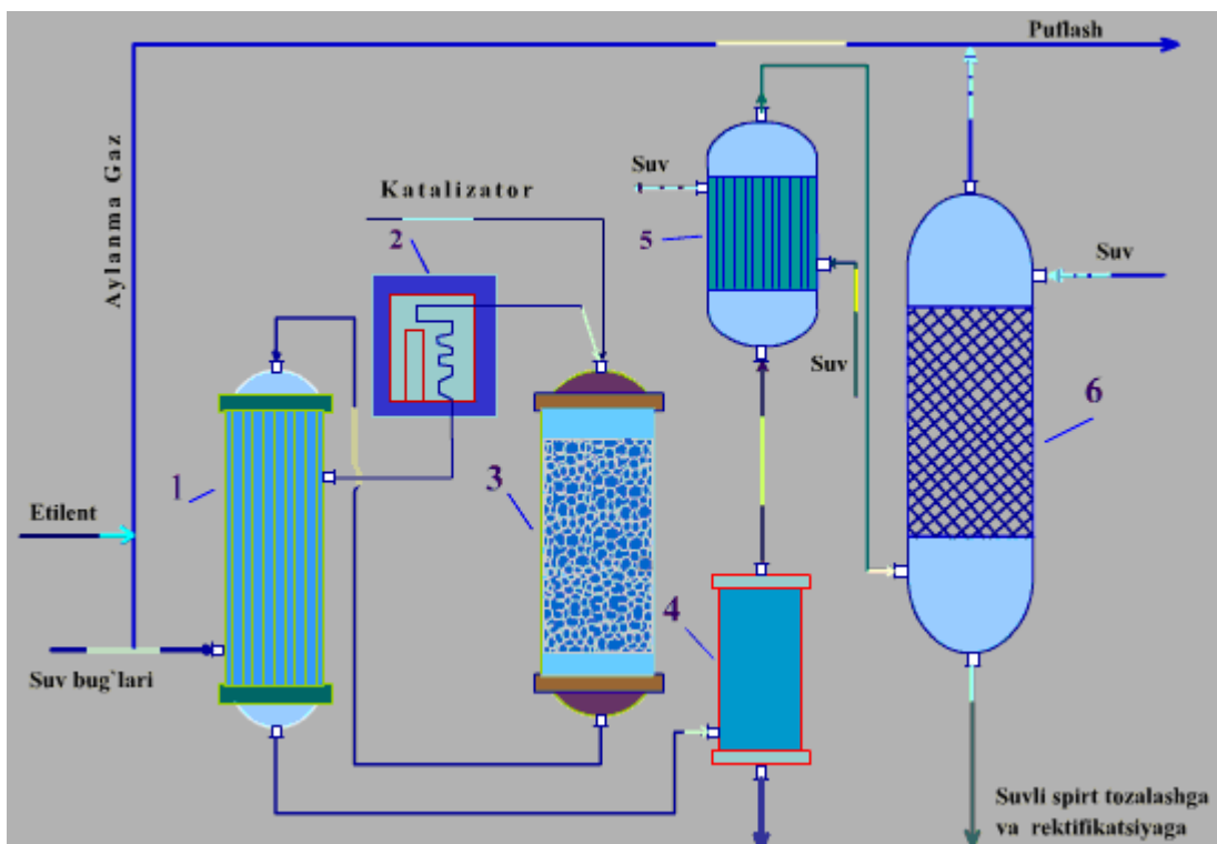
108-rasm Etalon ishlab chiqarish uchun etilenni bug'li muhitda katalitik gidratlash qurilmasining sxemasi.
