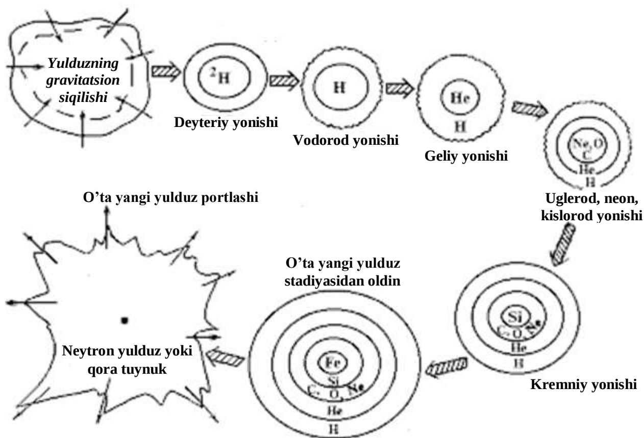
Rasm 1. Massiv yulduzining ( M > 25 M_{\odot} ) evolyutsiyasi etaplari
