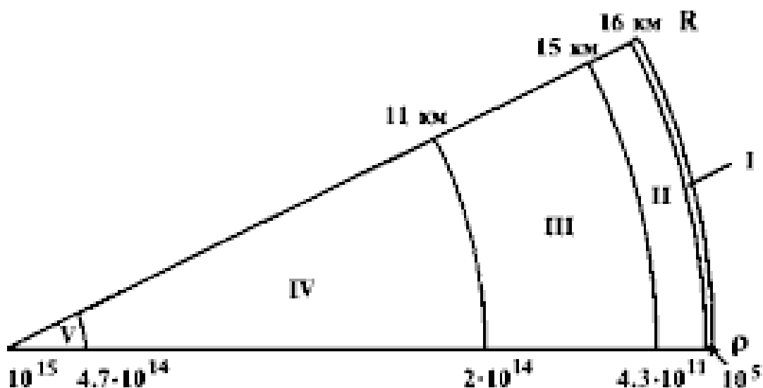
Rasm 10. Massasi 1,4 M_{\odot} bo'lgan R = 16 km radiusli neytron yulduzining kesimi.
