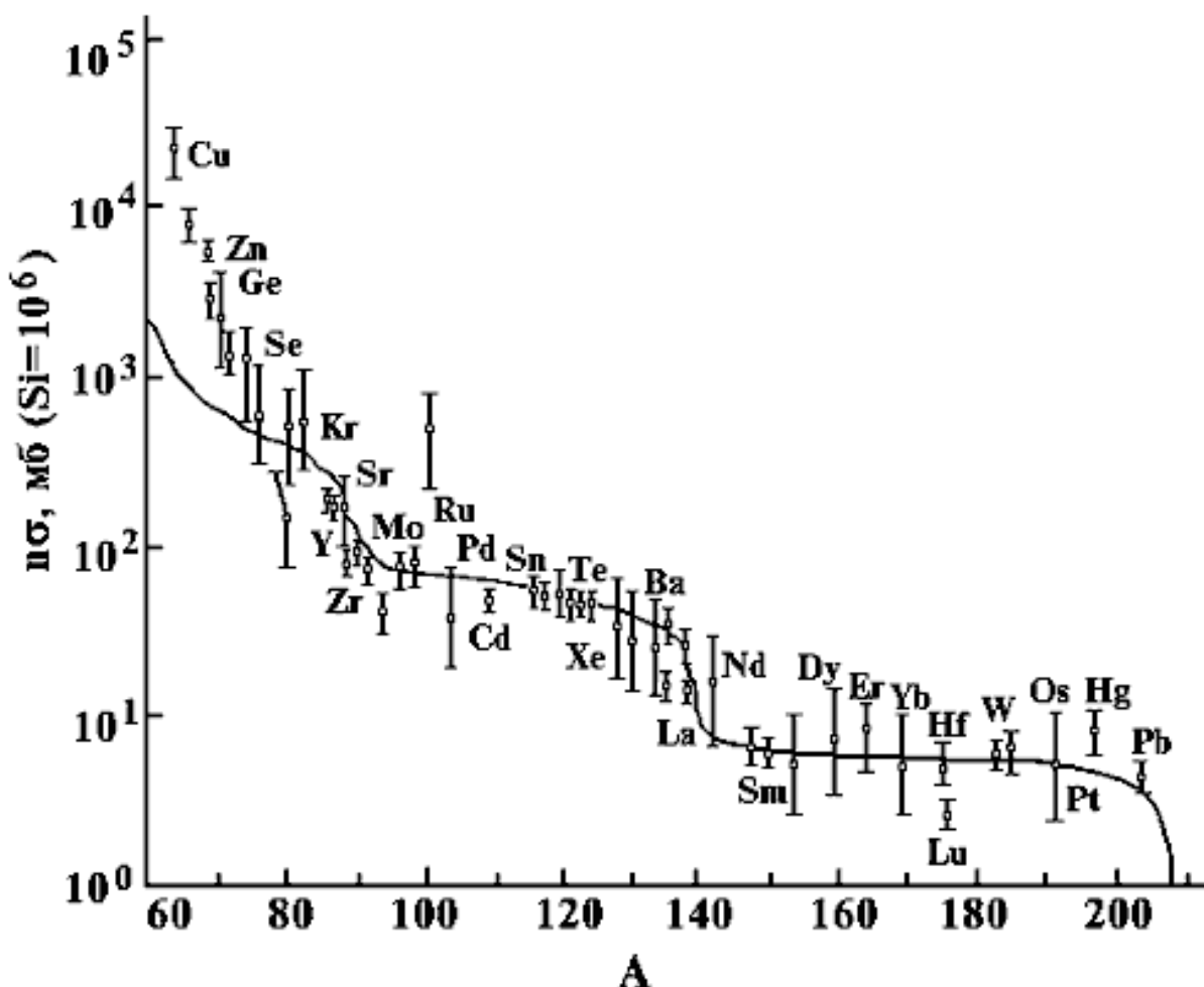
Rasm 5. Quyosh sistemasi elementlari uchun n\sigma -ni A -ga bog'lanishi.
