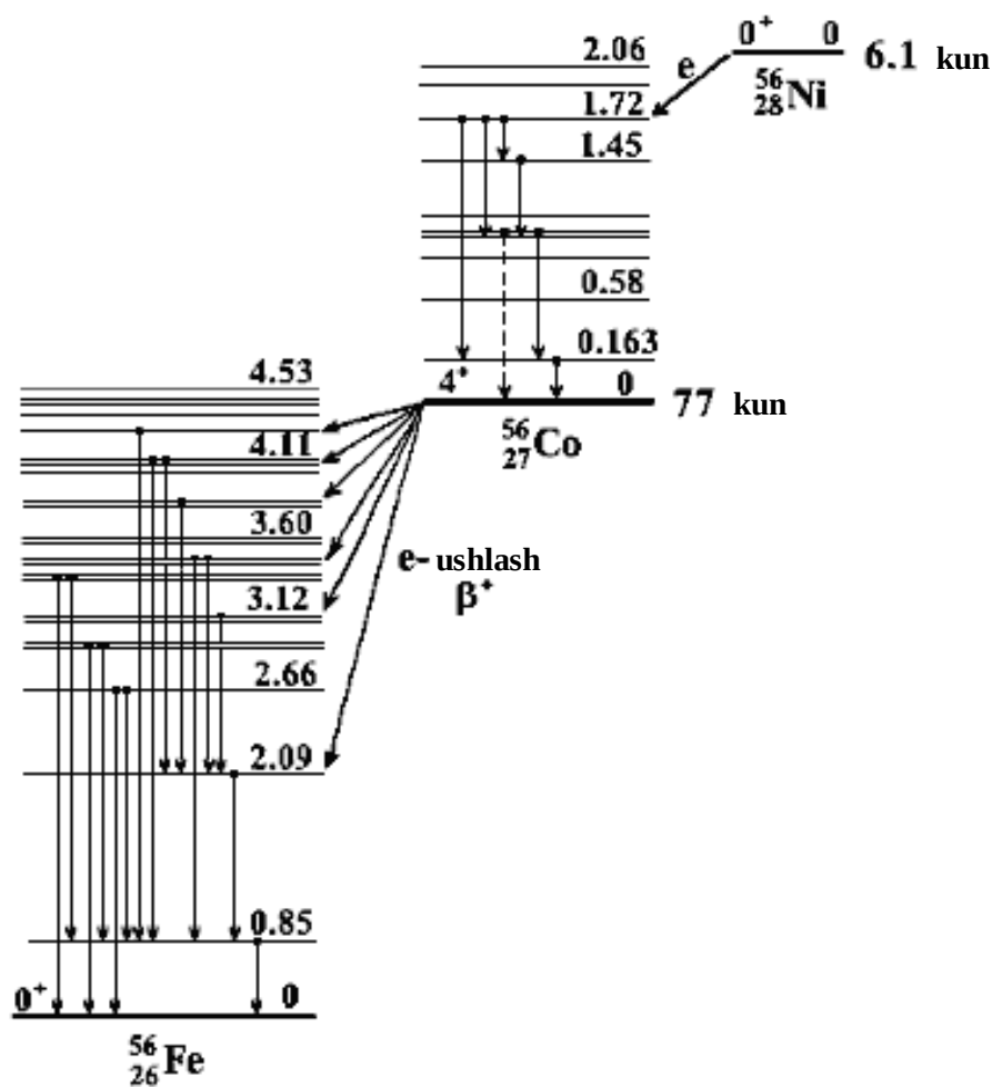
Rasm – 7a. Ni^{56} \rightarrow {}^{56}Co \rightarrow {}^{56}Fe zanjirida \beta va \gamma o'tishlarining sxemasi. Energetik sathlar ustida yadroning qo'zg'alish energiyasi MeV da keltirilgan. Asosiy holatlar uchun spini va yarim emirilish davri ko'rsatilgan.
