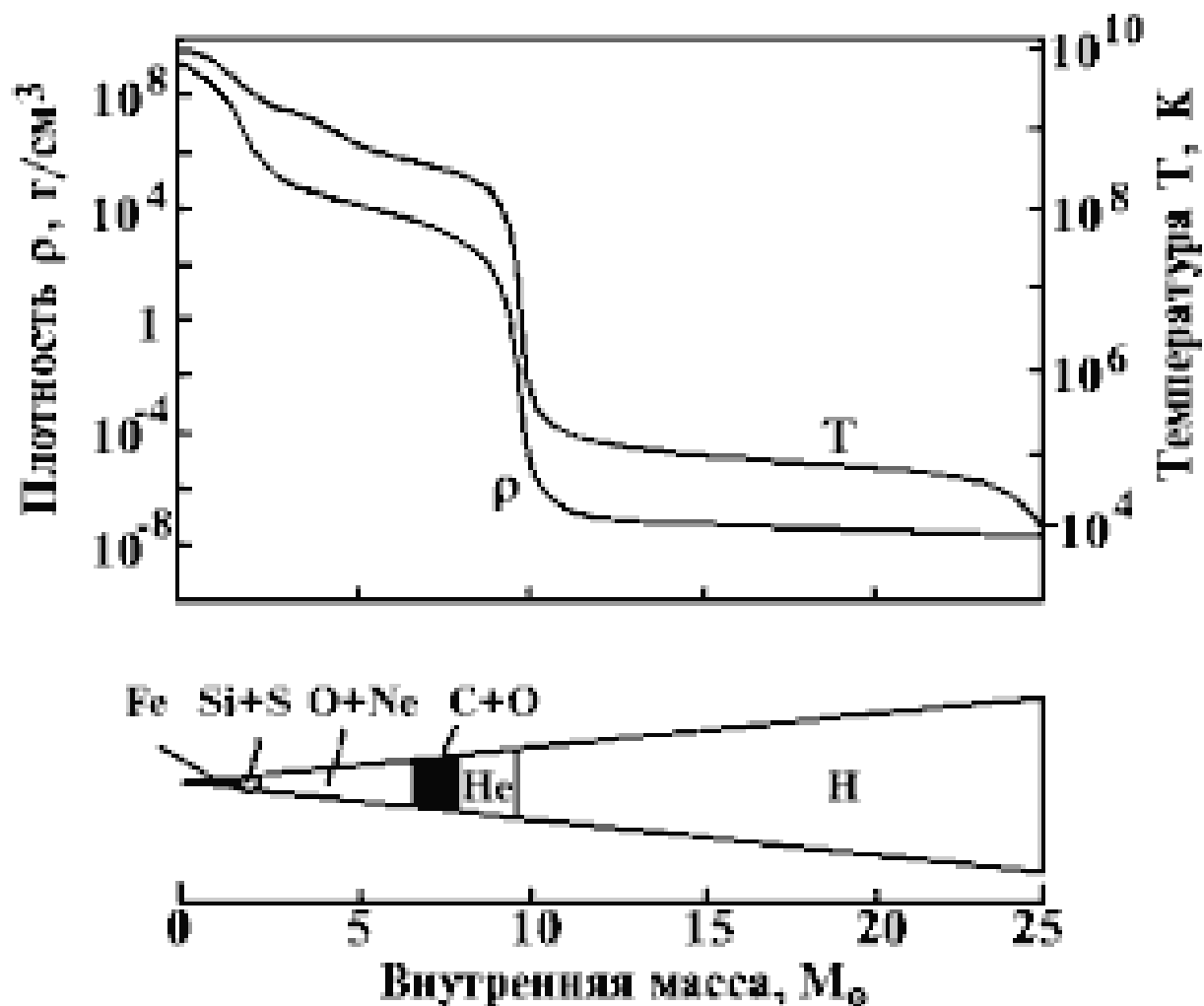
Rasm 8. Massiv yulduzning evolyutsiyasi oxirida gravitatsion kollapsdan oldin xarakterli tuzilishi.
