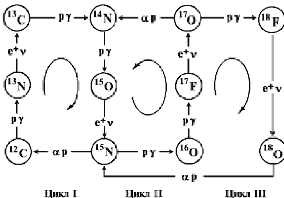
Rasm 4. Massasi 5 M_0 bo'lgan yulduzning uglerod yona boshlanishi momentidagi ximiyaviy tarkibi keltirilgan. Yulduz tarkibidagi C, He va H uning umumiy massasi ulushida ko'rsatilgan.
