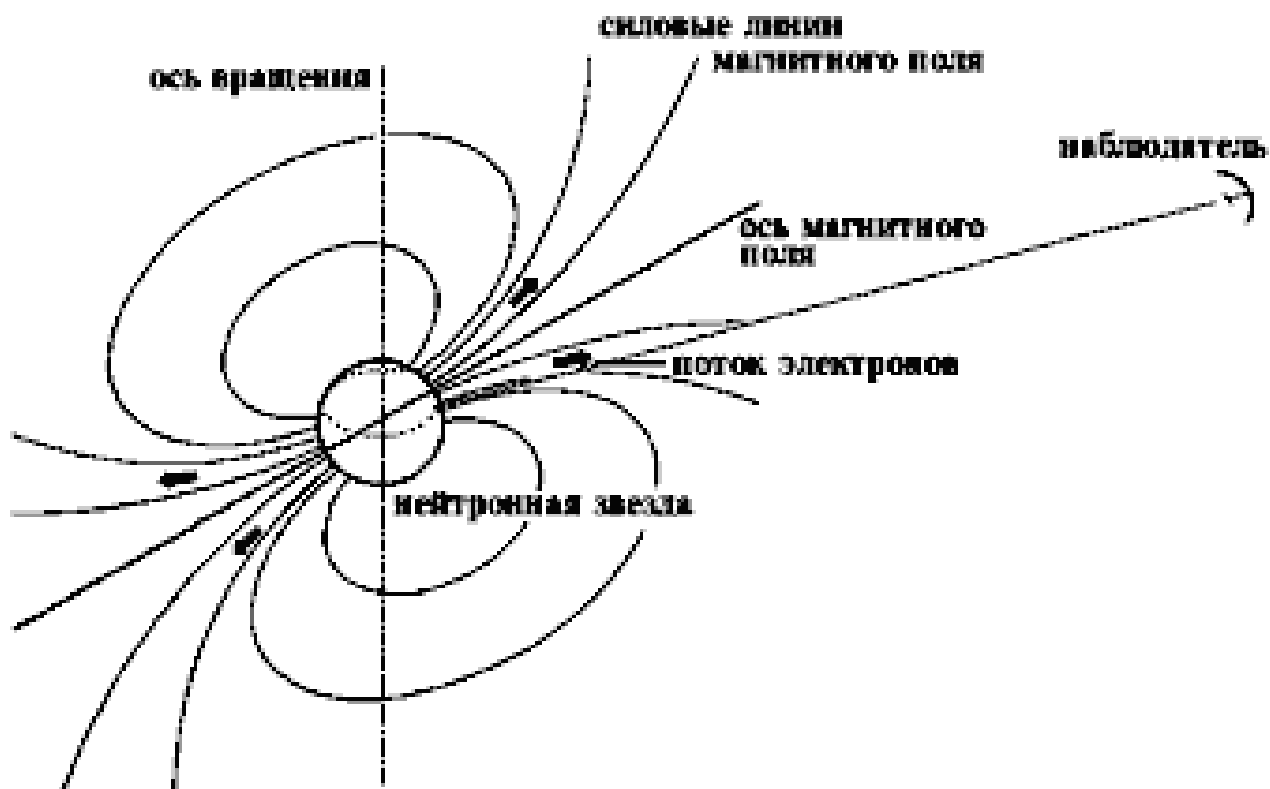
Rasm 9. Pulsar modeli.
