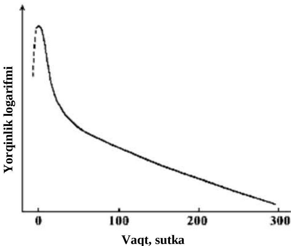
Rasm 6. I-chi tipdagi o'ta yangi yulduz yorqinlik chizig'i.
