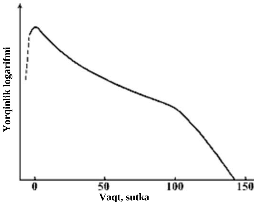
Rasm 7. II-chi tipdagi o'ta yangi yulduz yorqinlik chizig'i.
