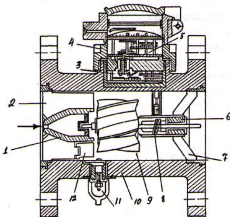
55- rasm. Spiralsimon parrakli tezlik hisoblagichi.
