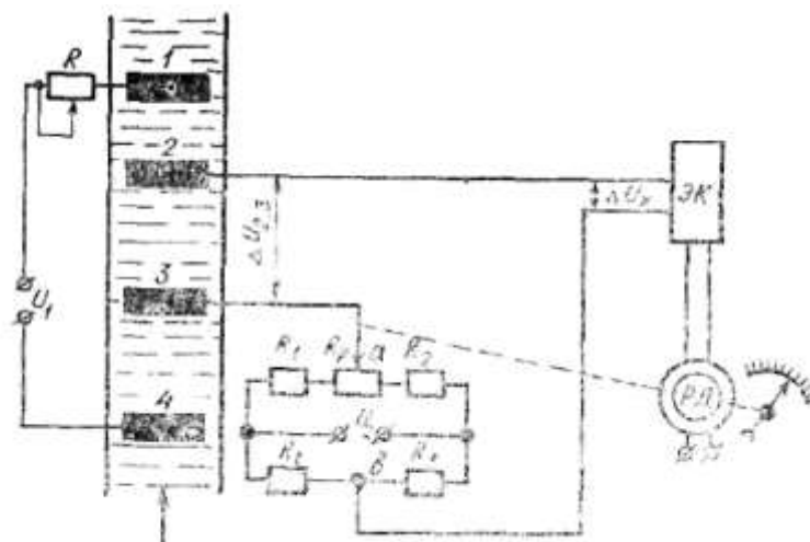
69- rasm. Turt elektrodli ulchash yacheykasi bo'lgan kenduktsmetrning sxemasi.
