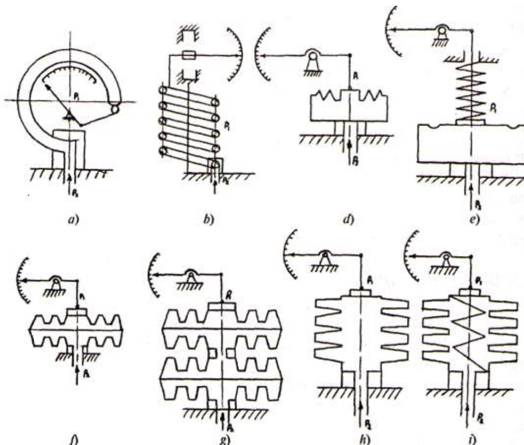
41 – rasm. Deformatsion (pujinali) manometrlarning sezgir elementlari.
