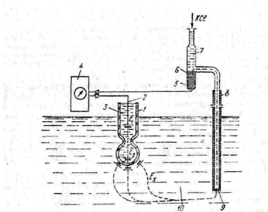
73- rasm. Shisha va elektrolari bo'lgan pH – metr
