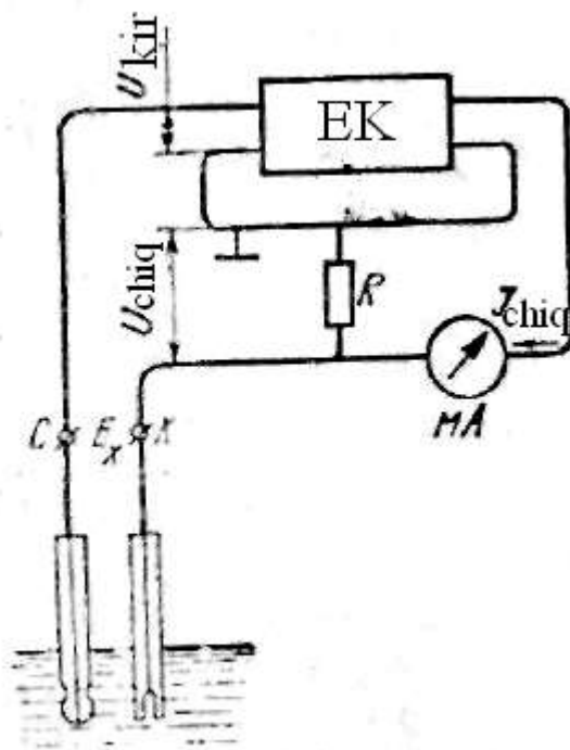
75- rasm. Elektrod sistemi EYuK ini uzgartkich P-201 bilan o'lchash sxemasi
