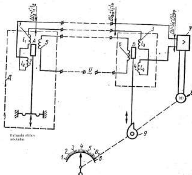
94-rasm. Differensial-transformatorli uzatish sistemasining prinsipl sxemasi.
