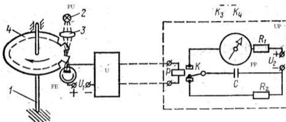
104- rasm. Chastota - impul'sli sistemasini prinsipial sxemasi.
