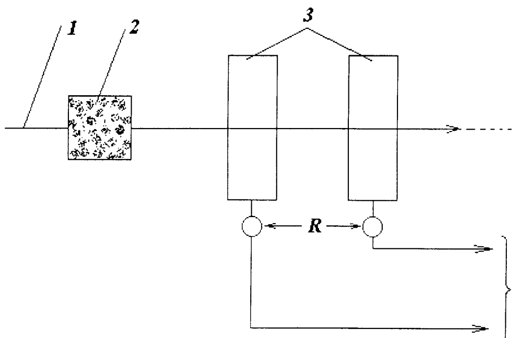
14- rasm. Iplar qalinligini o'lchash sxemasi
