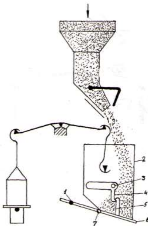
58-rasm. Osti ochiladigan cho'michli avtomat tarozi.
