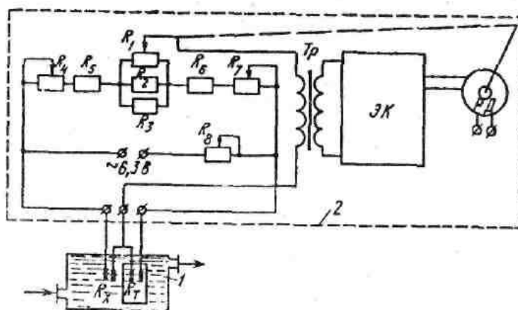
70- rasm. Sul'fat kislota konsentratomerining prinsipial sxemasi
