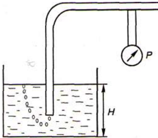
65- rasm. P'ezometrik zichlik o'lchagichning printsipl sxemasi.
