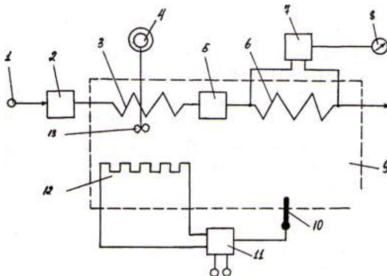
76 - rasm. Avtomatik kapillyar viskozimetrning struktura sxemasi.
