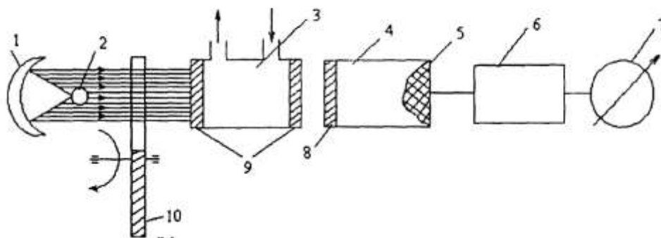
79 - rasm. Optik-akustik analizatorining printsiptial sxemasi.
