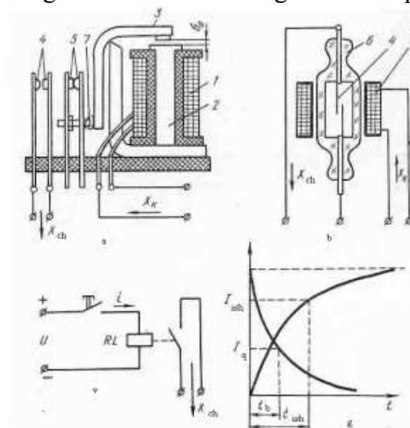
83- rasm. O'zgarimas tok relesi: a-aylanuvchi yakorli rele; b-yakorsiz rele (gerkon); v- relening elektr sxemasi; g - relening dinamik tavsif grafiklari; 1 -elektromagnit g'altagi (o'ramasi), 2 – qo'zg'almas po'lat o'zak; 3-o'zak (yakor), 4 - toksiz holatdagi ochiq kontakt, 5 - toksiz holatdagi yopiq kontakt, 6-shisha kolbacha.
