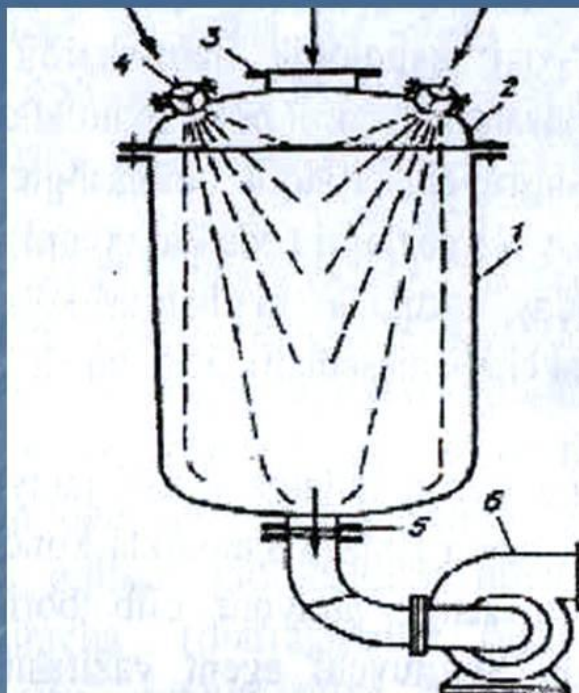
Тўғри йўналишли аралаштирувчи конденсатор: 1-қобик; 2-қопқоқ; 3-буғ потрубкеси; 4-соплю; 5- сув ва ҳаво чиқарувчи потрубка; 6-насос.
