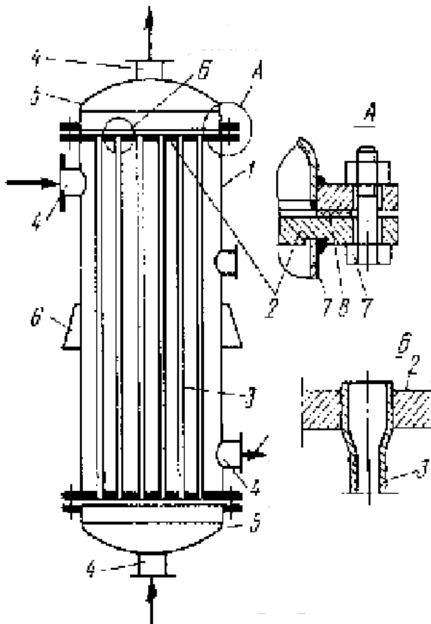
9- расм. Бир юлли қобиқ трубали конденсатор: 1- қобиқ; 2- труба турлари; 3 - трубалар; 4- қопқоф; 5,6 - иссиқлик агентлари кирадиган ва чиқадиган штуцерлар; 7- болт; 8- қистирма.
