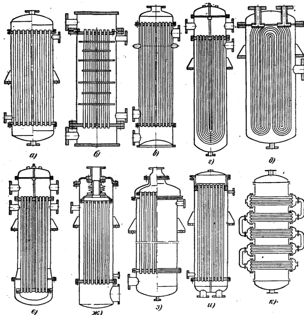
4-расм. Қобик труба иссиқлик алмашиниш қурилмалари.
