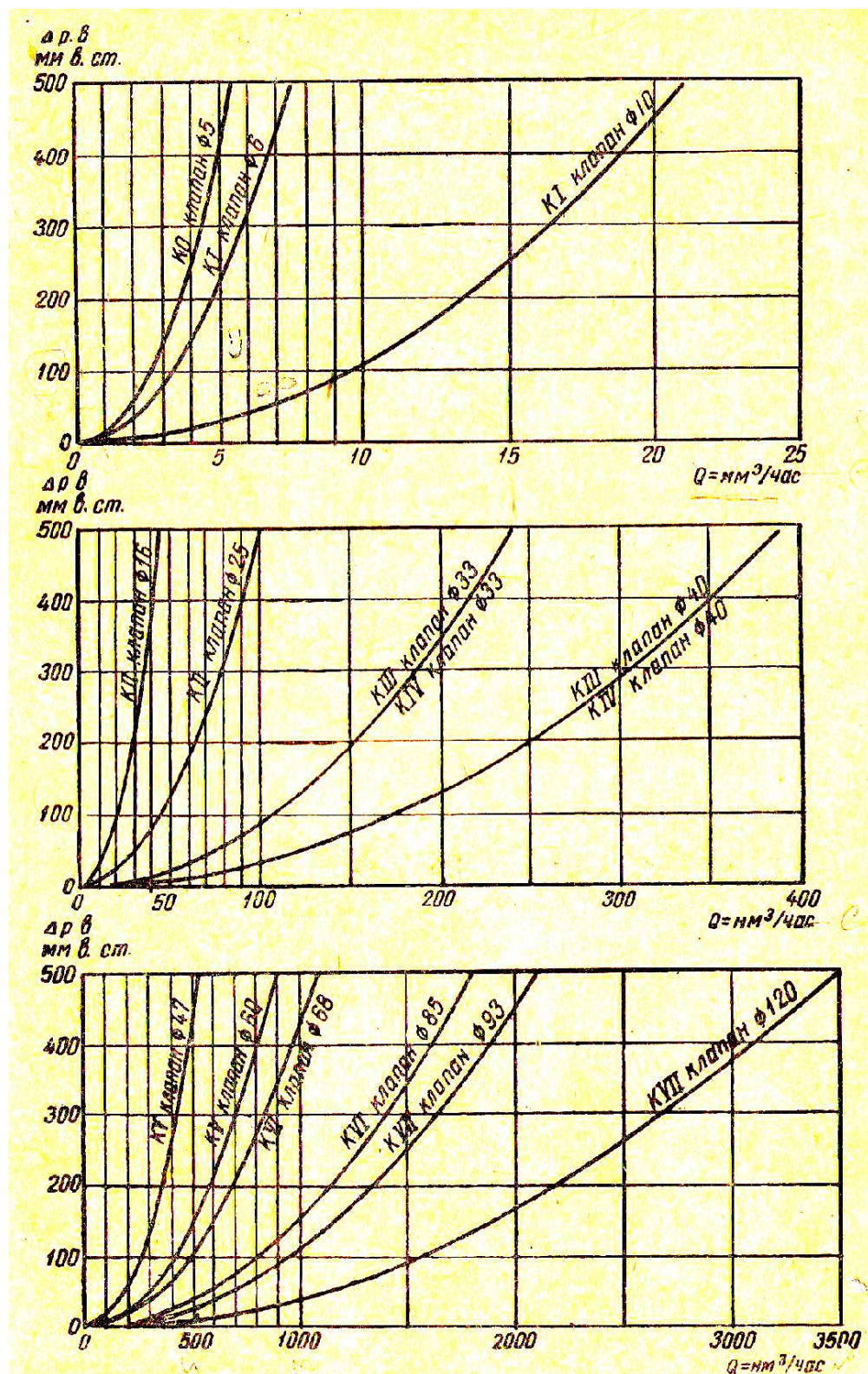
3.2-расм. “К” типли босимни бошқарувчининг таснифи.
