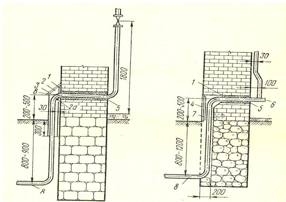
3.11-расм. Бинога газ тармоқларини киритиш ва монтаж қилиш:
