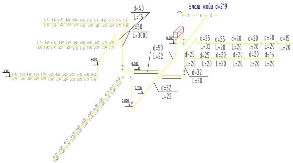
Икки босқичли таъбиий газ тармоғини аксионометрик кўриниши
