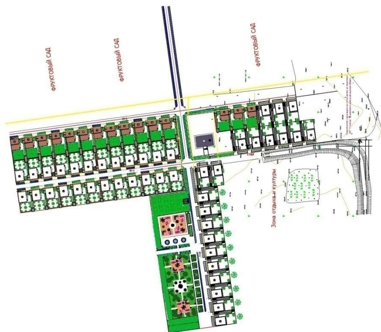
2.2-расм. Уч босқичли газ тармоғининг бош режаси.
