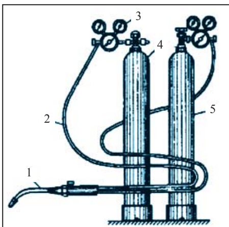
26-su'wret. Gaz benen kepslerlew ushi'n u'skeneler: 1-gorelka; 2-shlanglar; 3-reduktor; 4-kislorodli' ballon; 5-acetilenli' ballon.
