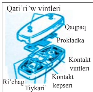
75-su'wret. Aspa aji'rati'p-qosqi'shti'n' du'zilisi.
