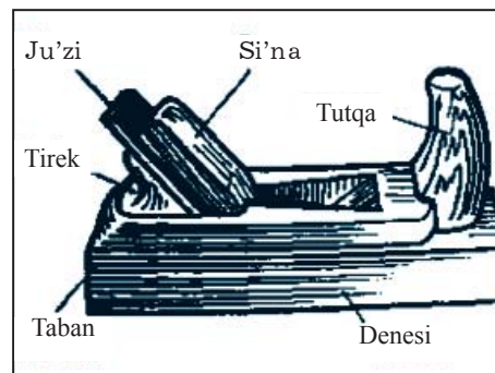
51-su'wret. Su'rginin' du'zilisi.
