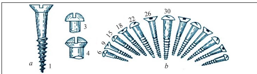
64-su'wret. Burama shegeler: a) shege yepelikleri: 1-jasi'ri'n; 2-yari'm jasi'ri'n; 3-yari'm domalaq; b) burama shegelerdin' wo'lshepleri.
