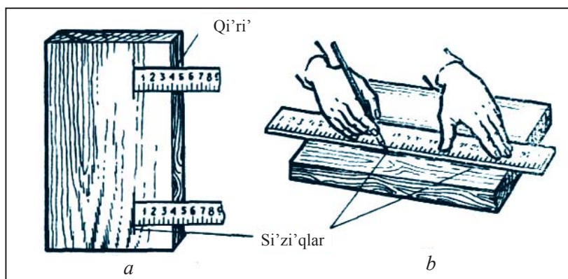
40-su'wret. Masshtabli' si'zg'i'sh ja'rdeminde detaldi' rejelew: a) detaldi'n' yenin wo'lshe'w; b) reje si'zi'g'i'n wo'tkeriw.
