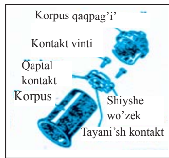
77-su'wret. Aspa patronni'n' du'zilisi.
