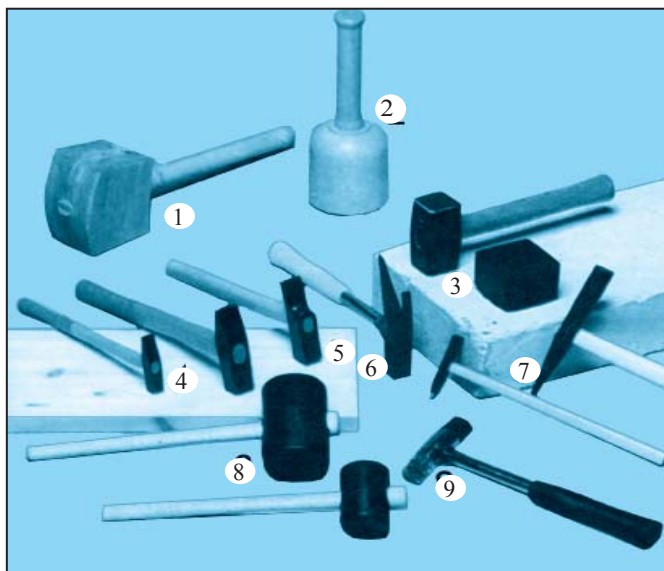
13-su'wret. Slesarli'q balg'alari' ha'm ag'ash toqpaq: 1,2 – ag'ash balg'alar; 3,4,5,6,7 – polat balg'alar; 8,9 – plastik balg'alar.
