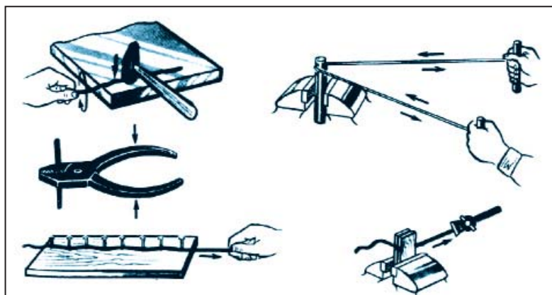
25-su'wret. Si'mlardi' tuwri'law usi'llari'.
