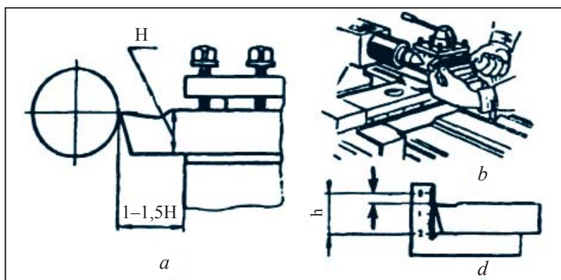
22-su'wret. Keskishti wornati'w: a ) keskish ha'm woni' jaylasti'ri'w; b ) keskishtin' biyikligin tekseriw; d ) mu'yeshli shablon.
