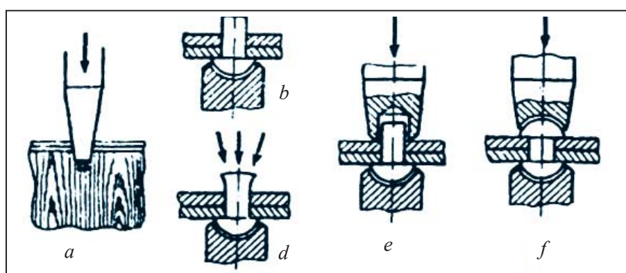
29-su'wret. Toytarmali' jalg'aw procesinin' izbe-izligi.
