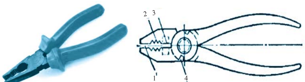
12-su'wret. Slesarli'q atawi'zlar: 1 – tegis qi'siwshi' bo'limi; 2 – cilindr formasi'ndag'i' buyi'mlardi' qi'si'p uslap turi'w ushi'n mo'lsherlengen dog'a ta'rizli bo'legi; 3 – kesuwshi ju'zleri; 4 – domalaq kesimge iye si'mlardi' qi'rqi'w ushi'n woyi'qsha.
