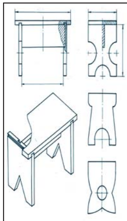
67-su'wret. Kursini tayarlaw si'zi'lmasi'.
