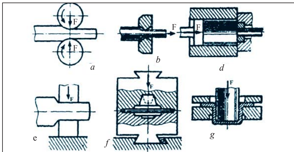
23-su'wret. Basi'm menen metallarg'a islew beriw: a) prokatka; b) sozi'p ali'w; d) presslew; e) qi'zdi'ri'p balg'a menen islew beriw; f) i'ssi'li'q ko'lemli shtampovka; g) suwi'q listli shtampovka.
