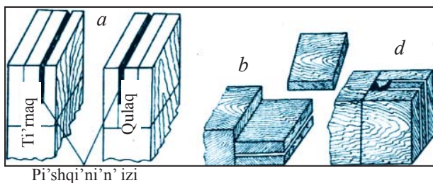
63-su'wret. Ti'rnaqti' jasaw ha'm qulaq ashi'w: a) ti'rnaq ha'm qulaqlardi' tiliw; b) ti'rnaqti' kertiw; d) qulaqti' woyi'w.
