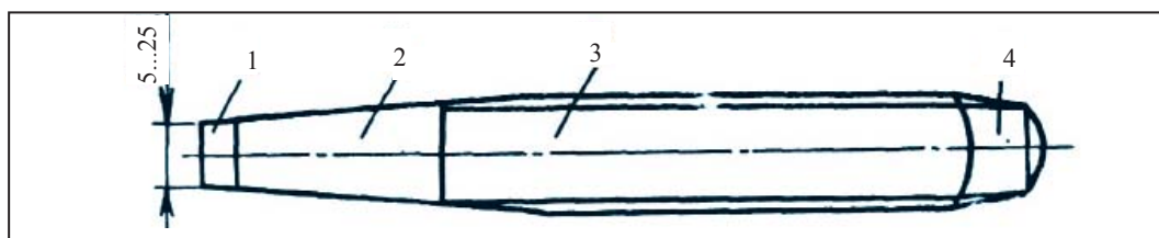
10-su'wret. Tokarli'q zubilosı'. 1–ju'zi. 2–jumi's bo'limi. 3–worta bo'limi. 4–basi'.
