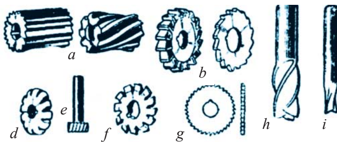
9-su'wret. Frezalardi'n' tu'rleri: a) cilinr ta'rizli; b) diskli; d) bo'rtik; e) pazli'; f) do'n'es; g) mu'yeshli; h) qi'rqi'wshi'; i) ushli'.
