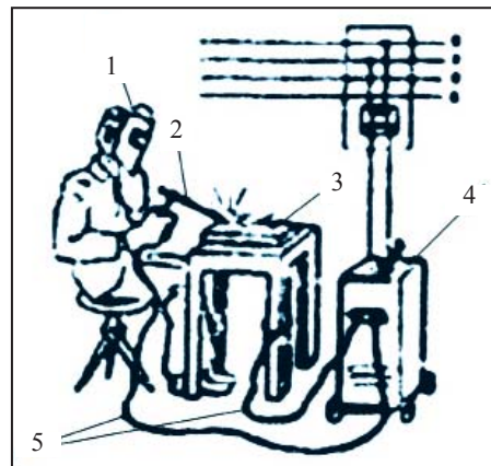
27-su'wret. Elektr kepslerew ushi'n u'skeneler: 1-qorg'awshi' maska; 2-elektrod; 3-buyi'm; 4-kepslerew apparati'; 5-si'mlar.
