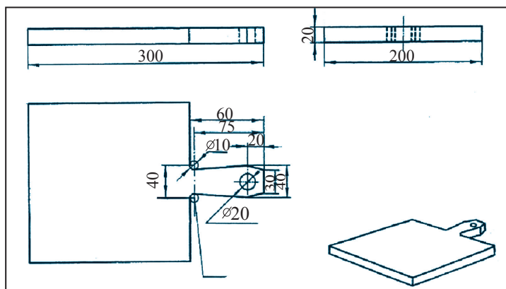
61-nji surat. Gök önümler dogralýan tagtany taýýarlamagyň çyzgysy.
