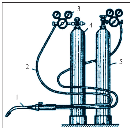
26-njy surat. Gaz bilen kebşirlemek üçin enjamlar: 1 – gyzdyryjy; 2 – şlanglar; 3 – reduktor; 4 – kislorodly ballon; 5 – asetilenli ballon.
