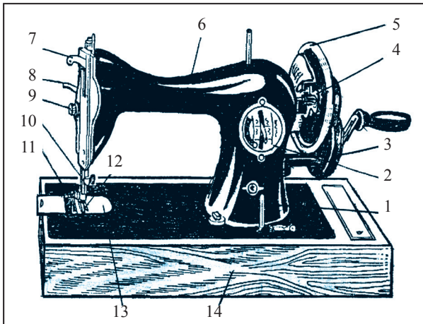
27-nji surat. El ýöretmeli tikin maşynynyň esasy bölekleri.
