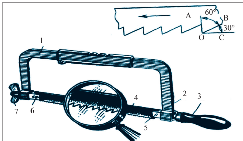
8-nji surat. Desseli slesarçylyk byçgysy: 1 – esas (ramka); 2 – guýruk; 3 – desse; 4 – polotnosy; 5 – ştift; 6 – çekiji wint; 7 – gulakly gaýka.
