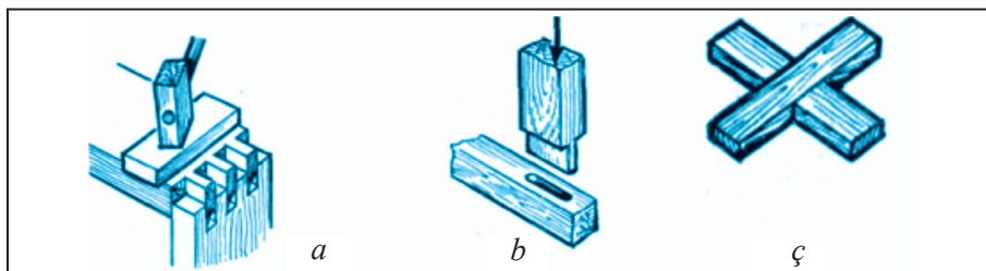
62-nji surat. Dyrnakly birikmeleri gurnamak:
