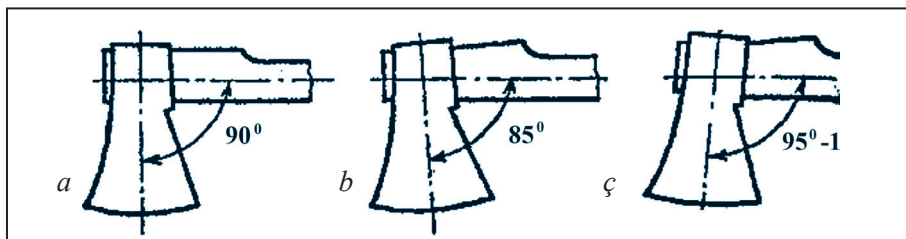
56-njy surat. Paltanyň tygynyň dessä görä ýerleşşi: a) göni burç astynda (odun aýyrmak üçin); b) ýiti burç astynda (şahalary çapmak üçin; ç) kütäk burç astynda (daragty birneme çapyp goýmak üçin).
