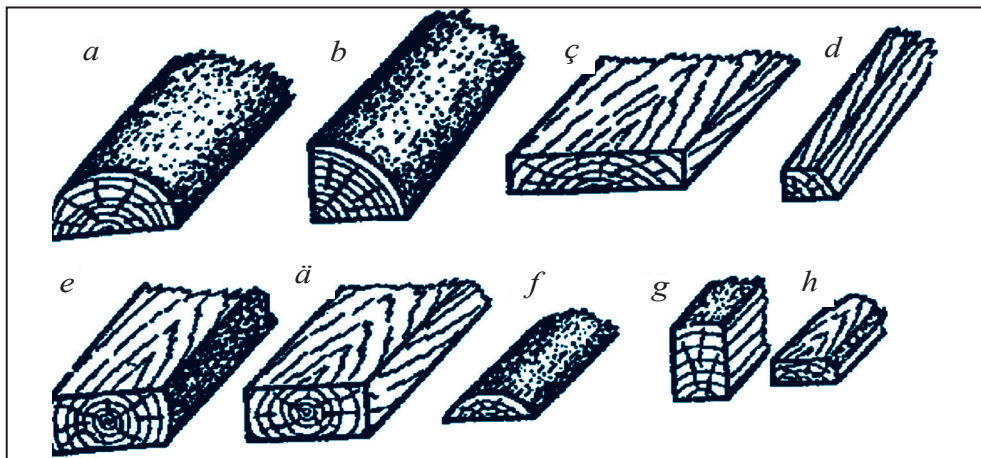
33-nji surat. Byçgylan materiallaryň nusgalary: a) plastinka; b) çärýeklik; ç) arassalap kesilen tagta; d) çeti gyrkylan reýka; e) iki gyraňly brus; ä) arassalap kesilen brus; f) kapantagta; g) üç gyraňly brus; h) şpala.
