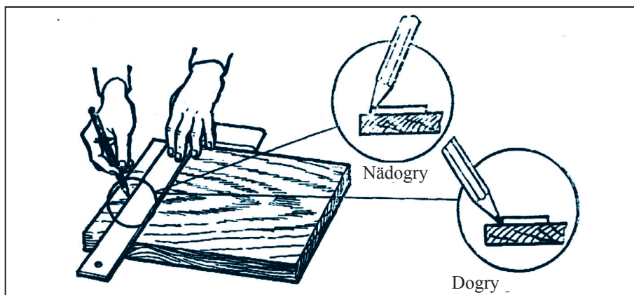
41-nji surat. Burçlugyň kömeginde çyzyklary geçirmek.
