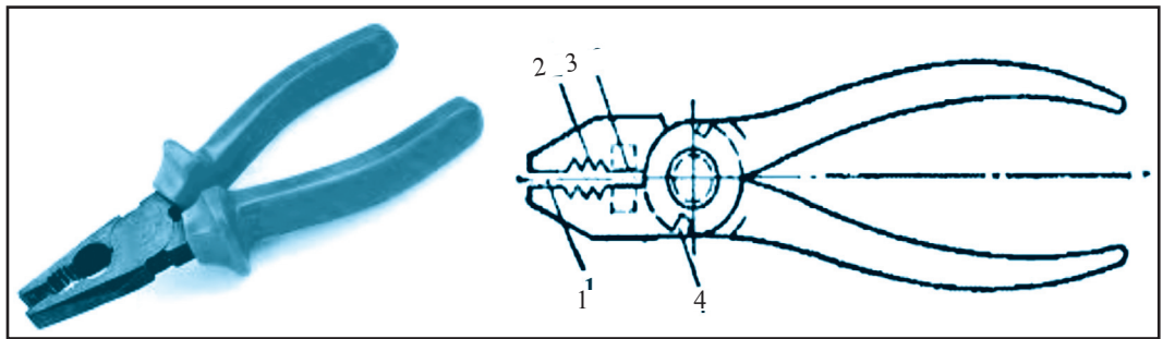
12-nji surat. Slesarçylyk atagzy: 1 – ýasy gysyjy bölegi; 2 – silindr şekilindäki zatlary berk saklap durmak üçin niýetlenen ýoý şekilli bölek; 3 – kesiji tyglar; 4 – togalak kesikli simleri gyrkmak üçin oýuk.
