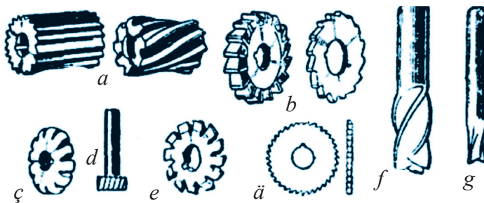
9-njy surat. Frezanyň görnüşleri: a) silindr şekilli; b) diskli; c) düwürtikli; d) pazly; e) güberçekli; ä) burçly; f) gyrkyjy; g) uçly.
