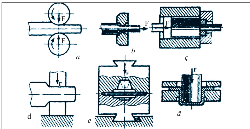
23-nji surat. Basyş bilen metallary işläp bejermek: a) prokatlama; b) sozma; ç) dykyzlandyrma; d) gyzdyryp çekiçde işläp bejermek; e) yssy göwürimli ştamplama; ä) sowuk listli ştamplama.
