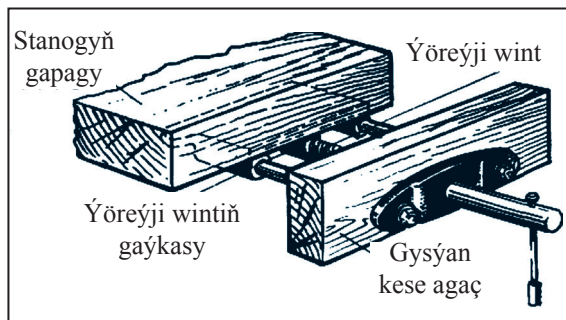
38-nji surat. Neçjarçylyk werstagynyň isgenjesi.
