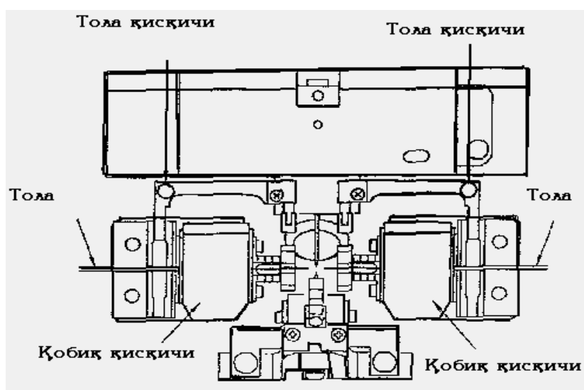
1.11-Расм. Толани пайвандлаш аппаратиға тўғри жойлаштирши.
