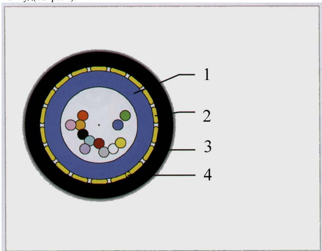
6.3. – расм. A-DQ(BN)H 1х12 русумли кабел.
