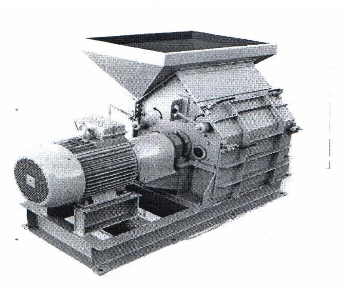
6-расм. Дон янчгич машинаси
