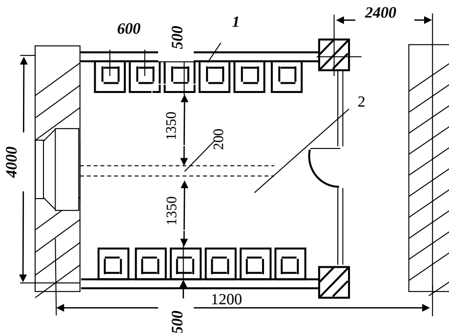
12.5-рasm. ... виниш хонаси схемаси
