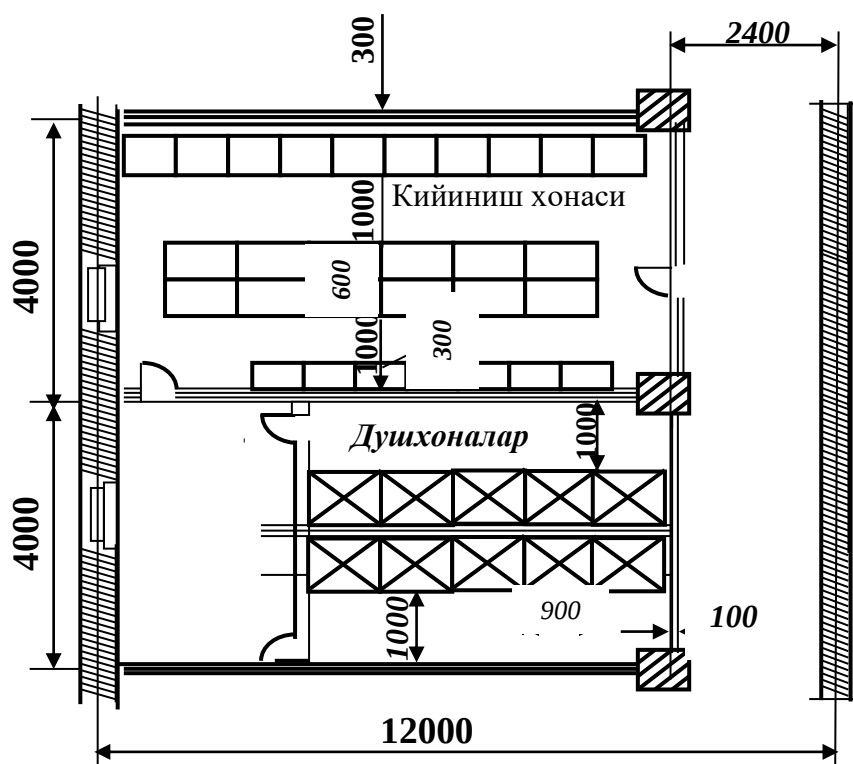
12.6-рasm. Душхонанинг схемаси.
