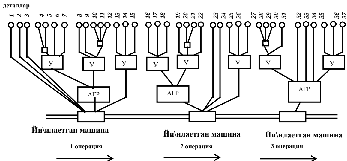
10.3-расм. Ҳаракатланувчи объектли оқим бўйича йиғиш схемаси
