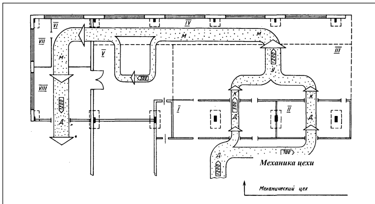
11.1-расм. Йиғув цехи юк ташиши технологик
