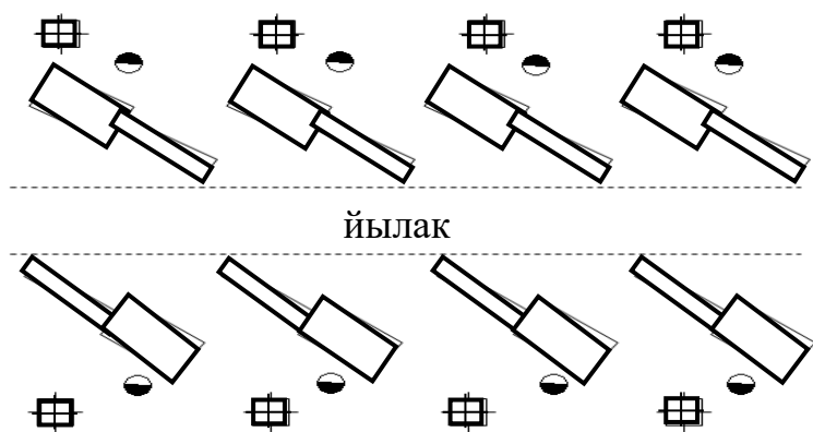
7.20-расм. Токарлик револьверли дастгоҳларни бурчак остида жойлаштириш
