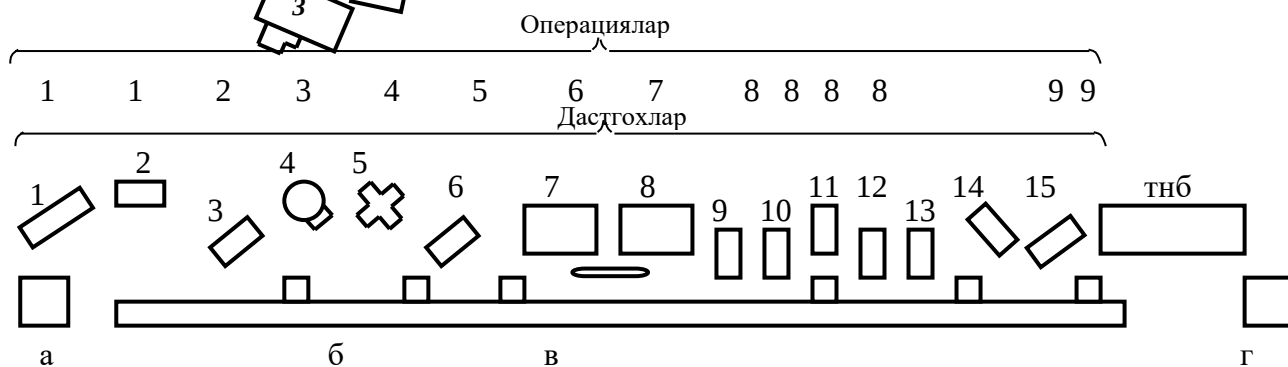
7.28-расм. Лентали конвейер қўлланган поршенларга ишлов берувчи оқим бўйича линия режасининг схемаси
