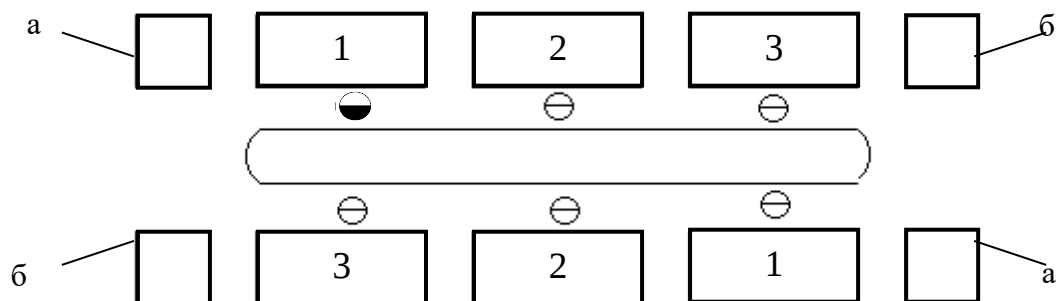
7.25-расм. Бир ишчини бир вақтнинг ўзида ишлаши учун 6 та дастгоҳни жойлаштириш а-заготовка, б-тайёр деталлар, 1,2,3 – операциялар
