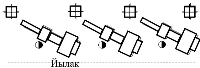
7.20-расм. Токарлик револьверли дастгоҳларни бурчак остида жойлаштириш
