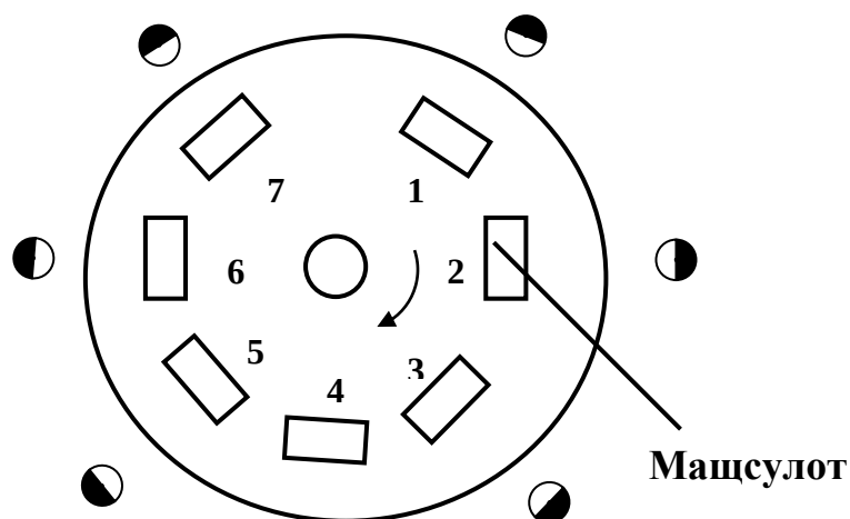
10.7-расм. Каруселли столда йиғиш схемаси
