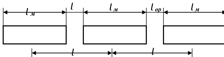
10.4-расм. Икки иш жойи ўқлари орасидаги масофани аниқлаш 1, 2, 3-йигилувчи машиналар
