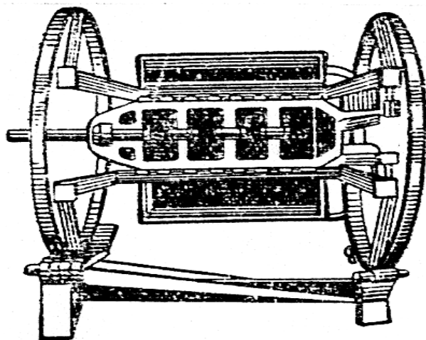
10.2-расм. Йиғиш вақтида маҳсулотнинг зарур ҳолатини таъминловчи буралувчи дастгоҳ
