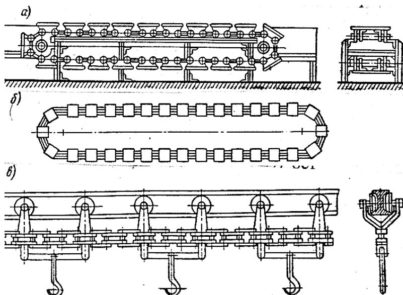
10.5-расм. Йиғиш ишлари учун конвейерлар схемаси
