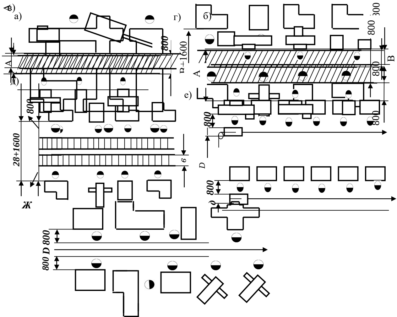
7.14-расм. Дастгоҳлар орасидаги йўлак кенглиги, линия дастгоҳлари билан осма ва ер усти конвейерлари орасидаги масофалар
