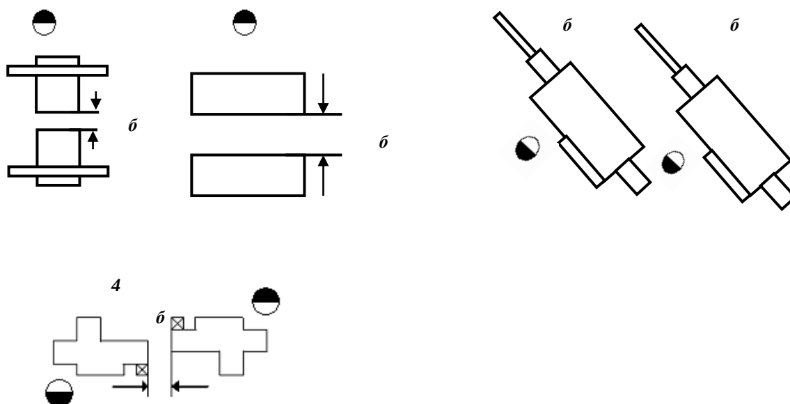
7.6-расм. Дастгоҳларнинг бир-бирига орқа томони билан жойлаштирганда «б» ўлчам қиймати
