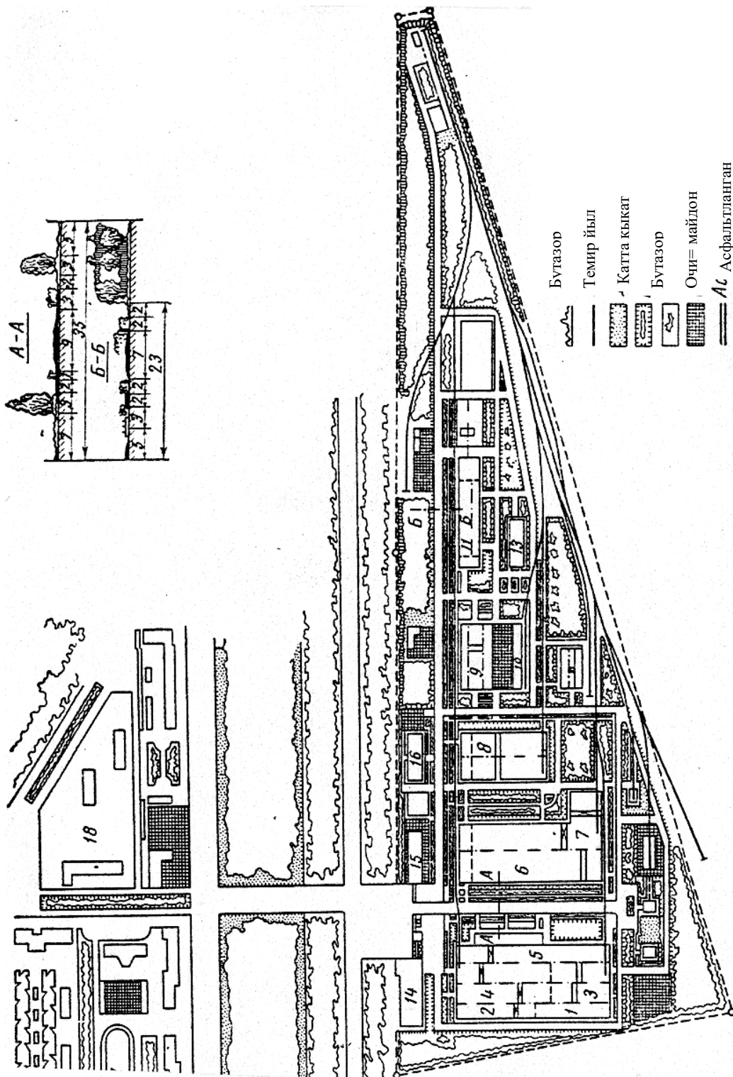
2.1-расм. Машинасозлик корхонасининг бош режаси
