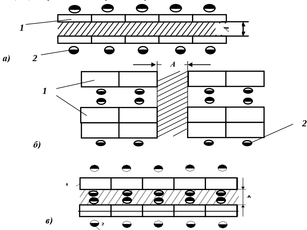
10.9-расм. Верстаклар орасида йўлак ва йўлкаларни жойлаштириш схемаси
