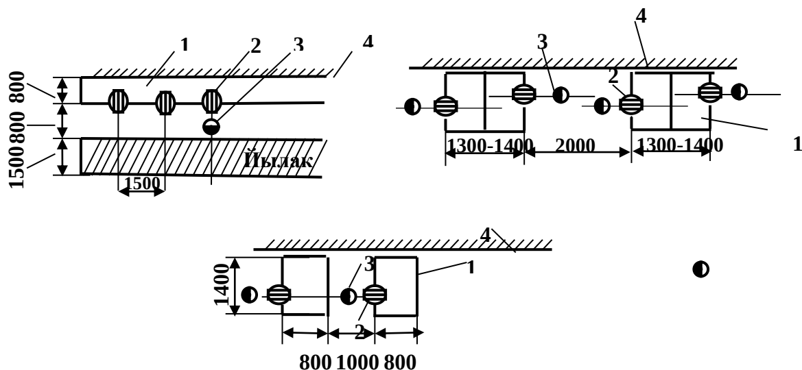
10.8-расм. Чилангарлик верстакларини жойлаштириш схемаси
