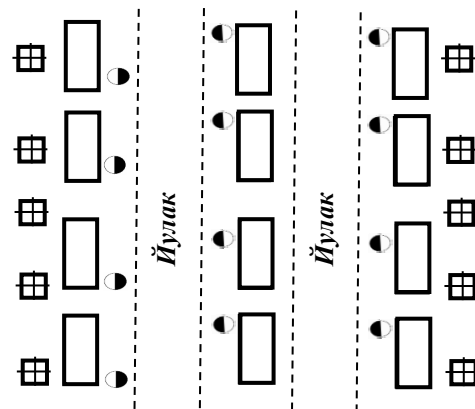
7.16-расм. Дастгоҳларни уч қатор жойлаштириш
