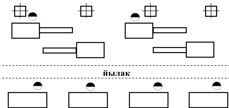
7.22-расм. Токарлик револьверли дастгоҳларни шахмат усулида жойлаштириш
