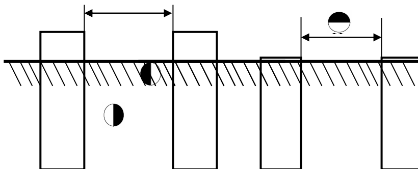
7.13-расм. Йўлакка нисбатан дастгоҳларнинг қўндаланг жойлаштиришдаги масофалар
