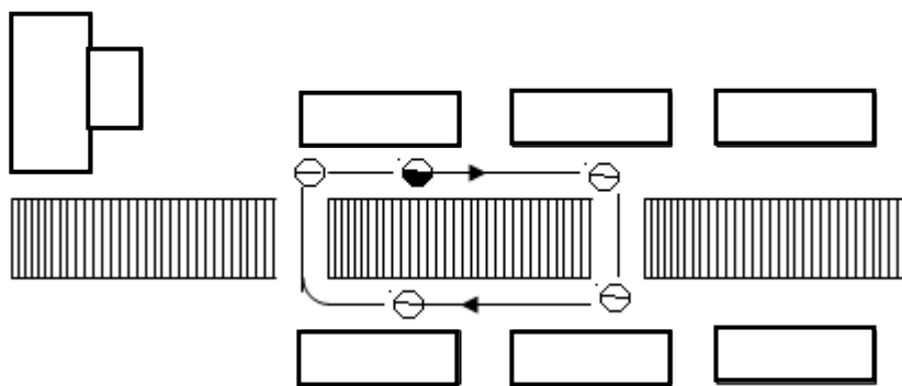
7.26-расм. Кўп дастгоҳли хизмат кўрсатишда рольганг атрофида дастгоҳларни икки қатор жойлаштириш
