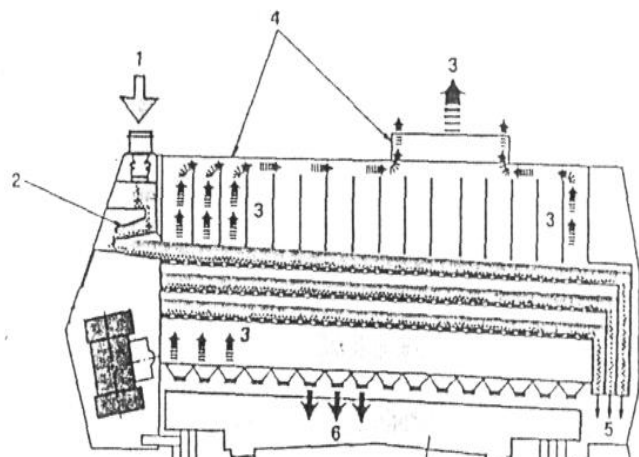
21- расм. "Пуромат" совуриш-элаш машинасининг узунасига кесии қирқими:
