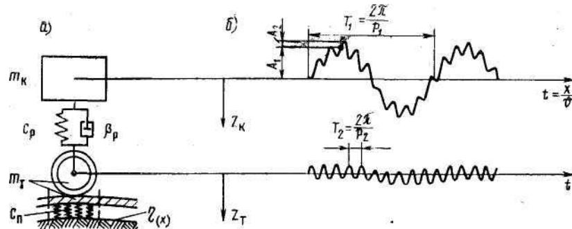
Рисунок 3.1. Схема для расчета симметричных колебаний вагона (а) и графики собственных колебаний масс кузова и тележек (б).
