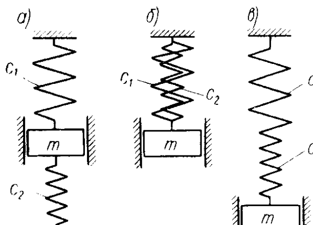
Рисунок 6.2. Динамические системы к задаче 6.4.1.
