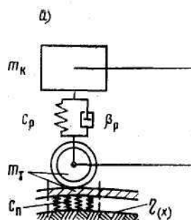
Рисунок 6.10. Расчетная схема к задаче 6.5.1.
