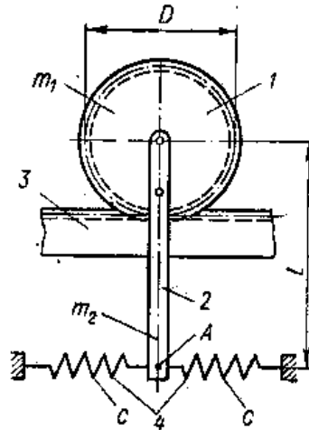
Рисунок 6.3. Зубчатое колесо на рейке.
