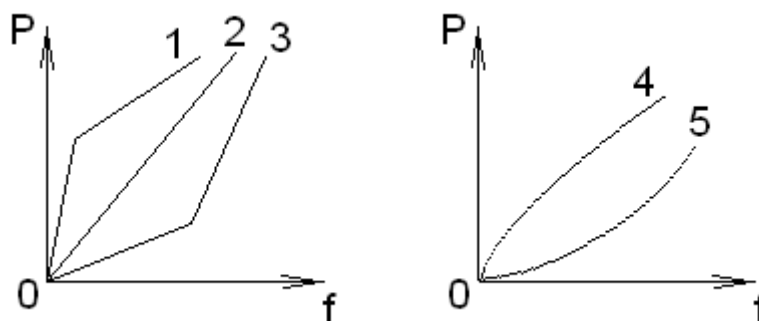
Рисунок 1.2. Силовые характеристики упругих связей.
