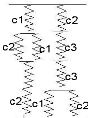
Рисунок 6.1. Комбинированное соединение пружин.
