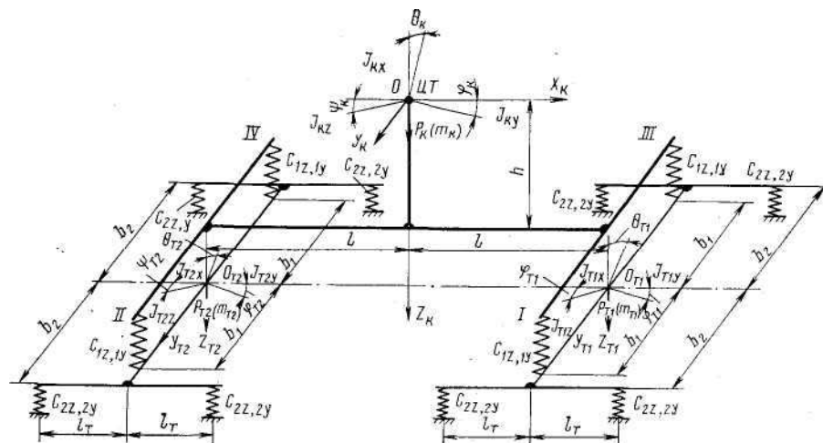
Рисунок 4.1. Расчетная схема вагона с двойным рессорным подвешиванием
