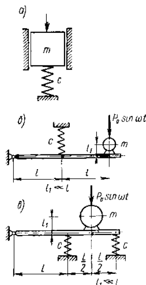
Рисунок 6.14. Схемы к задаче 6.5.5.
