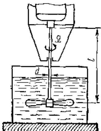
Рисунок 6.8. Динамические системы.
