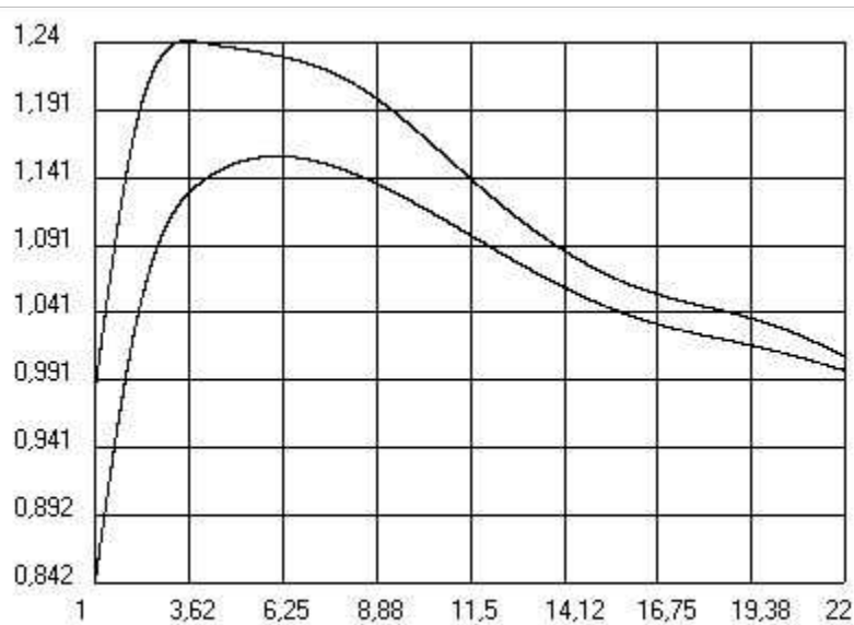
Рисунок 5.1. График значений коэффициента влияния частоты на утомляемость.
