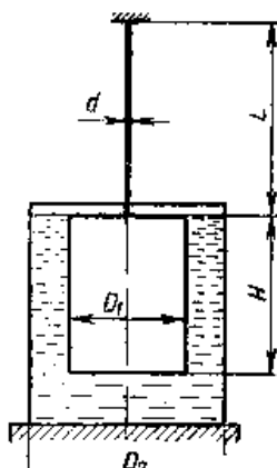
Рисунок 6.9. Динамическая система к задаче 6.4.8.
