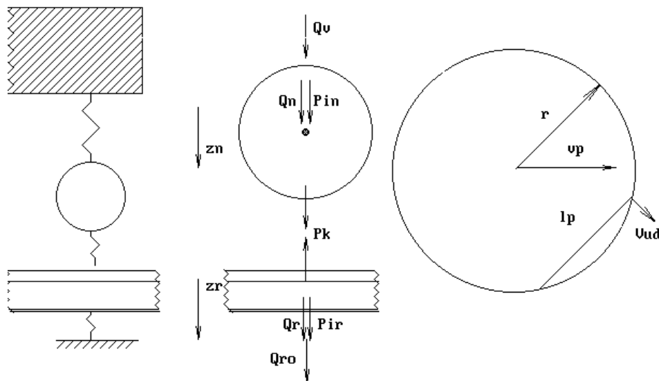
Рисунок 2.1. Расчетная схема удара колеса по рельсу.
