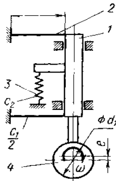
Рисунок 6.12. Схема датчика биений.
