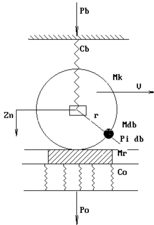
Рисунок 2.3. Расчетная схема движения несбалансированного колеса.
