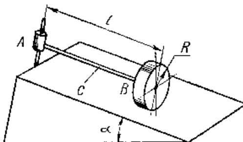
Рисунок 6.5. Динамическая система к задаче 6.4.4.
