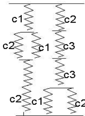
Рисунок 6.1. Комбинированное соединение пружин.
