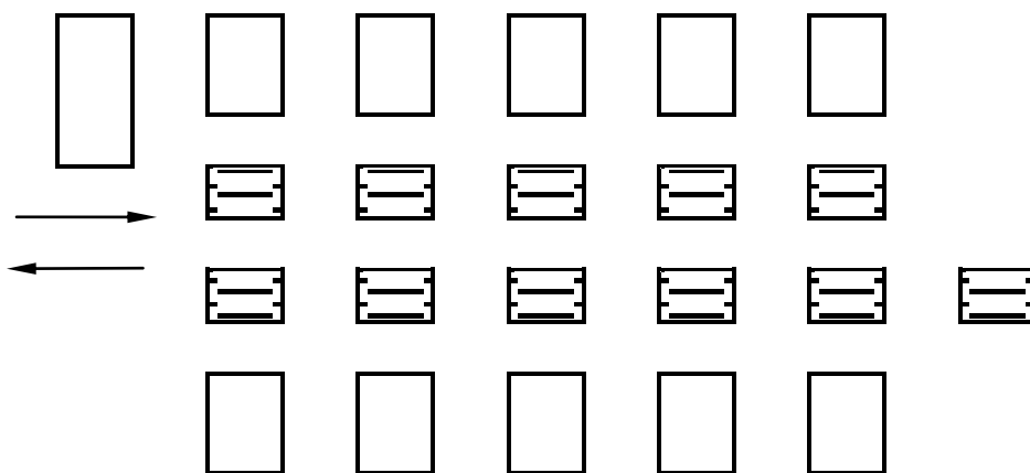
б) - Транспортировка пачек деталей в двухпозиционных зажимах 1р-15 Рис.1. Расположение рабочих мест в потоках при использовании средств транспортировки с режимом ДОО [4].
