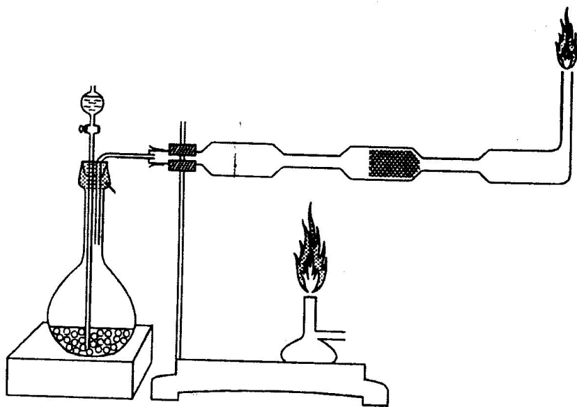
46-rasm. Oz miqdordagi mishyak birikmalarini tahlil qilish uchun ishlatiladigan qurilma.
