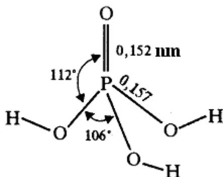
45-rasm. Ortofosfat kislota molekulasi tuzilishi.
