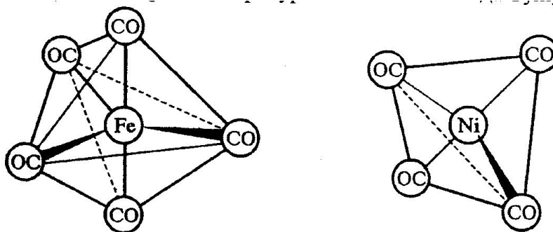
40- rasm. Temir va nikel karbonillarining tuzilishi.
