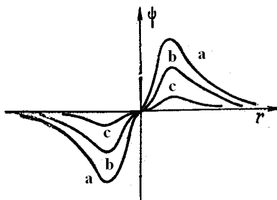
9-rasm. 2p elektronlarning to'liq funktsiyasi grafigi.
