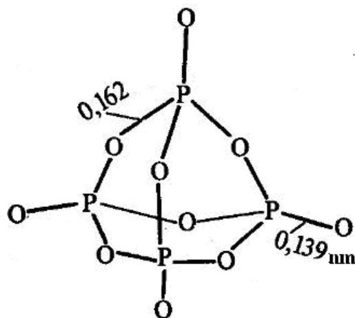
44-rasm. Fosfor (Y) oksid molekulasining tuzilishi.
