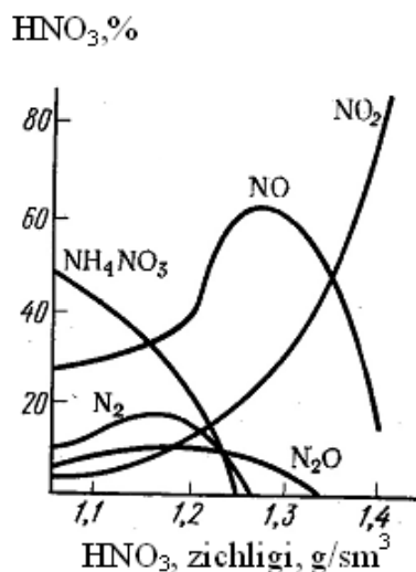
34-rasm. Temir bilan qaytarilishda nitrat kislota konsentratsiyasining qaytarilish mahsulotlariga ta'siri.
