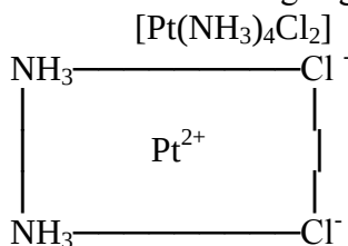
tsis - izomer
