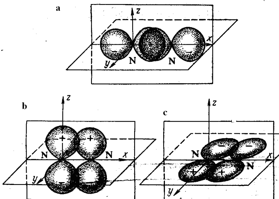
16-rasm. Azot molekulasidagi 2p -elektron bulutlarning qoplanishi.
