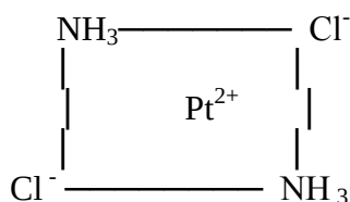
trans - izomer
