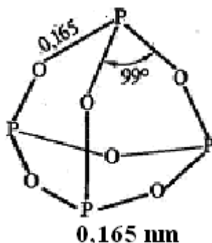
43-rasm. Fosfor (III) oksid molekulasi tuzilishi.
