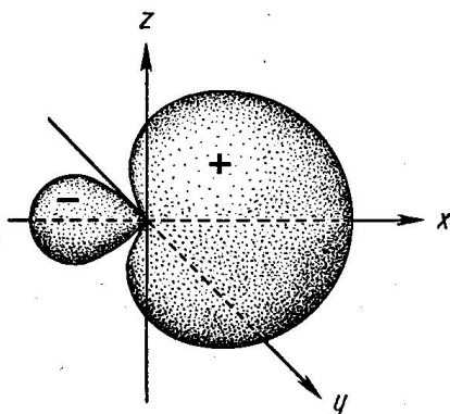
18. rasm. sp-gibrid orbitallarining alohida hosil bo'lish sxemasi.
