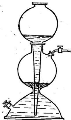
31-rasm. Vodorod olish uchun Kipp qurilmasi.
