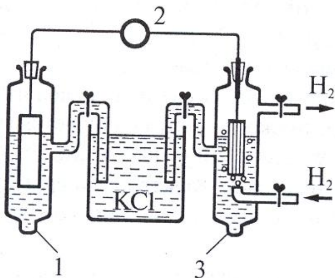
30-rasm. Noma'lum elektrodlar potensialini o'lchash uchun ishlatiladigan elektrodlar zanjirini ko'rinishi.
