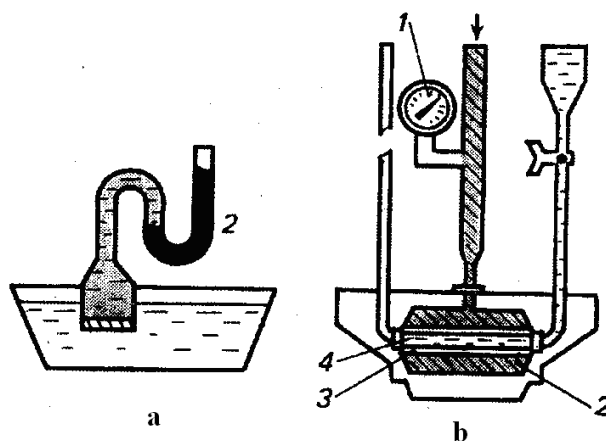
4-rasm. Osmotik bosimni o'lchashga imkon beruvchi uskuna.
