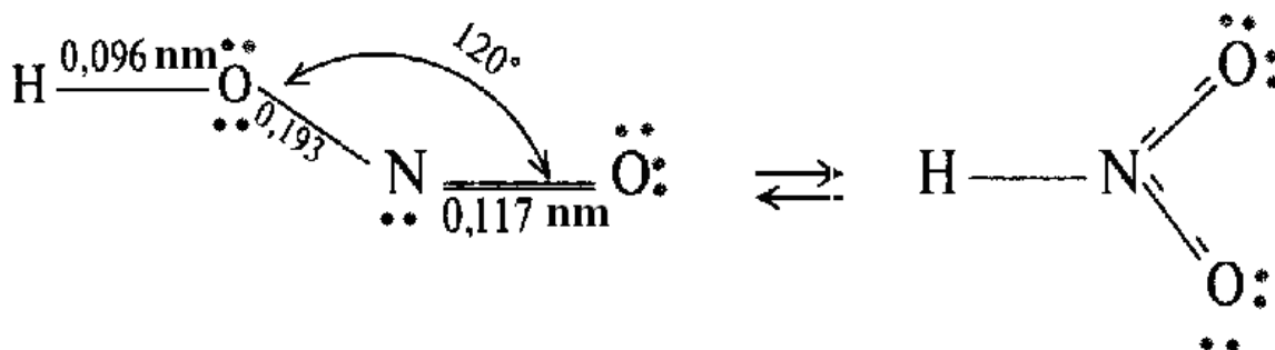
42-rasm. Nitrit kislota molekulasining tuzilishi.
