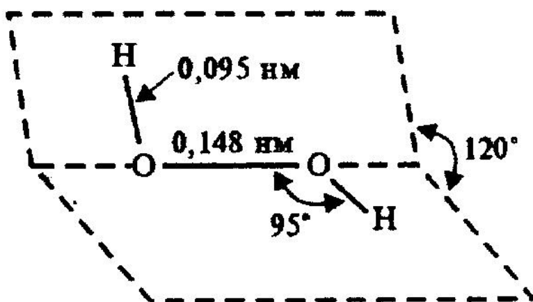
32-rasm. Vodorod peroksid molekulasining tuzilishi.
