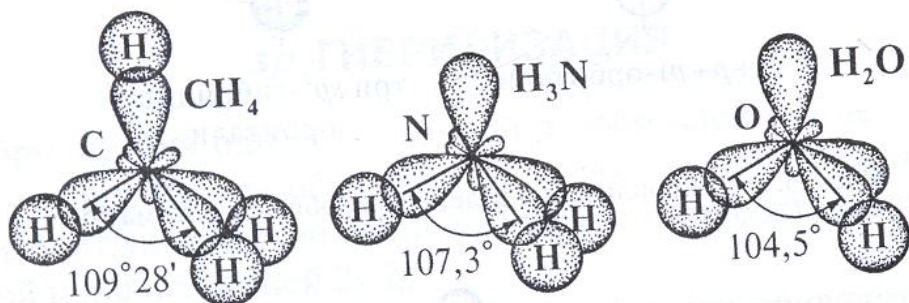
20-rasm. Metan, suv va ammiak molekulasidagi kimyoviy bog'larning hosil bo'lishi.
