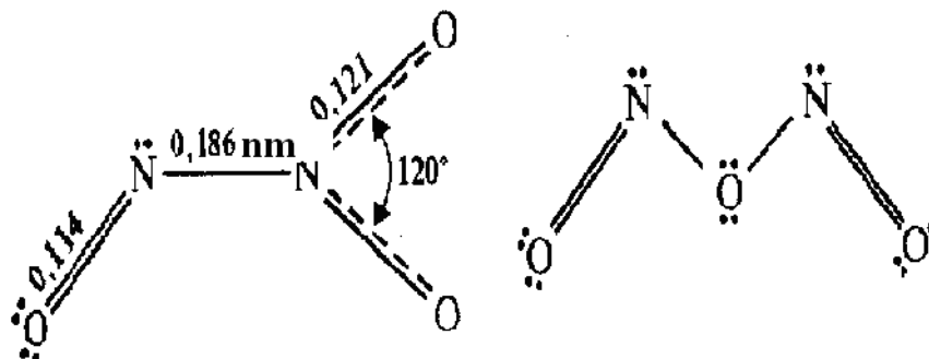
41-rasm. Azot (III) oksidi molekulasining tuzilishi.
