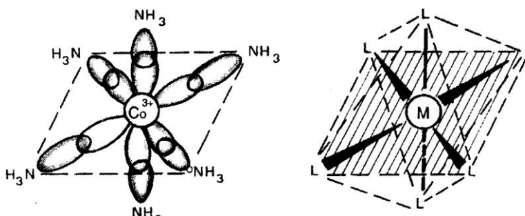
23-rasm. Koordinatsion son 6 bo'lgandagi amminlarning tuzilishi.
