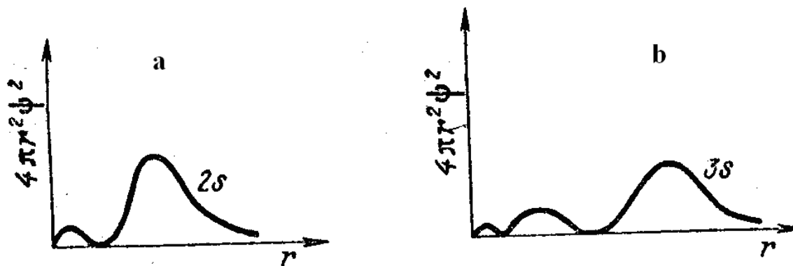
8-rasm. 2s- va 3s- elektronlarning radial taqsimlanish grafigi.
