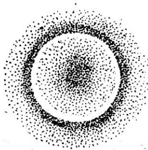
7-rasm. 2-s elektronga tegishli elektron bulut.
