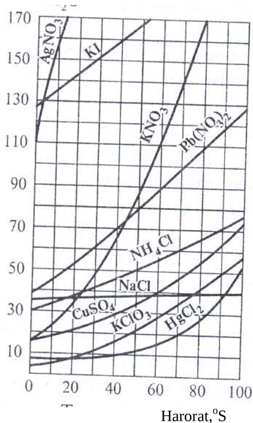
3-rasm. Eruvchanlik egri chiziqlari.
