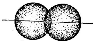
13-rasm. Vodorod molekulasida hosil bo'lishida atomlar elektron bulutlarining qoplanishi.
