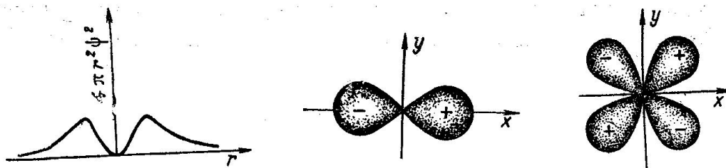
10-rasm. 2p- elektronlarning radial taqsimlanish ehtimolligini ko'rsatuvchi egri chiziqlar.
