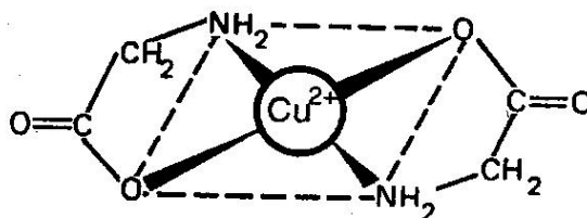
24-rasm. Dietilendiaminomis(II) va diglisinatomis(II) komplekslarining hosil bo'lish sxemasi.
