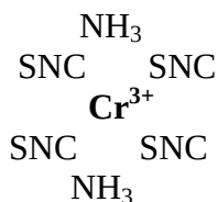
trans - izomer
