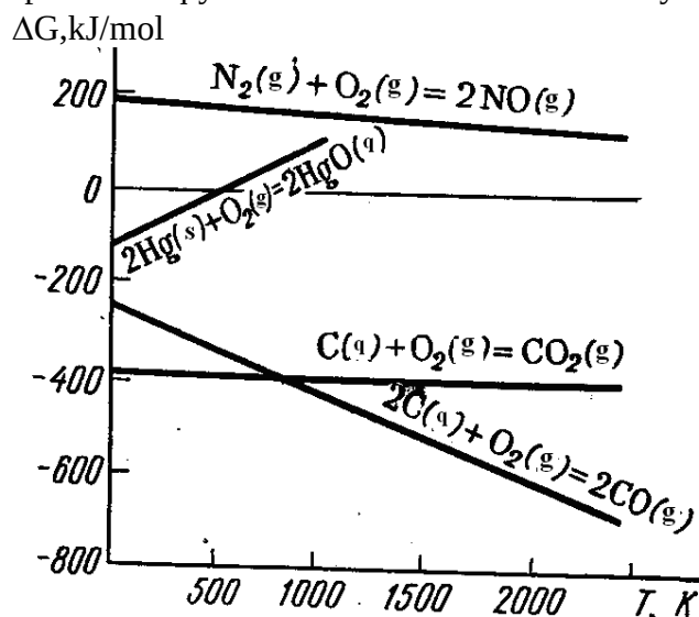
2-rasm. Kimyoviy reaksiyalarning izobar izotermik potensial qiymatining haroratga bog'liqligi.
