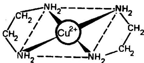
24-rasm. Dietilendiaminomis(II) va diglisinatomis(II) komplekslarining hosil bo'lish sxemasi.
