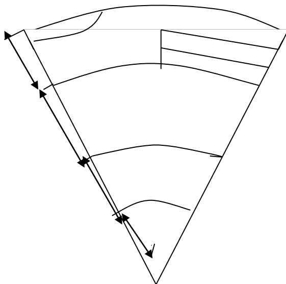
1-rasm. Yerning ichki tuzilishi sxemasi.
