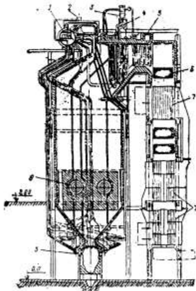
13.5-расм. ПК-19 патндаги бир барабанли қозон агрегати.
