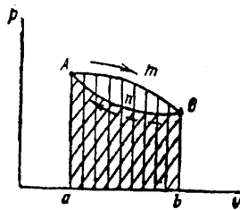
3.1-расм. Айланма процесснинг р-в диаграммада тасвирланиши
