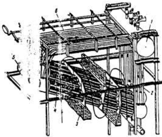
13.2-расм Шухов-типи системасидаги горизонтал сув-трубади қозон
