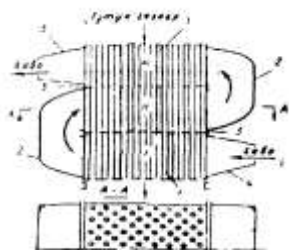
13.10-расм. Ҳитомасининг схемаси.
