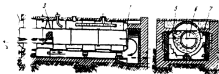
13.1-расм. Аланга трубали қозон схемаси.
