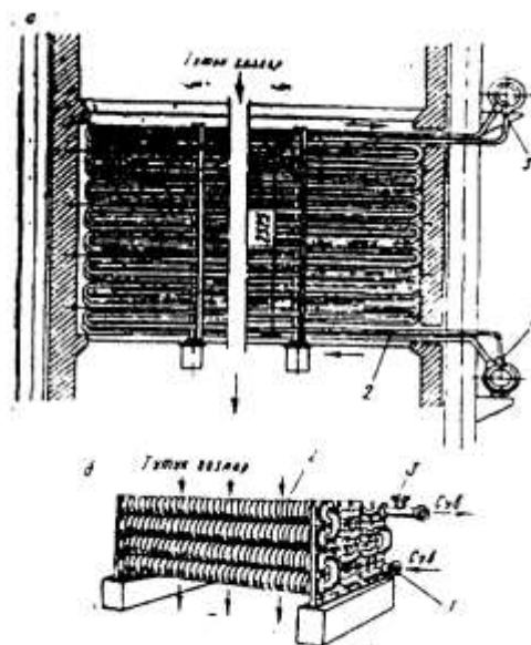
13.11-расм. Экономайзерлар
