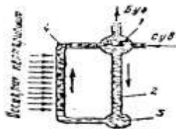
13.4-расм. Ўтхонада сувнинг табиий ҳаракати циркуляциясининг ёпиқ контурининг схемаси.
