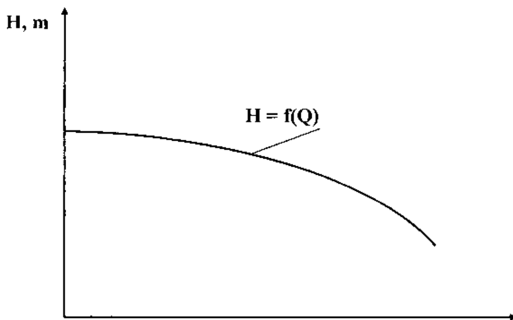
Рис. 2. Напорная характеристика насоса
