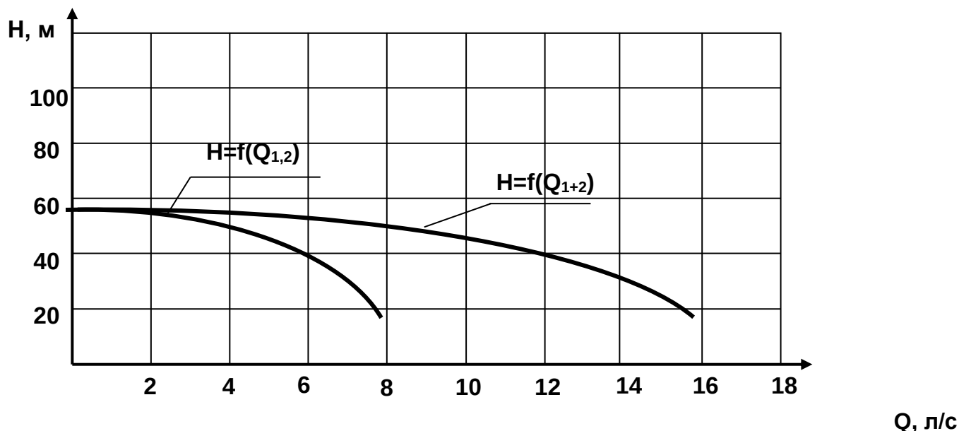
Расм 2. Кетма – кет ишлаётган иккита бир хил насосларнинг умумий напор характеристикасини қурамиз.
