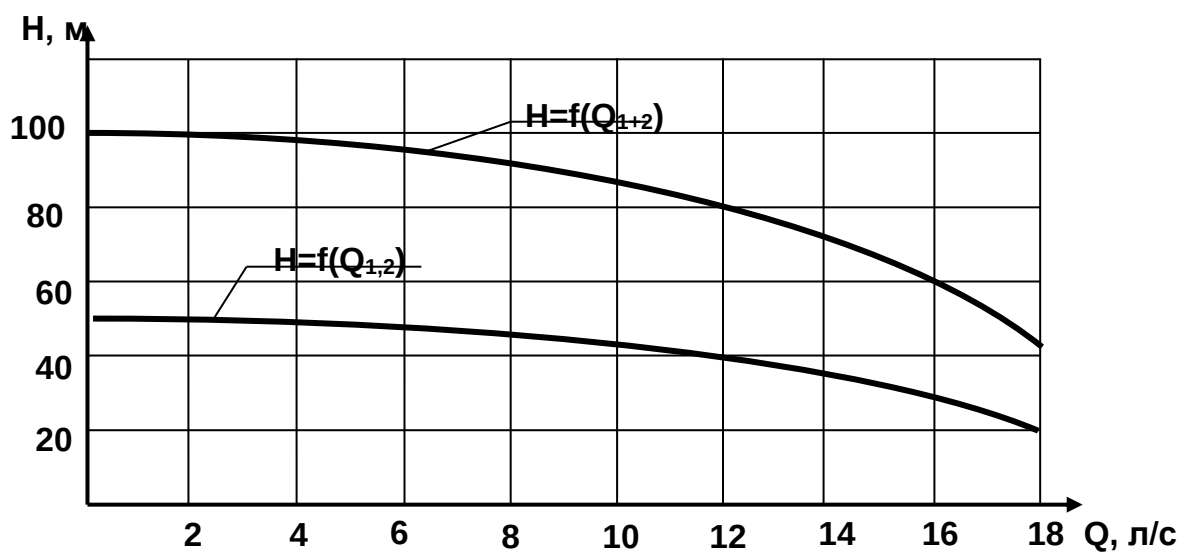
Расм 2. Кетма – кет ишлаётган иккита бир хил насосларнинг умумий напор характеристикасини курамиз.
