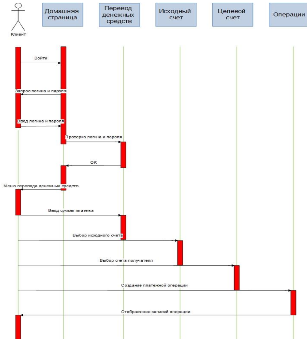
Рисунок 1.7 Последовательность действий объектов системы в меню «Перевод средств» 25
