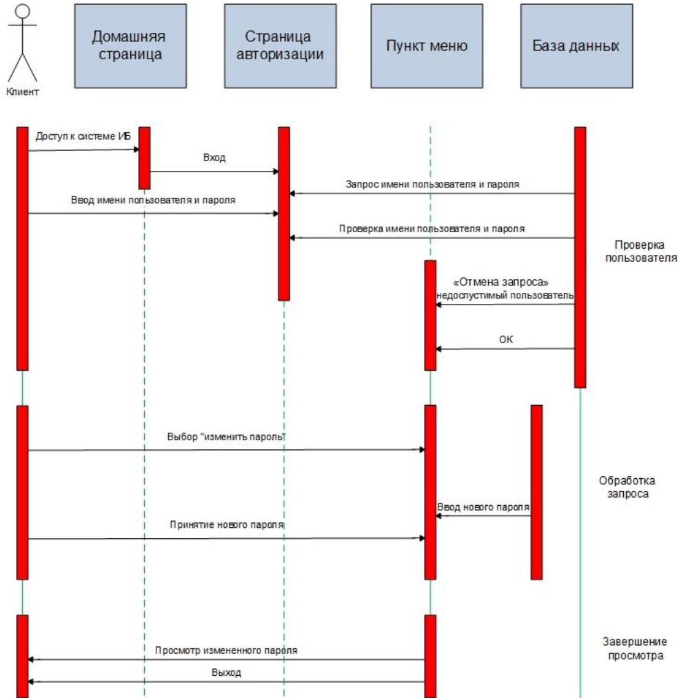
Рисунок 1.9 Последовательность действий объектов системы в меню «Настройки» 27
