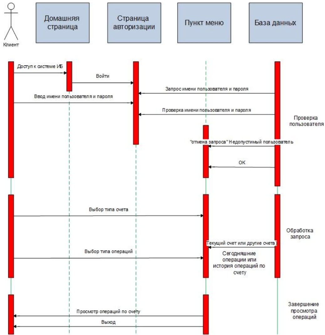
Рисунок 1.8 Последовательность действий объектов системы в меню «Просмотр операций по счету» 26
