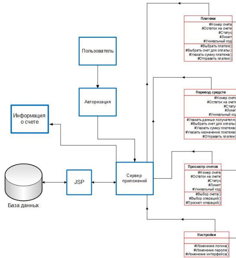
Рисунок 1.10 Физическая модель системы интернет-банкинга 28
