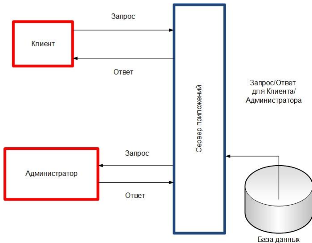
Рисунок 1.11 Архитектура приложений интернет-банкинга 29
