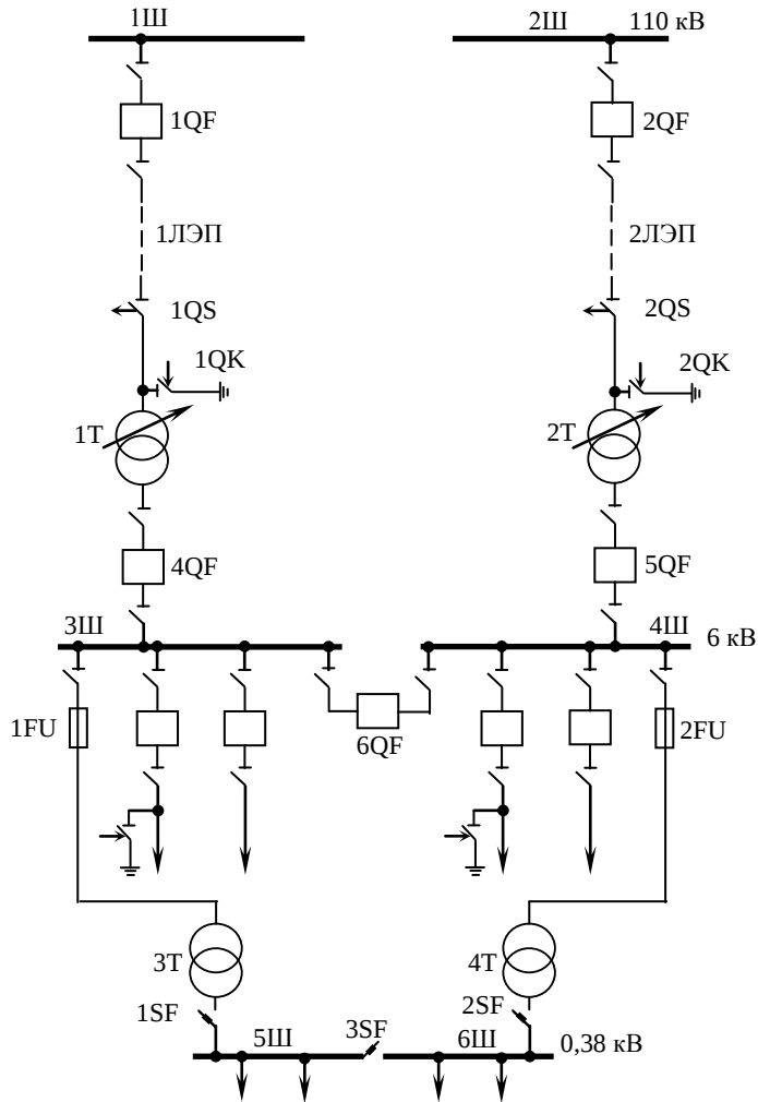
Рис.2.8. Схема электроснабжения с двумя питающими линиями, отделителями и короткозамыкателями в конце питающих ЛЭП
