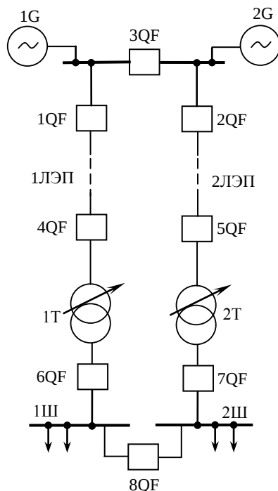
Рис.2.6. Схема электроснабжения с двумя питающими линиями и выключателями в начале и конце каждой из них
