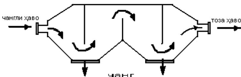
3-расм. Тўсиқли чанг чўктириш камераси
