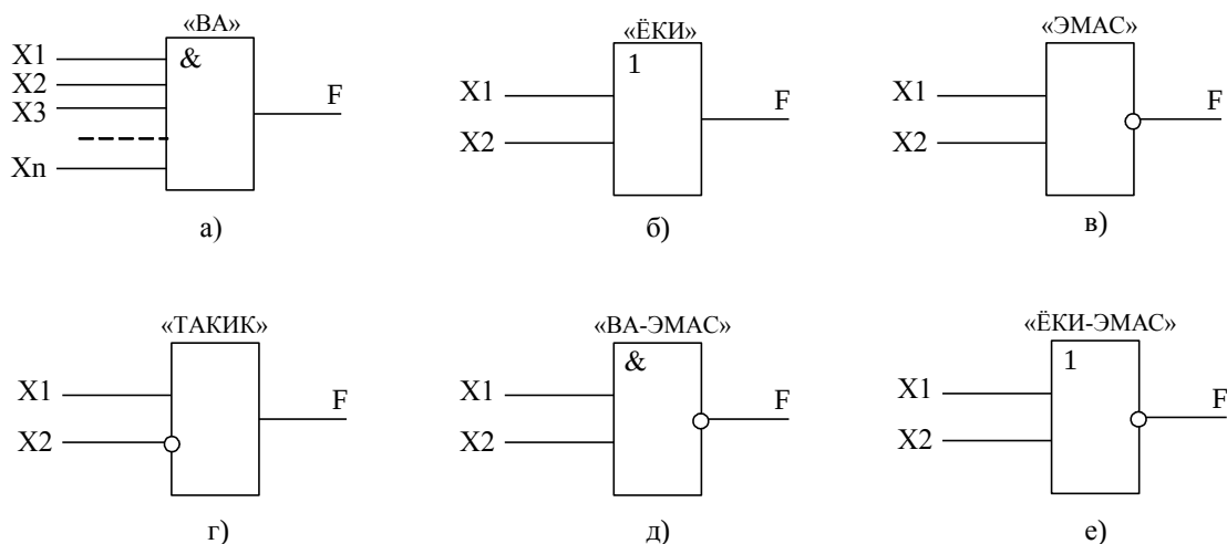
1-расм. Мантиқий элементларнинг шартли белгиси.
