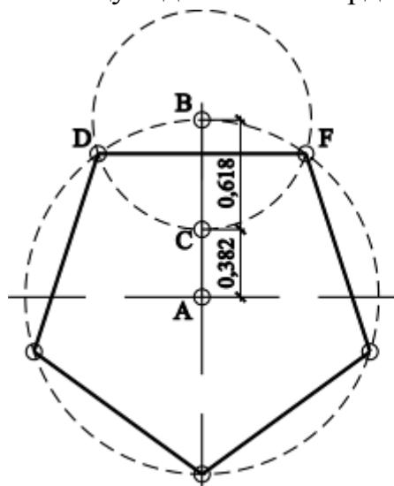
1-расм. Айланани тенг 5 томонли бурчакга бўлиш
