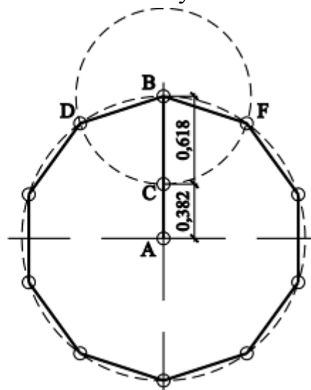
2-расм. Айланани тенг 10 томонли бурчакга бўлиш
