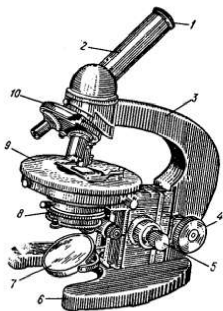
1-рasm. Микроскопининг (МБИ — 1) тузиллиши:
