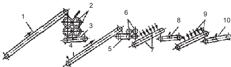
3.7-rasm. AKV mashinasining texnologik chizmasi:
