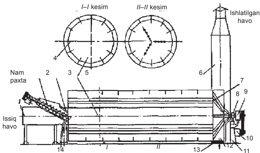
1.7-rasm. 2SB—10 rusumli quritgich chizmasi:
