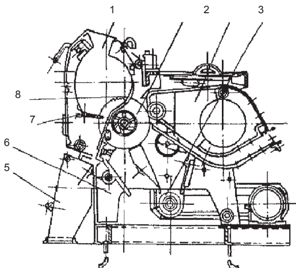
1.11-rasm. 3XDDM arrali jin:
