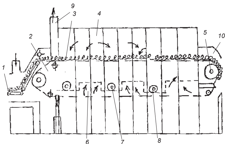
5.11-rasm. LX – 3 quritish moslamasining texnologik chizmasi:
