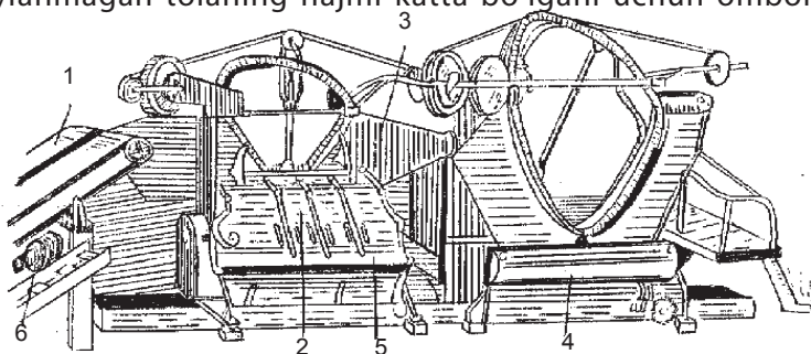
3.8-rasm. TMM—200 K rusumli ezish-titish mashinasining umumiy ko'rinishi chizmasi:
