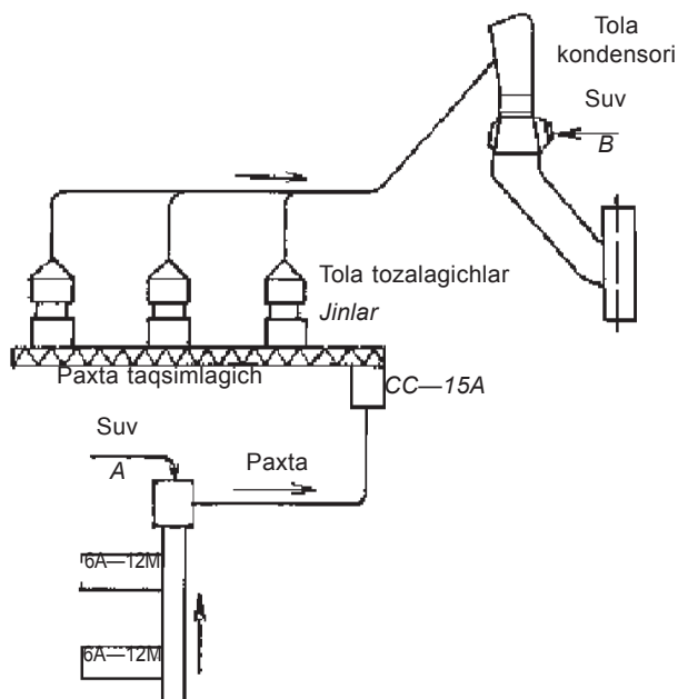
1.22-rasm. O'rta tolali paxta va tolani namlash qurilmasining chizmasi:
