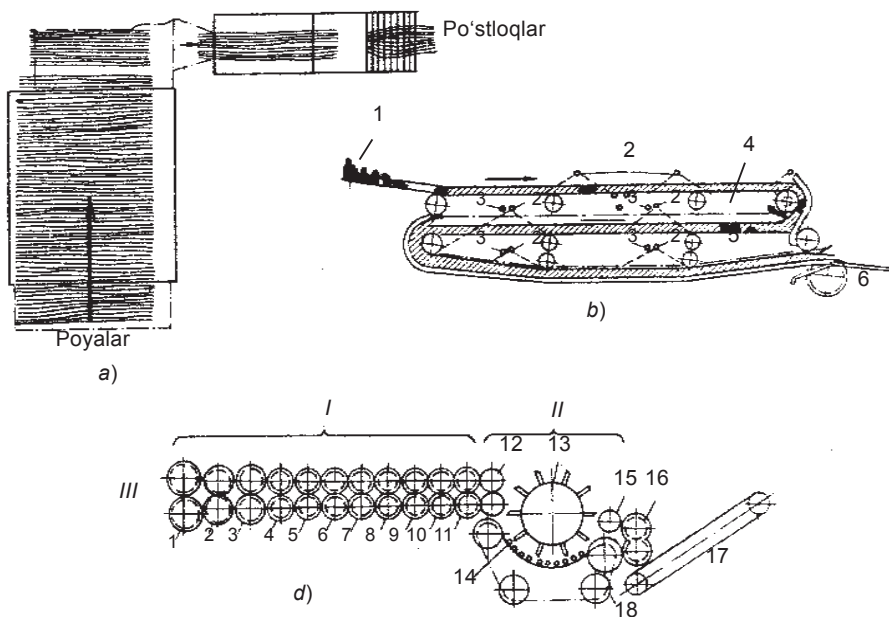
3.3-rasm. MT—100—K agregatining va namlash moslamasining chizmasi: a — MT—100—K agregatining texnologik chizmasi; b — namlash moslamasining chizmasi; 1 — poya uchun stol; 2 — yuqorigi namlash tizimi (teshikli quvurlar); 3 — pastki namlash tizimi; 4 — qoziqsiz zanjir; 5 — qoziqli zanjir; 6 — o'tkazish stoli; d — MT—100—K agregati ezish-titish qismining chizmasi.
