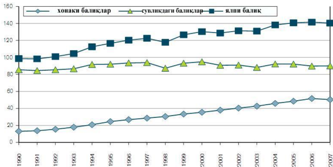
8-расм. Жаҳонда балиқ етиштириш 1990-2007 (млн.т)
