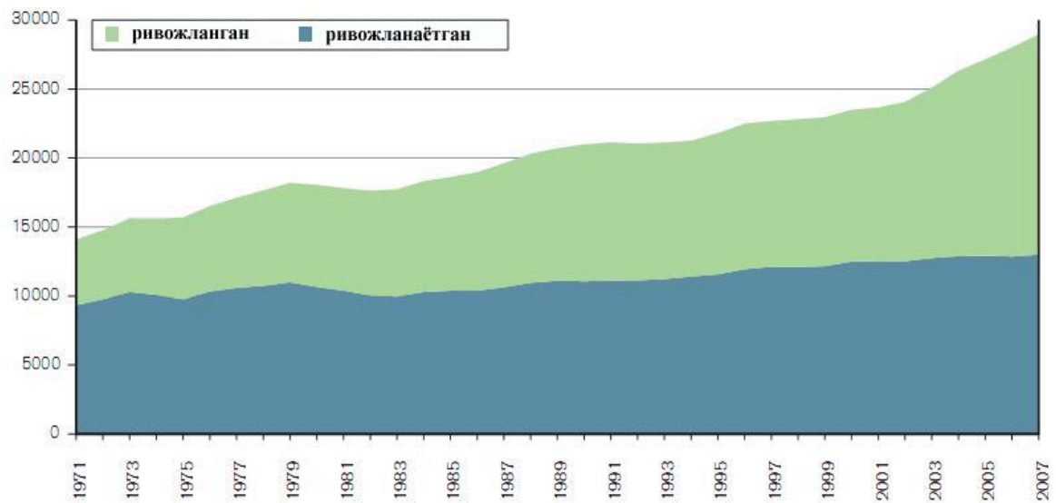
9-расм. Жаҳонда CO 2 ни атмосферага чиқарилиши
