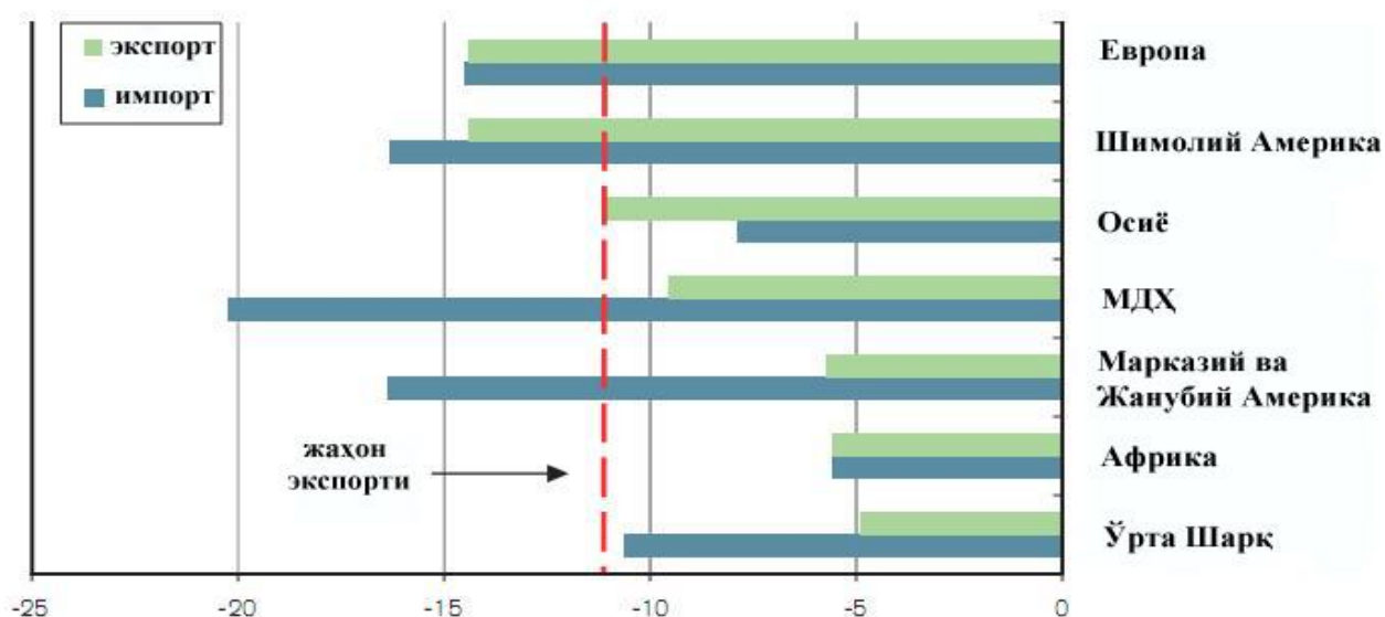
2-расм. Минтақалар бўйича товарлар савдосининг ўзгариши 5 ( 2009й. % ҳисобида)
