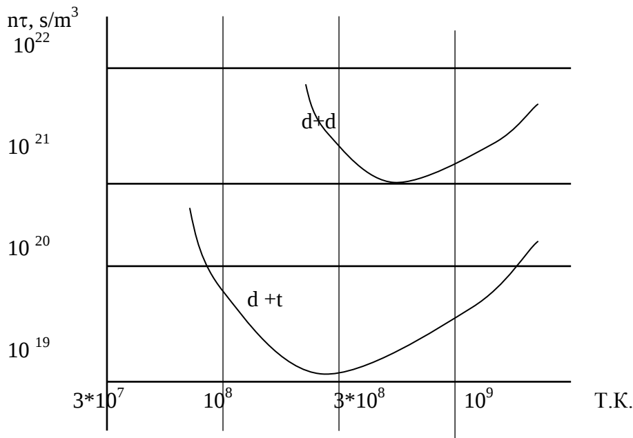
9.1-rasm. Deyteriy tritiy, deyteriy-deyteriy reaksiyalari uchun plazmani ushlab turish parametrining temperaturasi bog'liqligi.
