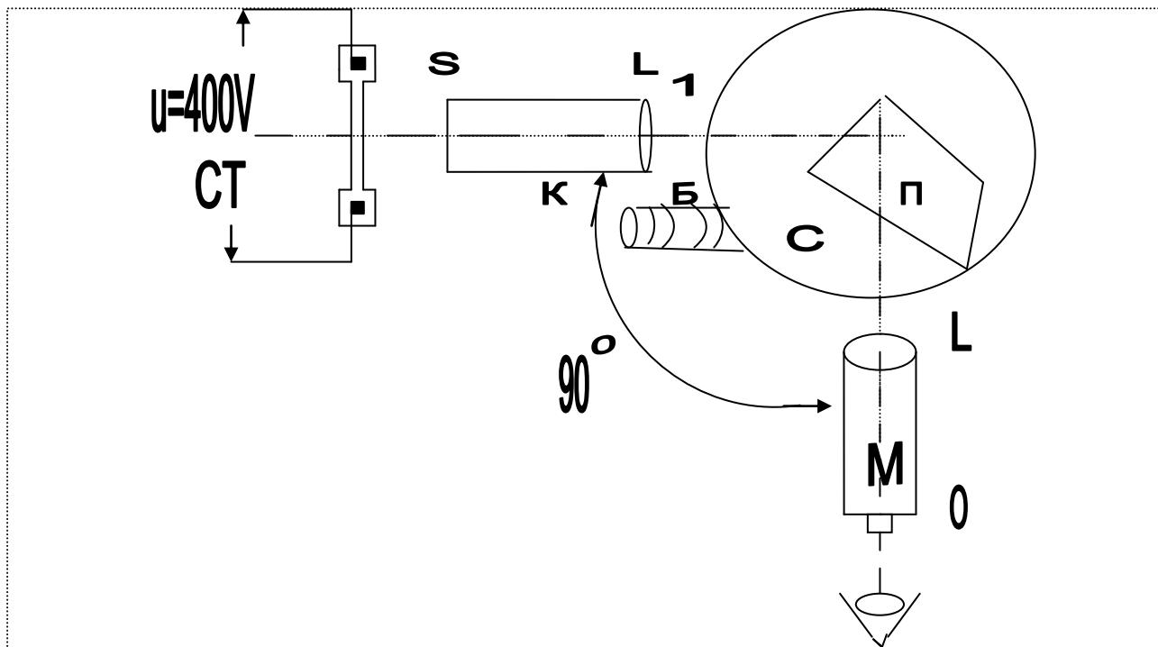
4-rasm. Monoxromatorning printsipl sxemasi. P-prizma, K-kollimator, O-okulyar, B-baraban, ST-spektral trubka.
