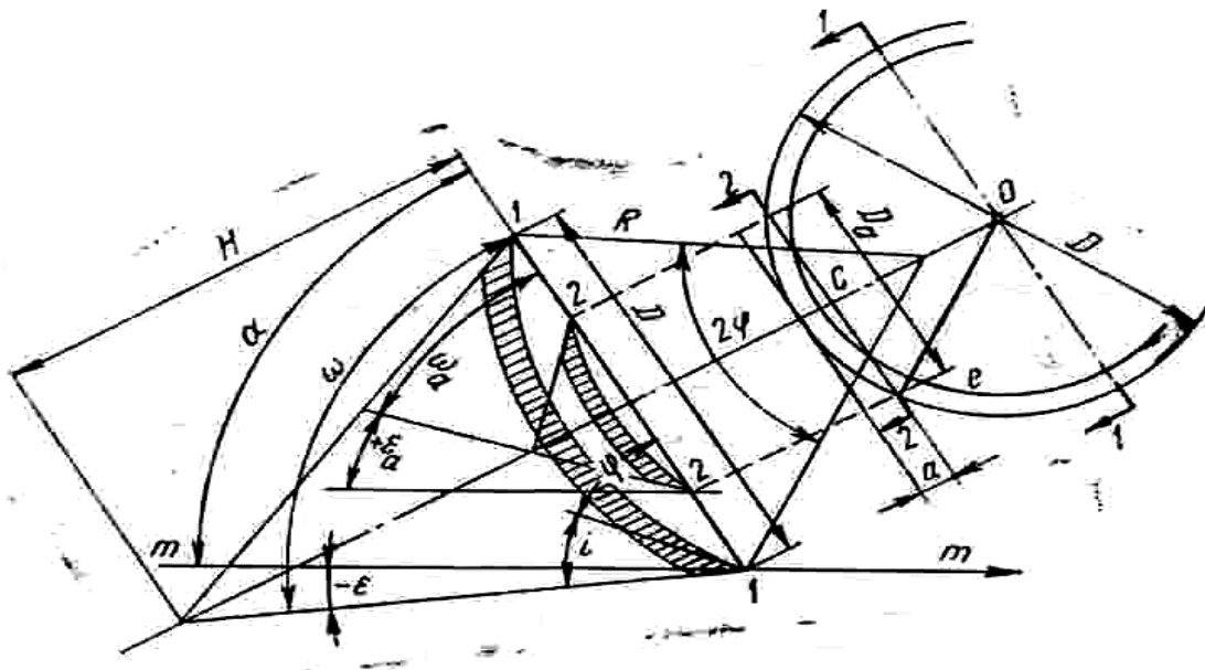
28-расм. Сферик дискнинг геометрик тавсифинини аниқлаш схемаси.
