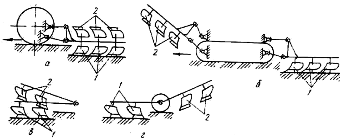
11-расм. Текис ҳайдаш плугларининг схемаси. А-айланма; б-мокисимон ҳаракатланувчи; в-клавишли; г-балансирсимон; 1-ўнг томонга ағдарувчи корпуслар; 2-чап томонга ағдарувчи корпуслар.
