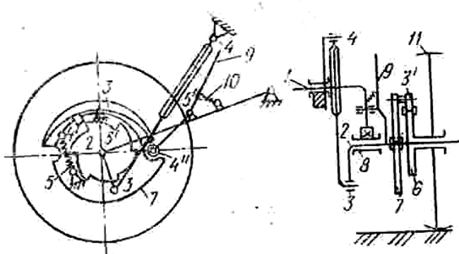
25-расм. Очик храповикли автомат. 1-2-3-4-ташқи кўтариш механизми; 2-3-4-5-ички механизм; 2-3-4-5-ишга солиш механизми; 1-чап ўқ тирсаги; 2-кривошип вал; 3-4-телескопик шатун; 5-пружина; 6-храповик; 7-диск; 8-подшипник; 9-ишга солиш ричаги; 10- пружина; 11-дала ғилидираги.
