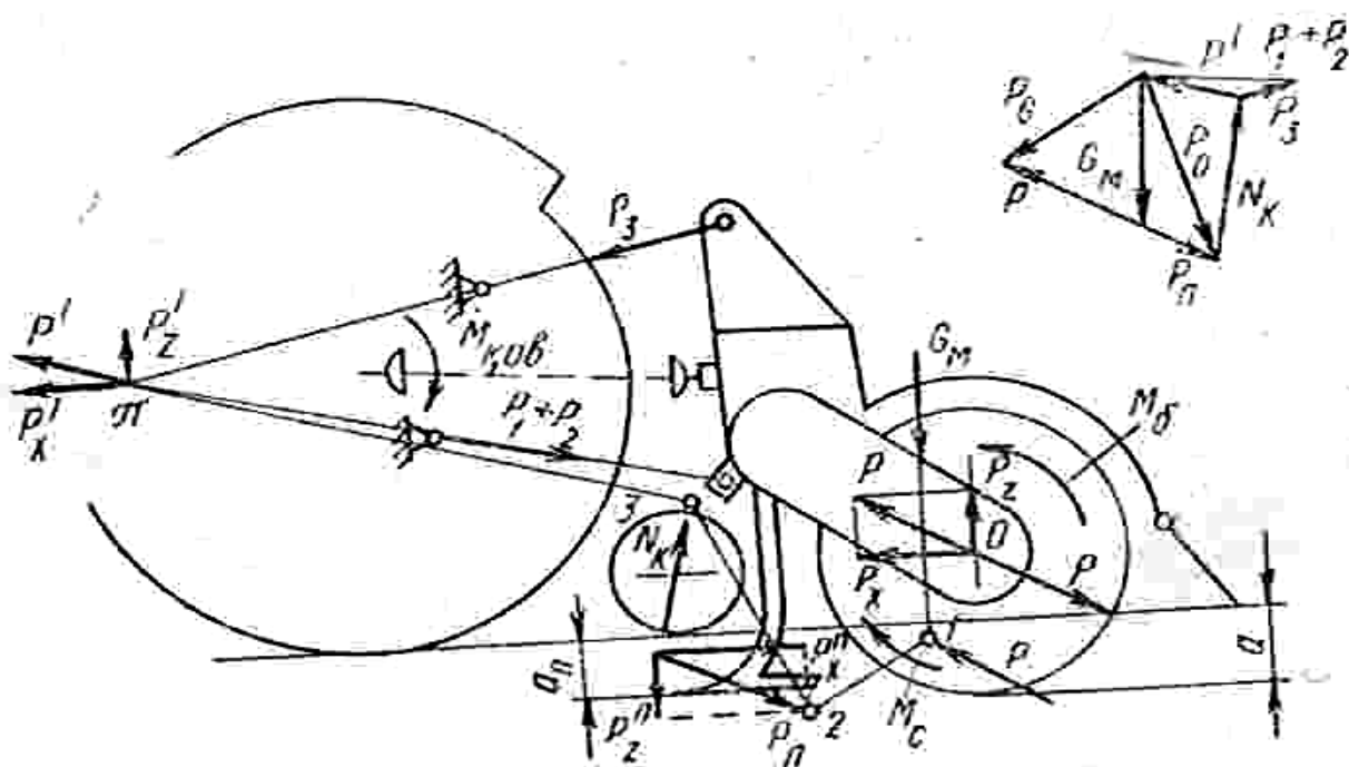
39-рasm. Ротацион фреза-култиваторга таъсир этувчи кучлар ва мувозанатлик шарти.
