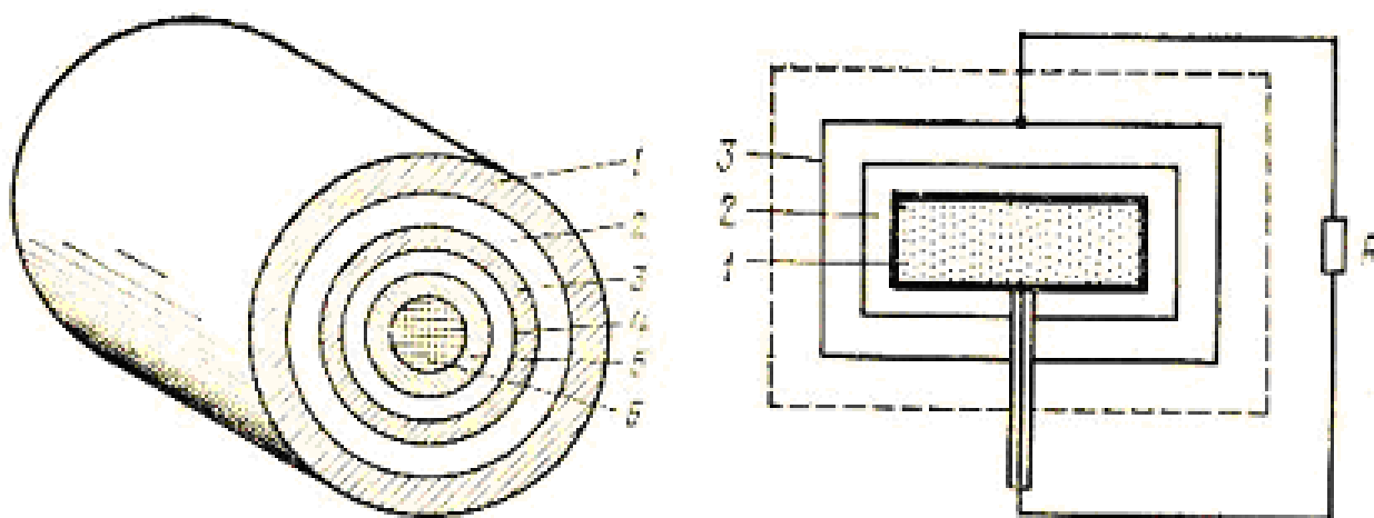
14.7-Rasm. Yadro energiyasini to'g'ridan to'g'ri elektr energiyaga o'zgartirish qurilmasining sxemasi.
