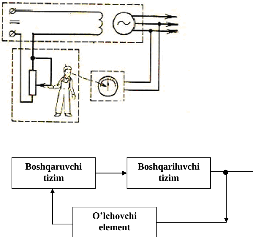
17.15. rasm. Inson tomonidan amalga oshiriladigan teskari aloqali sodda yopiq boshqarish tizimi.
