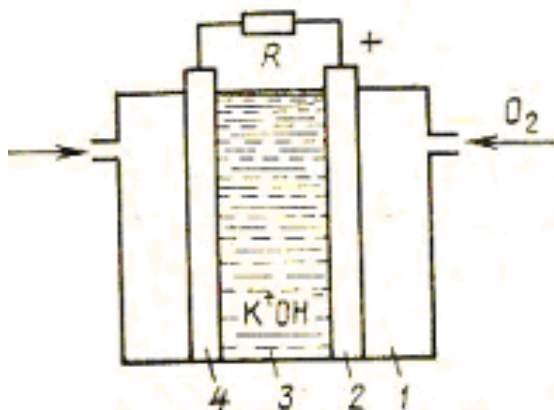
14.10-Rasm. Vodorod-kislorodli yoqilg'i elementi.
