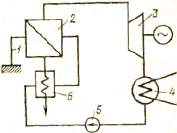
15.1-rasm. Vulqonli rayonlardagi geotermal elektr stantsiya sxemasi.
