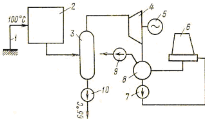
15.2-rasm. Vulqon sodir bo'lmaydigan rayonlardagi geotermal elektr stantsiya.
