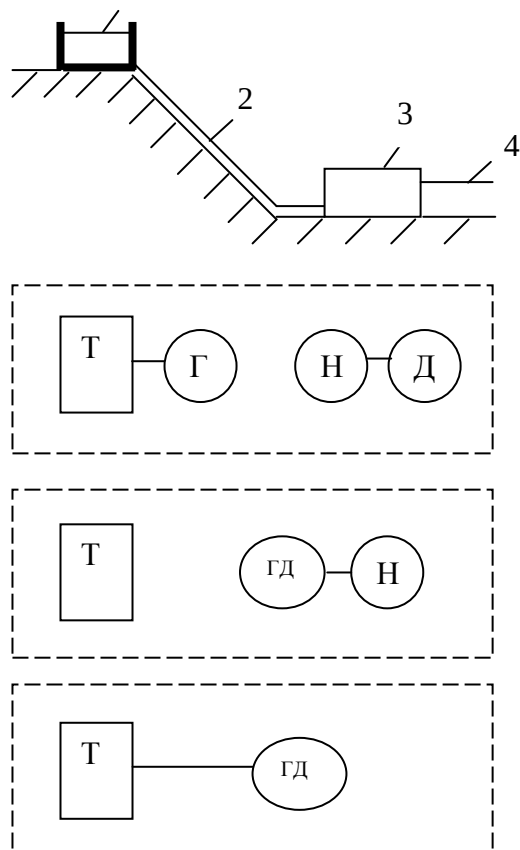
11.1- rasm. Hidroakkumulyatsiya stantsiyaning ishlash sxemasi.
