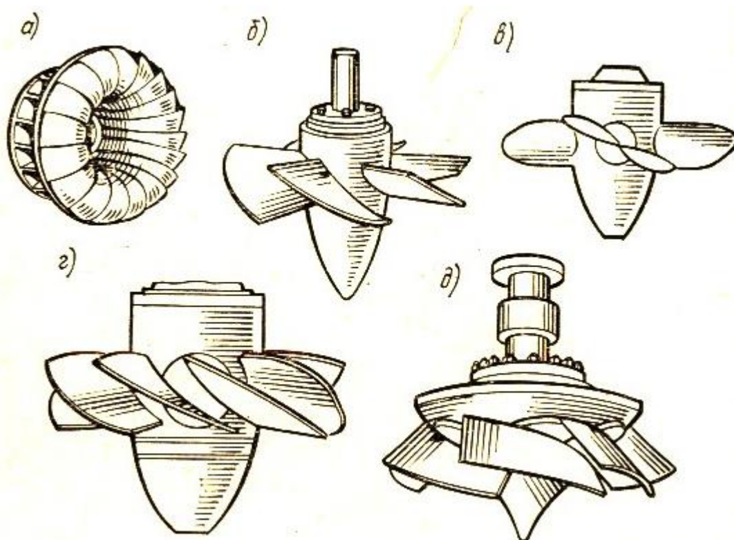
10.3-rasm. Reaktiv turbinalarning ishchi g`ildiraklarini o`mumiy ko`rinishi. a-radial o`qli, b-propellerli, v-buraluvchi parrakli, g-ikki patli, d-diagonalli.
