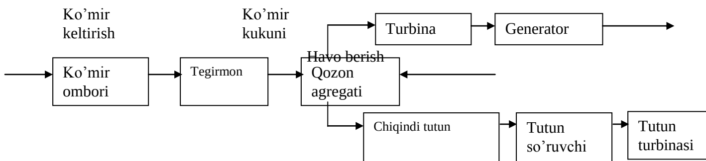
6.2-rasm. Issiqlik olish va uni elektr energiyaga aylantirishni IES da texnologik jarayoni sxemasi.
