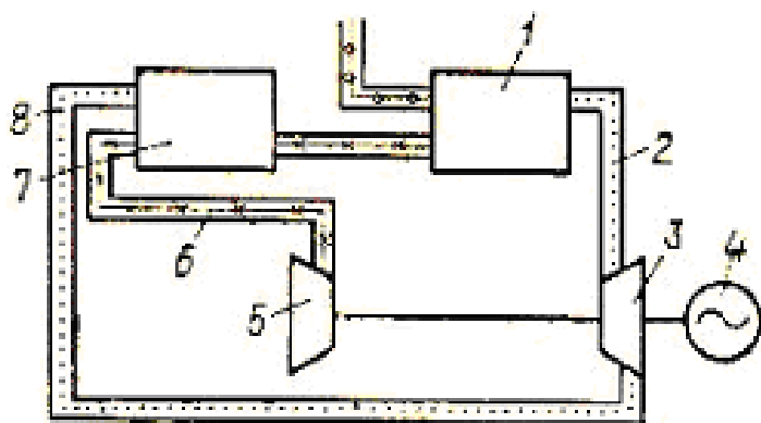
8.1-rasm. Gazturbina qurilmasining printsipl sxemi.
