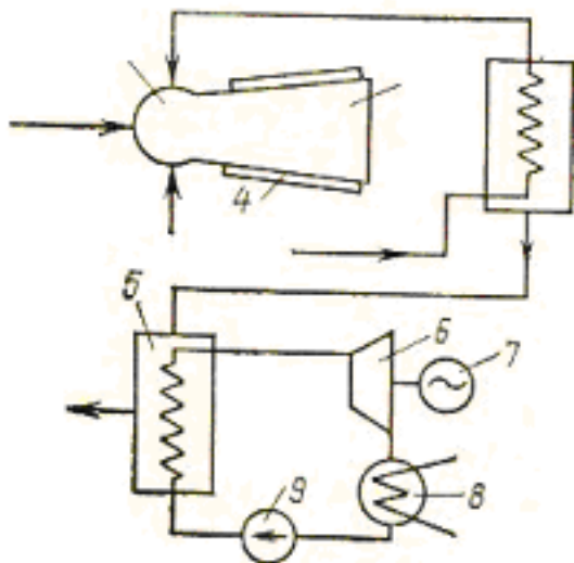
14.2-rasm.Bug'-kuch qurilmasi bilan MGD generatorining printsiipial sxemasi.
