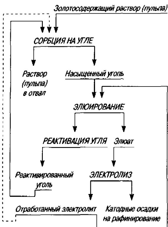
Рисунок 1- Схема угольно-сорбционного процесса
