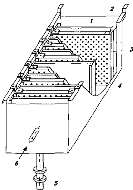
Рис. 6. Ванна конструкции «Минтек»
