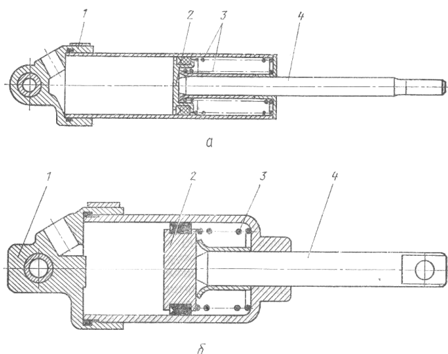
1.21-расм. Пневматик цилиндрлар. а-тормоз секинлаткич юритмаси, б- ёнилғи насоси юритмаси ричаги. 1-асос, 2-поршен, 3-пружина, 4-шток.
