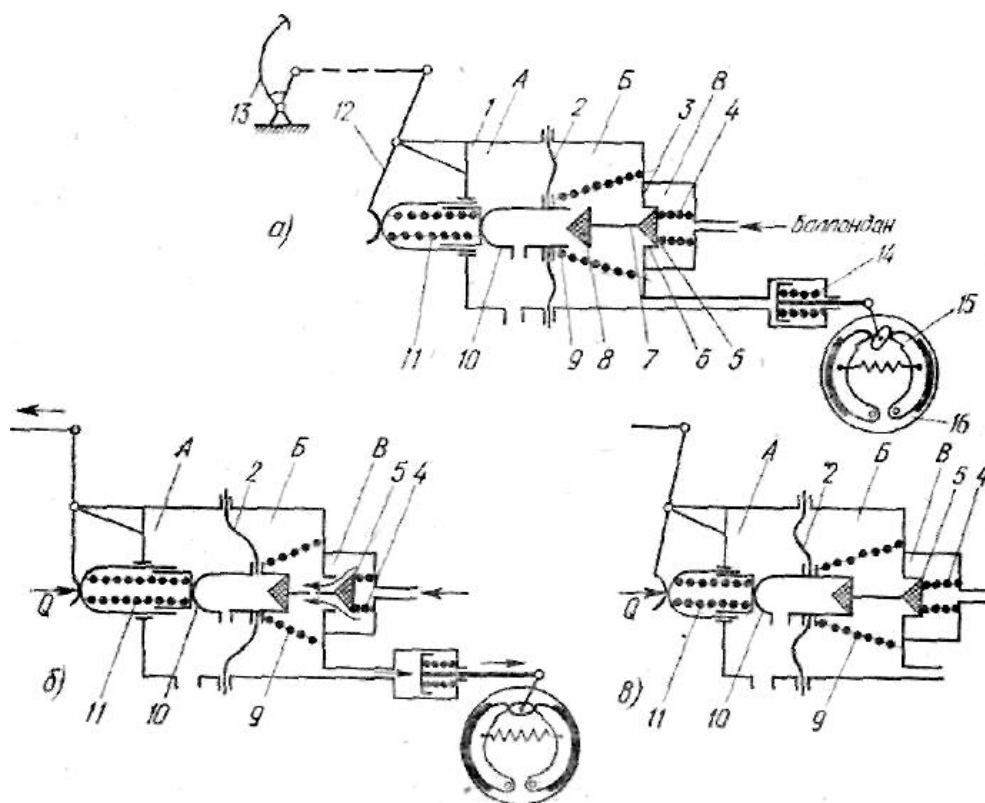
1.15-расм. Тўғри ҳаракатланувчи диафрагмали мослагич механизмининг схемаси:
