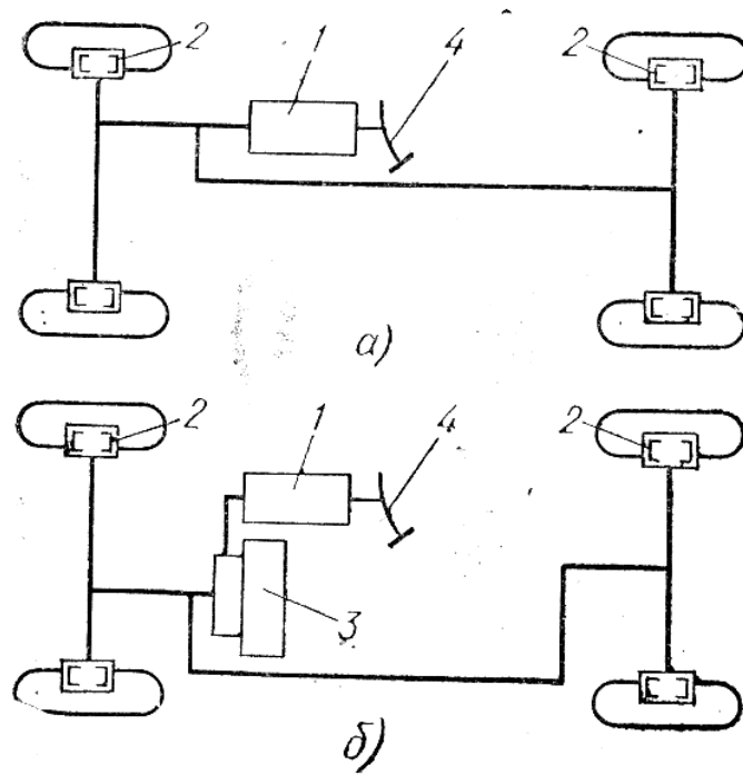
1.12-расм. Бир контурли гидравлик тормоз юритмасининг схемаси а-гидростатик юритма, б-гидроваккумли юритма.
