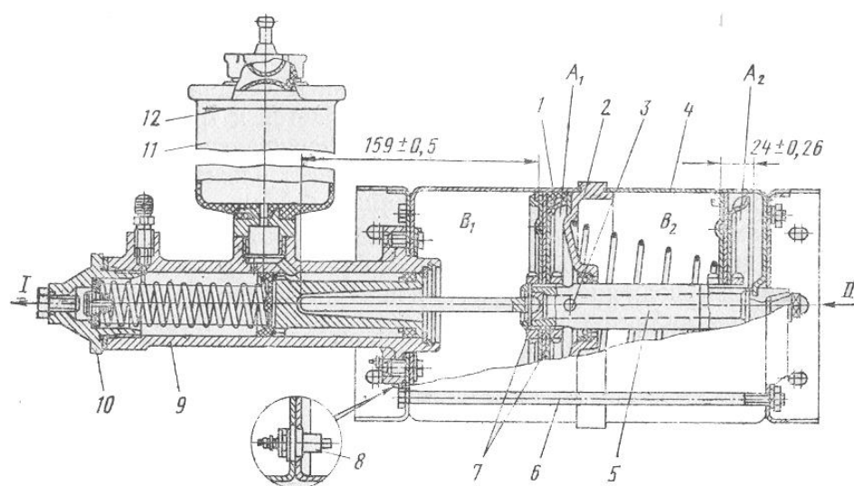
1.19-расм. Ҳаво кучайтиргичида бош гидравлик тормоз цилиндри 1-олдинги пневматик цилиндр, 2-резина қўйгич, 3-радиал тешик, 4-орқа
