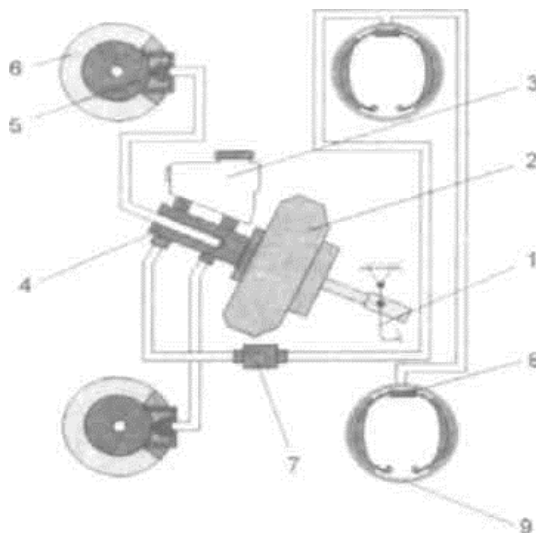
1.2-расм. «Тико» автомобилининг ишчи тормоз тизими.
