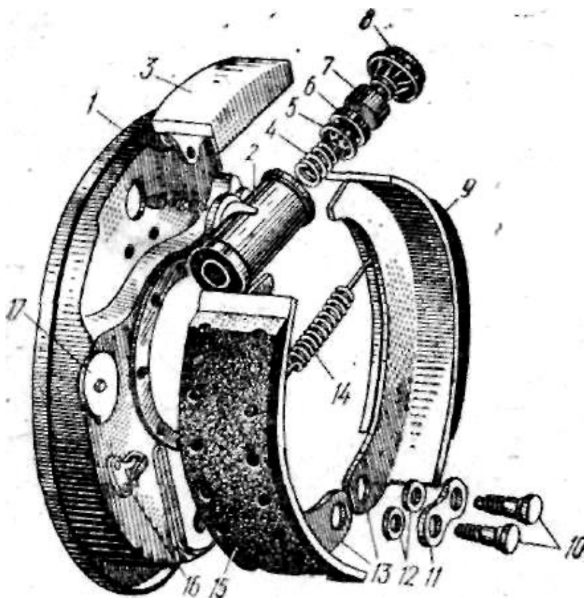
1.11-расм. ГАЗ-53А автомобилнинг кетинги ғилдирак тормози
