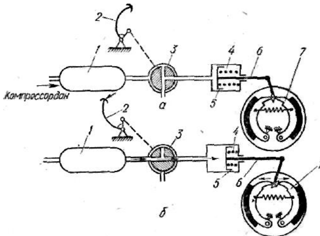
1.14- расм. Пневматик юритмали тормоз системасининг соддалашган схемаси: а) тормозланмаган ҳолати, б) тормозланган ҳолати.
