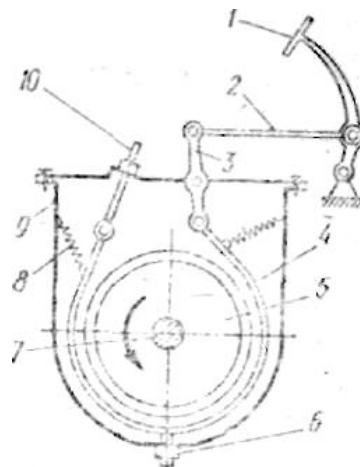
1.7-расм. Лентали барабан типигаги тормоз схемаси
