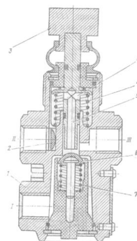
1.22-расм. Пневматик бошқариш крани.
