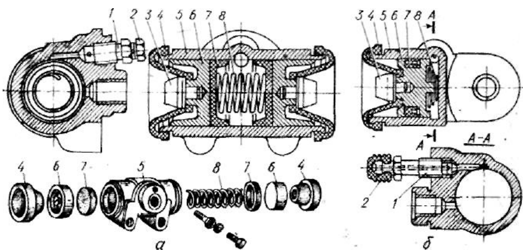
1.9- расм. Ғилдирак тормоз цилиндrlари:
