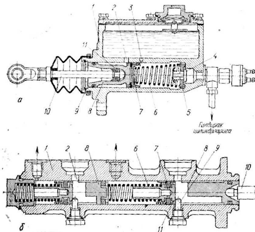
1.8- расм. Асосий тормоз цилиндрлари:
