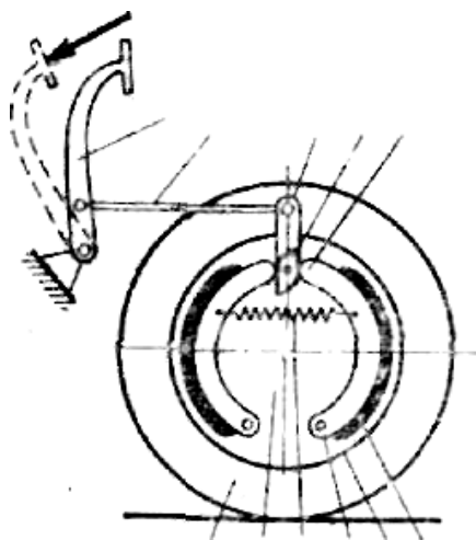
1.6-расм. Колодка барабан типигаги ғилдирак тормози
