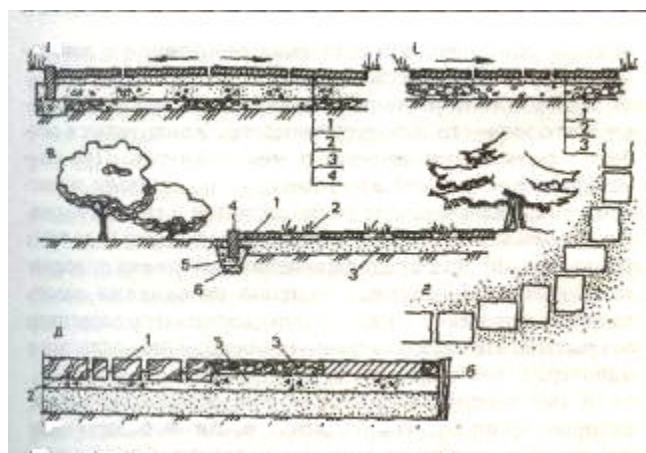
Рис. 19.. Конструкции парковых аллей и дорожек: а - транзитная дорога (1 - плиты бетонные, 6 см; 2 - выравнивающий слой цементного раствора, 3 см; 3 - бетон, 10 см; 4 - щебень или шлак, 5-10 см); б - садовая пешеходная аллея (! - плиты бетонные, 4~6 см; 2 - выравнивающий слой, 2~3 см; 3 - щебень, 3 см); в - дорожка на песчаном основании I! ~ обломы плит; 2 - растительный грунт; 3 - песок, III см); г - укладка плит на углах и поворотах; д - дорога с комбинированным покрытием (I - деревянные торцы, 10 см; 2 - цемент, 5 см; 3 - галька на цементном растворе; 4 - песок, 5 см; 5 - борт из деревянных чурок)
