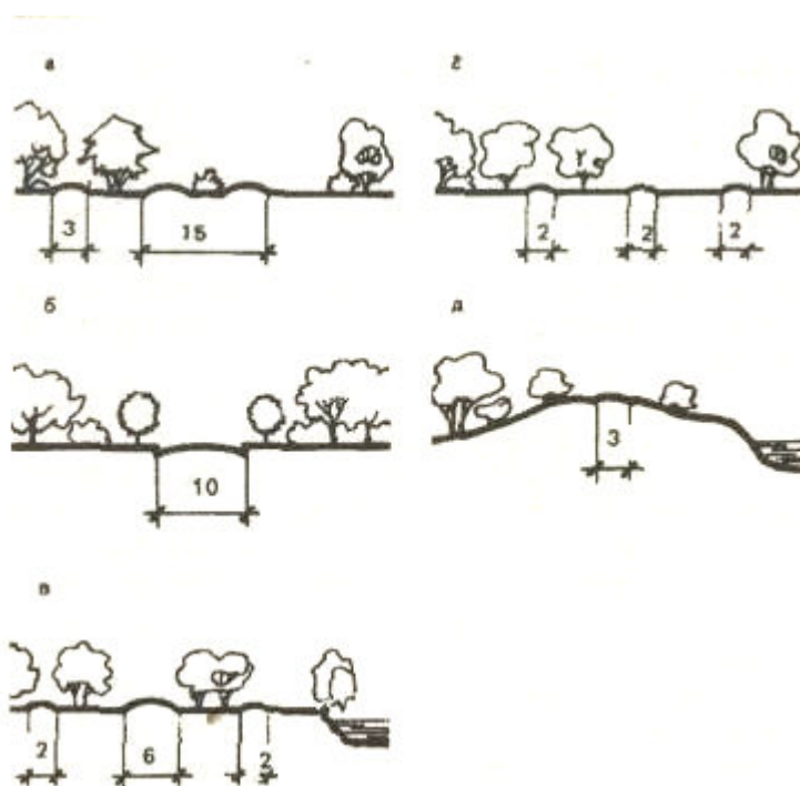
Рис.17. Поперечные профили парковых аллей и дорожек: а - аллея, разделенная кустарником; б - широкая регулярная аллея; в - аллея с сопутствующими дорожками; г - дорожек; д - дорожка вдоль водоема
