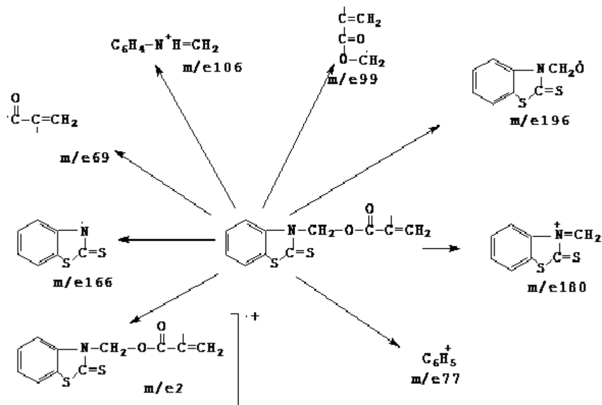
6- Rasm. a) Akril kislova benzthiazoltionilmetilen efiri Mass-spektri b) AKBTME mass-spektri sxemasida hosil bo`lgan fragmentlar tavsifi
