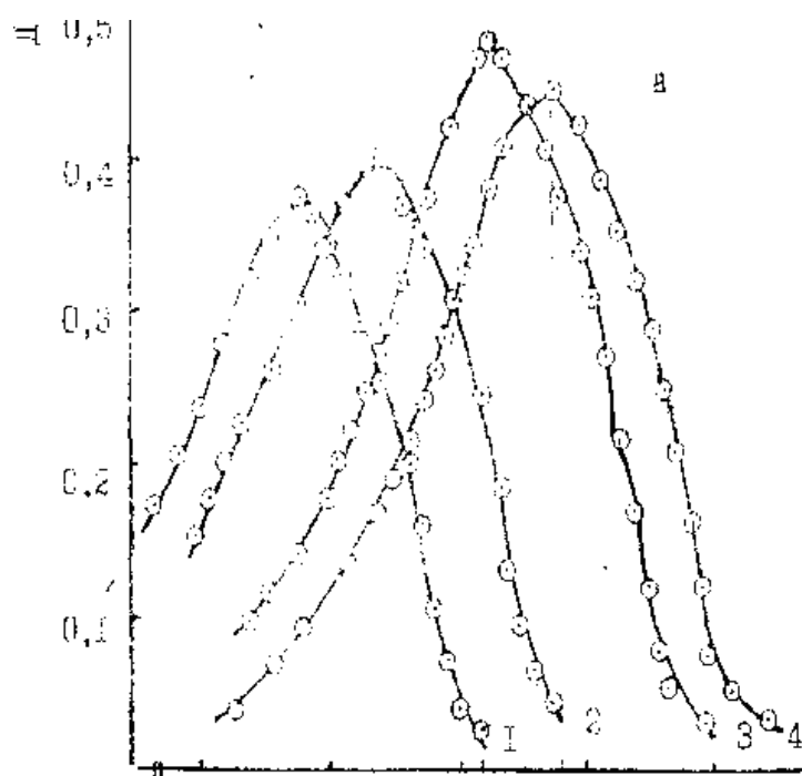
1-rasm. Akril kislota benzoksazonilmetilen efiri (a), akril kislota benzoksazoltionilmetilen efiri (b), akril kislota benziazolonilmetilen efir (v) va akril kislota benziazoltionilmetilen efir (g) lari UB- spektrlari
