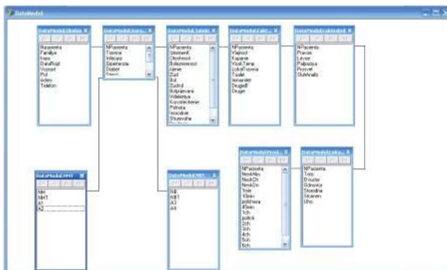
Рис. 4.5. Структура базы данных
