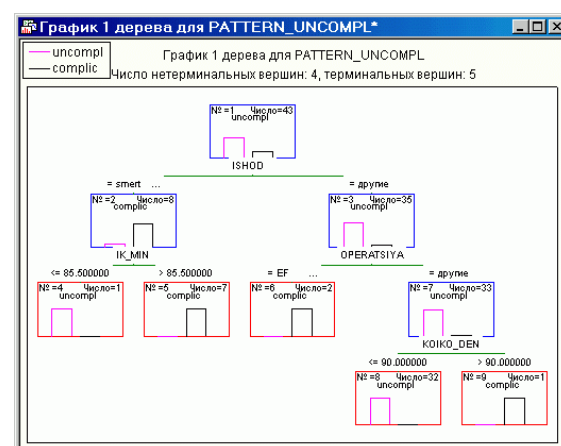
Рис.2.8. Дерево классификации
