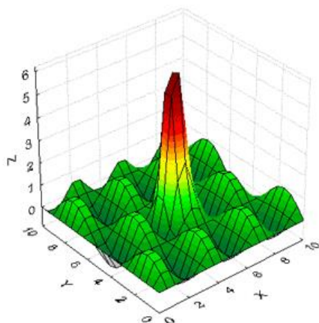
Рис.2.13. График функции
