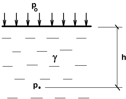
Рис. 1. Схема к основному уравнению гидростатики
