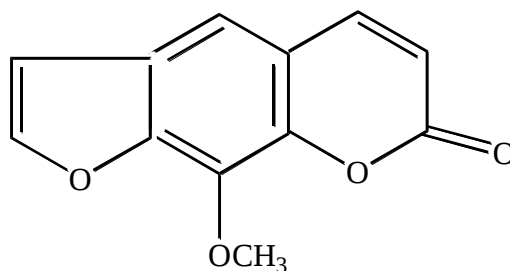
Ксантатоксин
