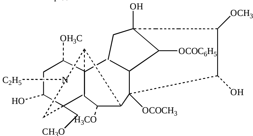
Аконитин
