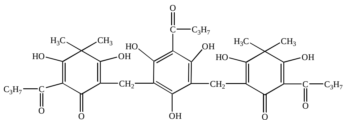
Филикс кислотаси
