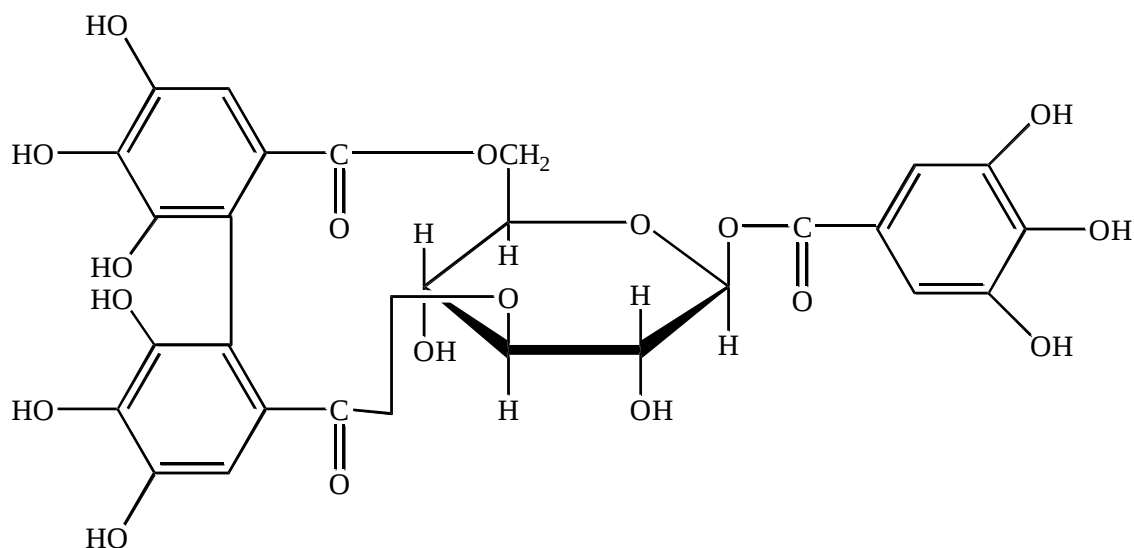
Корилагин
