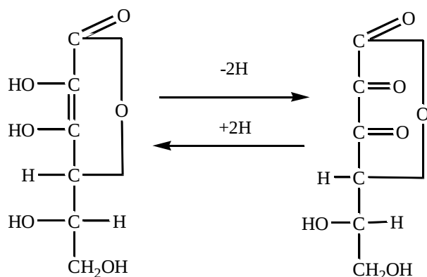
α-Аскорбин кислота
