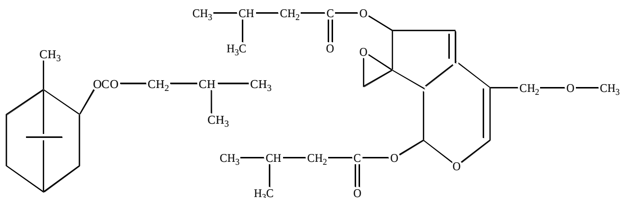
Борнилизовалерионат
