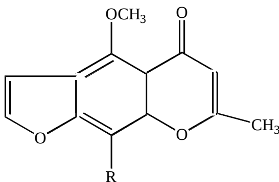
Келлин R-OCH_3
