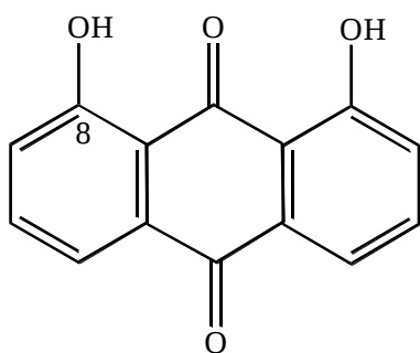
Хриаацин
