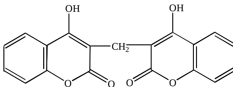
Дикумарол
