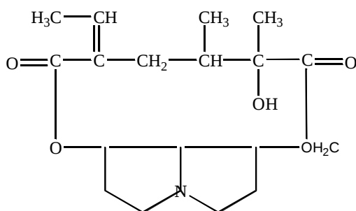
Платифиллин
