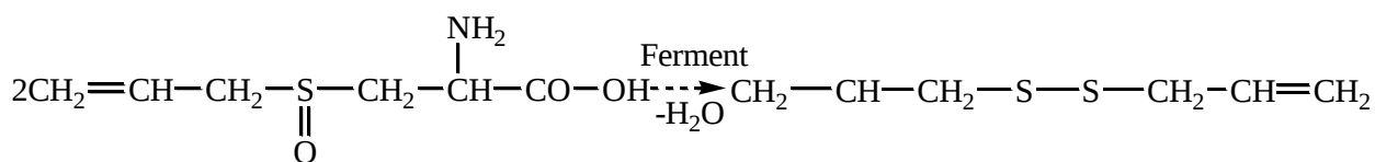
Аллиин
