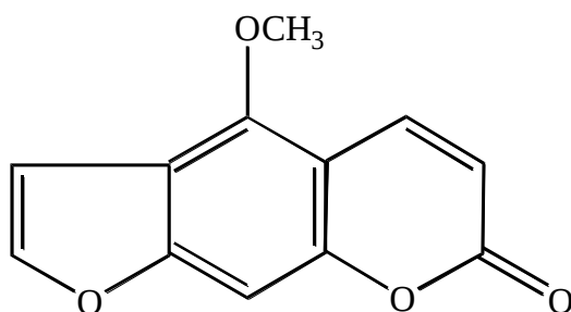
Бергаптен
