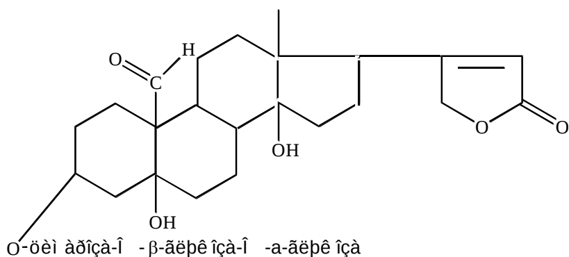
К- строфантозид
