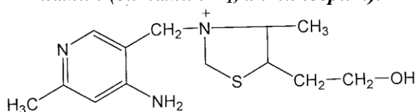
Тиамин
