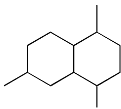
Каламен
