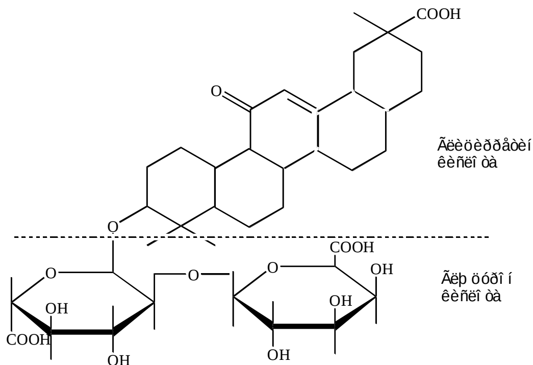
Глицерризин кислота
