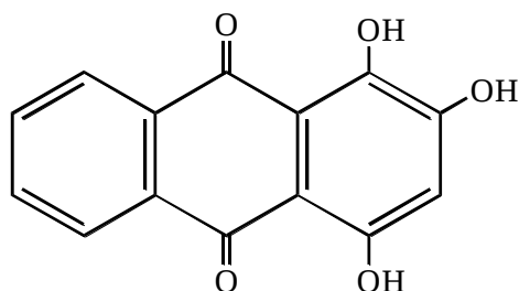
Пурпурин
