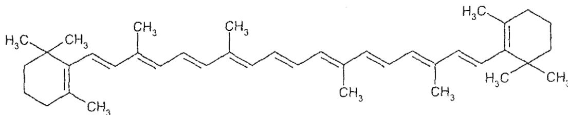
β-каротин
