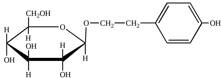
Салидрозид (родиолозид)
