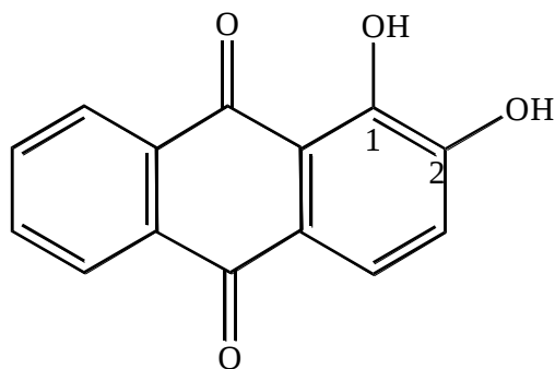
Алиаарин
