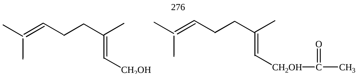
Гераниол
