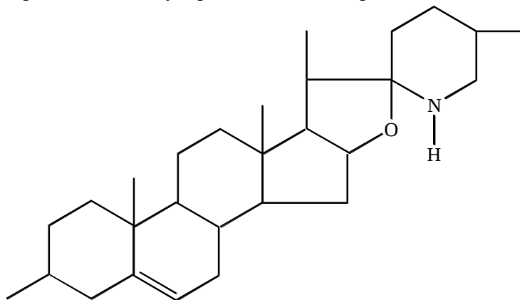
Соласодин
