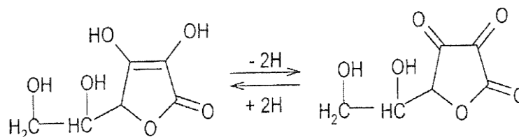
L-аскорбин кислота
