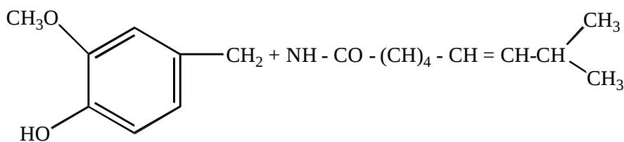
Капсаицин
