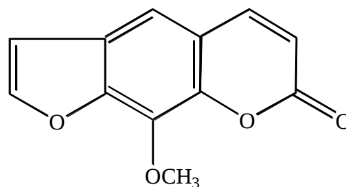
Ксантотоксин
