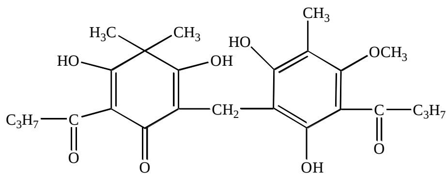
Флаваспидин
