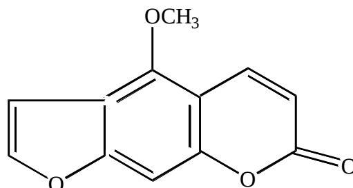
Бергаптен
