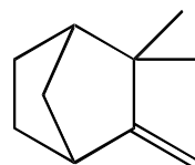
Камфен
