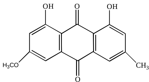
Фиоцион (реохриаин)
