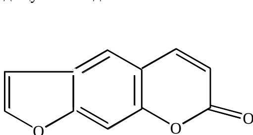
Псорален
