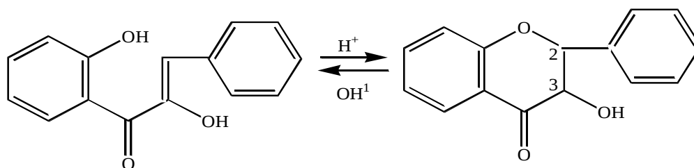
Флавонон
