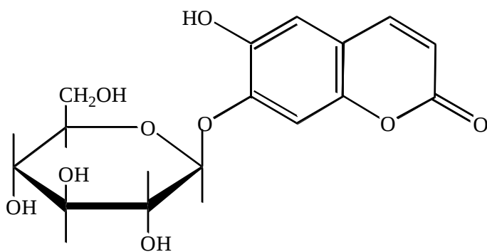
Цикорин
