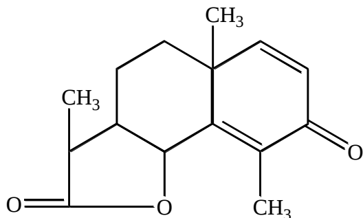
Сантонин
