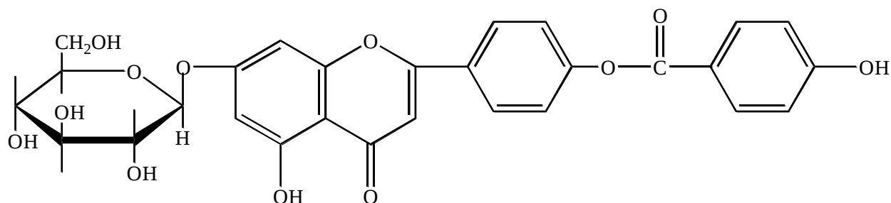
Квинквелозид
