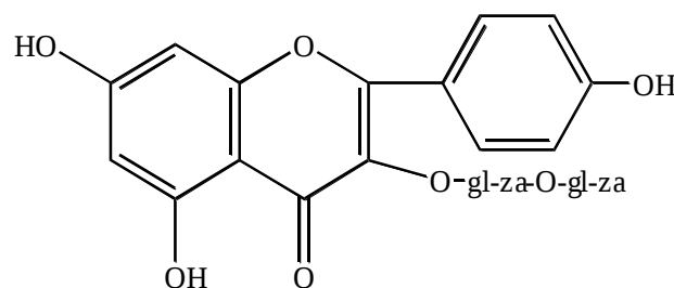
Кемефол 3-софорозид
