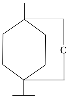
Цинеол
