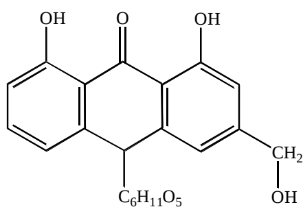
Алоэ-эмодин-антрон гликозиди
