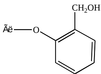
Салицин
