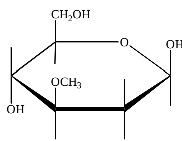
D - цимароза
