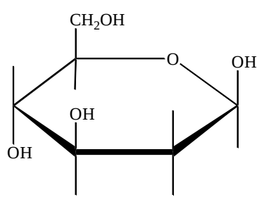
D - дигитоксоза
