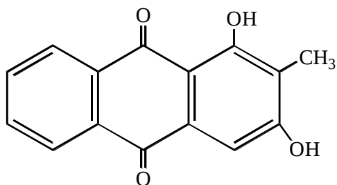
Пурпурин
