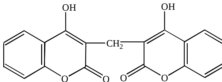
Дикумурол
