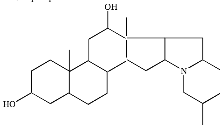
Рубимервин
