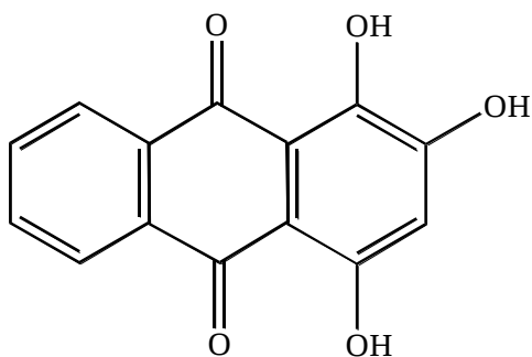
Пурпурин
