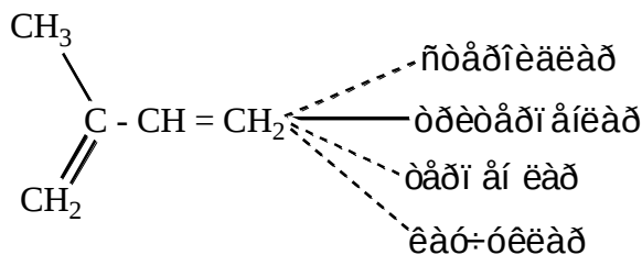
Изопрен
