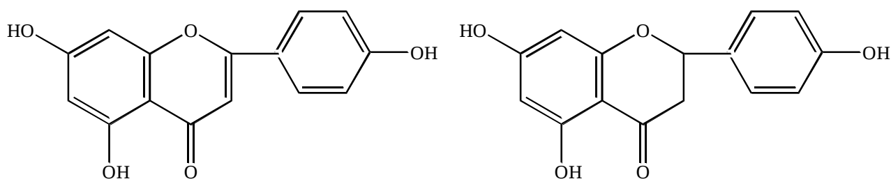
Апигенин
