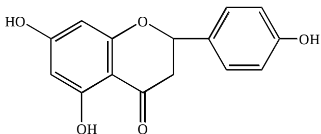
Нарингенин
