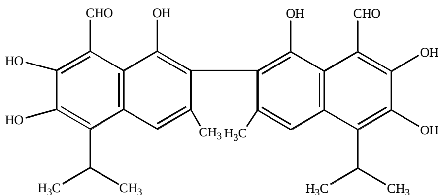
Госсипол
