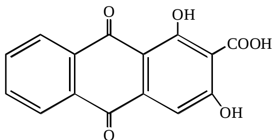
Псеудопурпурин
