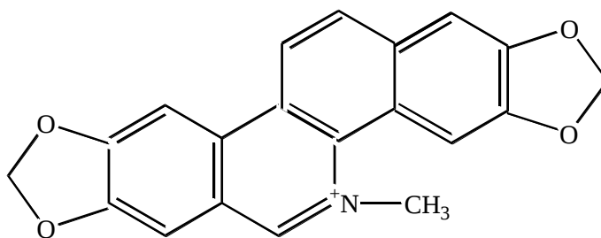
Сангвинарин
