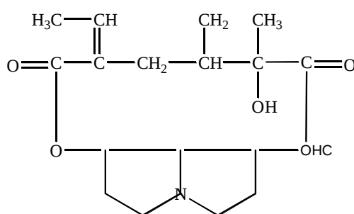
Сенецифиллин
