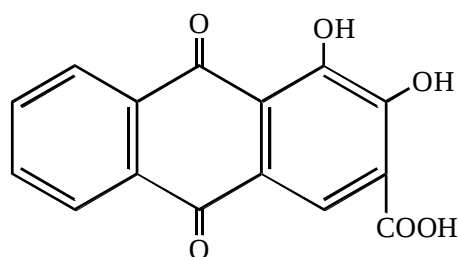
Псеудопурпурин
