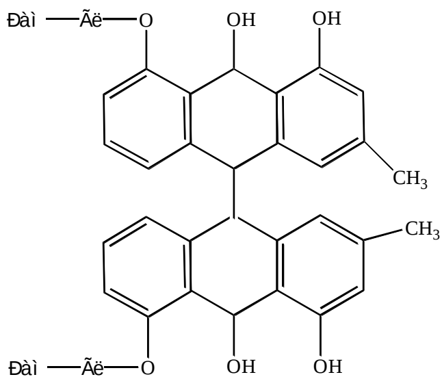
Франгуларозид
