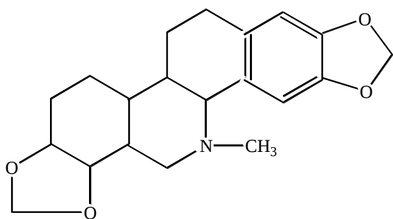
Хелидоин
