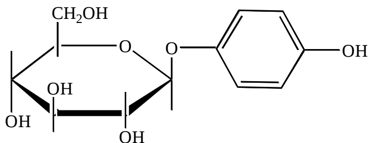
Арбутин
