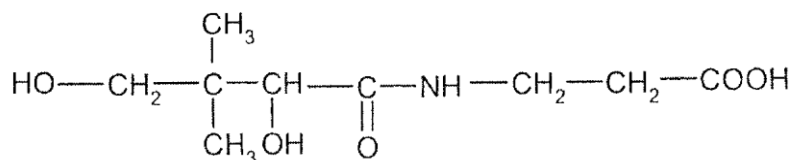
Пантотен кислота
