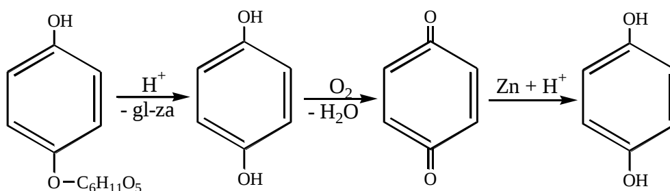
Арбутин
