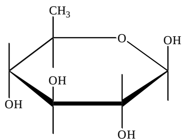
L - рамноза
