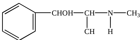
Эфедрин
