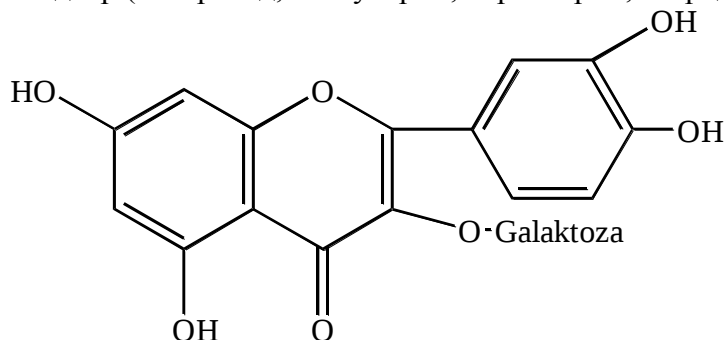
Гиперозид
