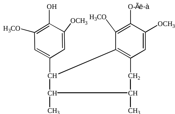
Фелигозид
