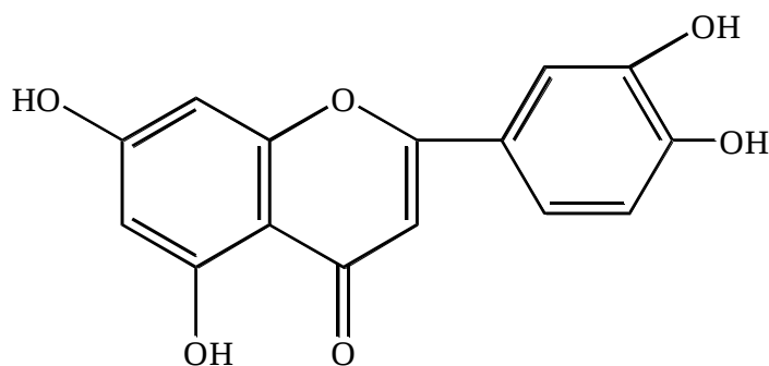
Лютеолин
