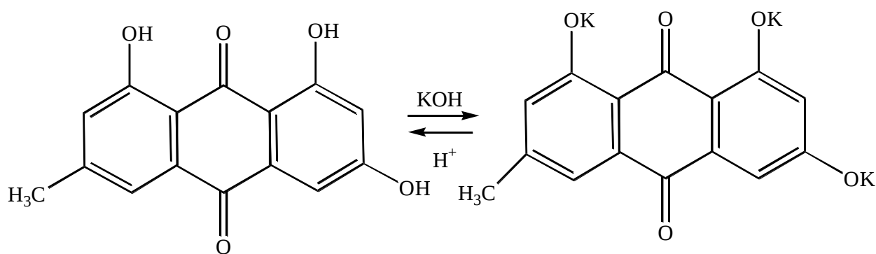
Реум эмодин
