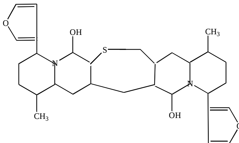
Нуфлеин
