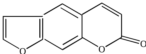
Псорален
