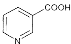
Никотин кислота
