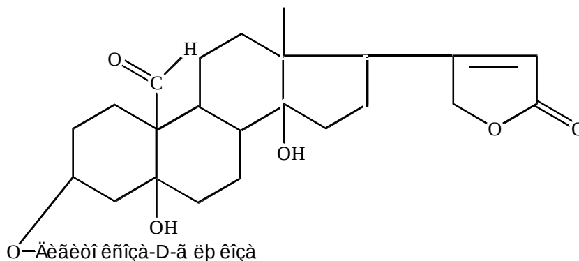
Эризимозид
