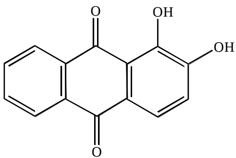
Алиаарин
