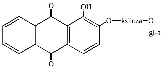
Руберитрин кислота
