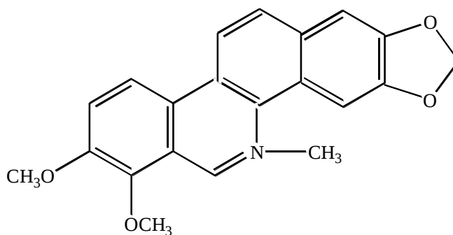
Хелеритрин
