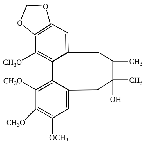
Гомизин А
