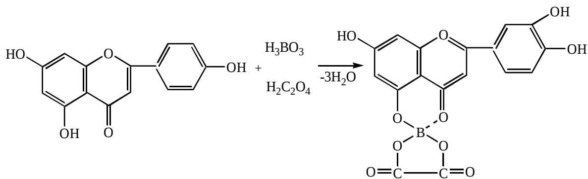
Апигенин
