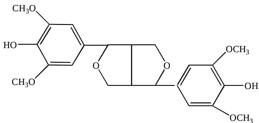
Сирингорезинол
