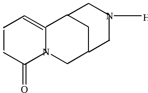
Цитизин
