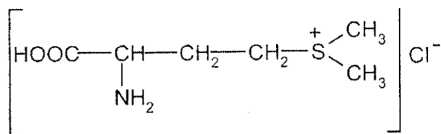
Витамин U
