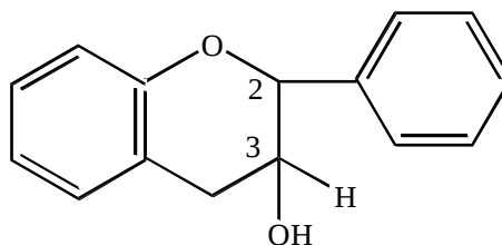
Катехин (3 - флавонол)
