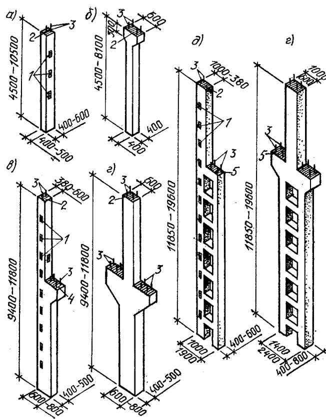
23-рasm. Ишлаб чиқариш биоларининг колонналари: а – крансиз биоларнинг четки қаторлари учун; б – крансиз биоларнинг ўрта қаторлари учун; в – кранли биоларнинг четки қаторларига мўлжалланган тўғри бурчакли колонна; г – кранли биоларнинг ўрта қаторларига мўлжалланган тўғри бурчакли колонна; д – кранли биоларнинг четки қаторларига мўлжалланган икки тармоқли колонна; е – кранли биоларнинг ўрта қаторларига мўлжалланган икки тармоқли колонна; 1 – қуйма деталар; 2 – пўлат каллак; 3 – анкер болтлар; 4 – консоль сиртидаги қуйма деталь; 5 – устун четидаги қуйма деталь
