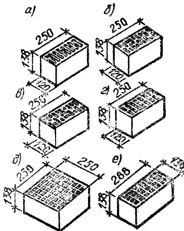
10-расм. Ичи ковак сопол тошлар: а – 7 ковакли; б – 15 ковакли; в – 21 ковакли; г – 28 ковакли; а – ковакларининг икки боши очиқ бўлган йирик блок; е – ковакларининг икки боши очиқ бўлган модуль блок.
