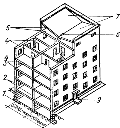
1-расм. Граждан биносининг асосий конструктив элементлари:
