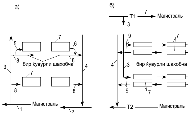
5.2-расм Пастдан (а) ва юқоридан (б) узатувчи сувли горизонтал иситиш тизимлари: 1, 2 – узатувчи ва қайтарувчи магистрал; 3 ва 4 – узатувчи ва қайтарувчи тик қукур; 5 ва 6 – узатувчи ва қайтарувчи улама; 7 – иситиш асбоблари; 8 – бир қукурли шахобча; 9 – бифиляр тармоқ.
