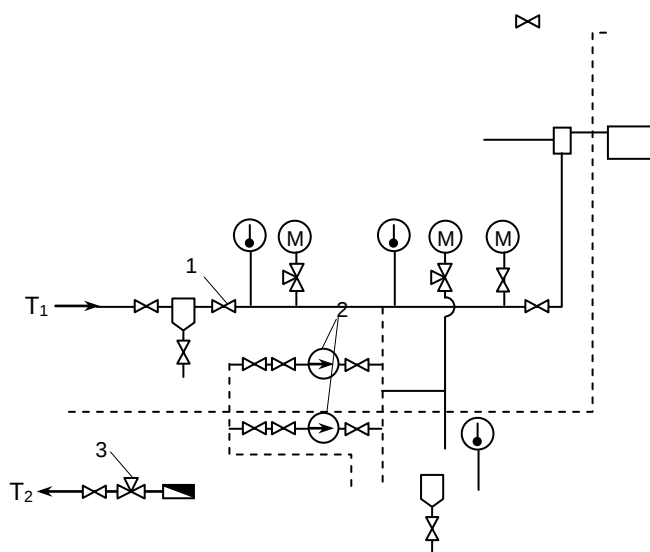
6.5-расм. Кундаланг улама қувурнинг насосга уланиш схемаси.
