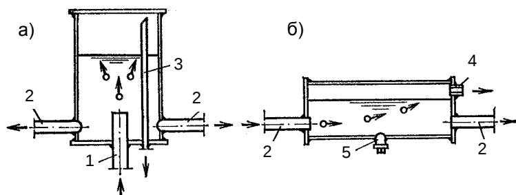
5.17-расм. Туғри оқимли ҳаво йиғувчи ускуналар: 1 – бош тик қувур; 2 – магистрал қувурлар; 3 – диаметри 15 мм бўлган ҳаво чиқарувчи қувур; 4 – диаметри 15 мм га тенг бўлган ва ҳаво чиқаришга мулжалланган муфта; 5 – диаметри 15 мм га тенг бўлган ва чиқиндини чиқаришга мулжалланган мослама.
