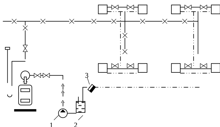
1.10-рasm. Паст босимли буғли очик иситиш тизимининг принципиал схемаси.
