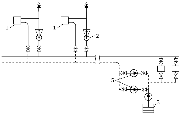
1.8-рasm. Сув-сувли туман иситиш тизимининг принципиал схемаси.
