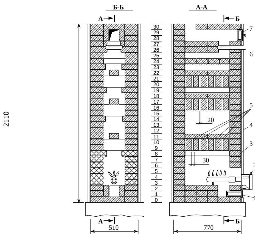
13.1-расм. Газ билан ишлайдиган АКХ-14 русумли печ: 1 - иккиламчи ҳавони бошқариш учун мослама; 2-газ маашъаласи дастаси (горелка); 3 - утхона; 4 – утхона усти ёпмаси; 5 - туғридан-туғри чиқариладиган тутун муриси; 6 – утхона ҳилини бошқарувчи учиргич; 7-ярим зич ёпилган эшикча.
