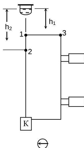
6.11-расм. Кенгайтирувчи идишнинг насослар ёрдамида ишловчи иситиш тизимига уланиш схемаси.
