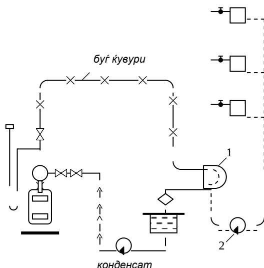
1.11-расм. Буғ-сувли иситиш тизимининг принципиал схемаси
