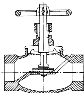
5.14-расм. Туғри шпинделлик жумрак - ТШЖ
