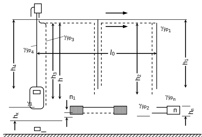
7.9-расм. Турар жой биноларидаги иситиш тизимининг узатувчи ва тескари магистраль қувурларининг шип тагида урнатилиши.
