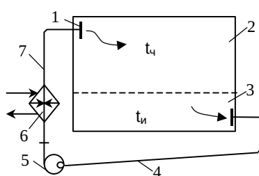
1.13-расм. Марказлаштирилган ҳаво иситувчи қурилманинг схемаси: 1 – ҳаво тарқатувчи панжара; 2 – иситиладиган хона; 3 – ишчи майдон; 4 – қайтувчи ҳаво қувури; 5 – ҳаво сургич паррак; 6 – калорифер; 7 – иссиқ ҳаво қувури.
