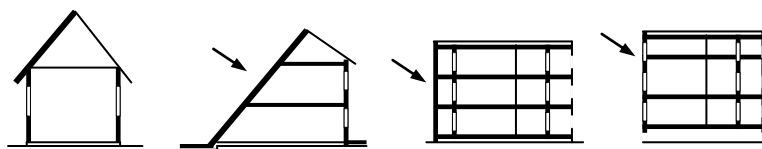
15.6-расм. Гелио қабул қилувчи қурилмаларнинг схемалари.
