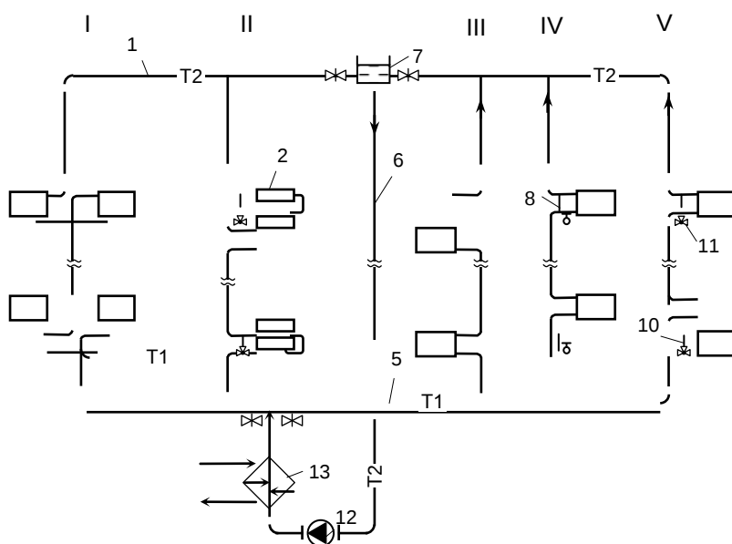
6.8, б-расм. Қуйидан тақсимланувчи бир қувурли ва «П» ҳарфи шаклидаги тиргаклари турли конструкцияли тик қувурли иситиш тизимлари: I - туғри оқимли тик қувур; II ва III силжитилган ва охири "П" шаклида уланган тик қувур; IV-V - туғри оқимли бошқарилувчи тик қувур.
