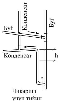
9.3-расм. Конденсатни олиб чиқариш учун ўрнатилган сифтмоқ
