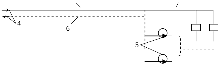
1.7-рasm. Туман сувли иситиш тизимининг принципиал схемаси.
