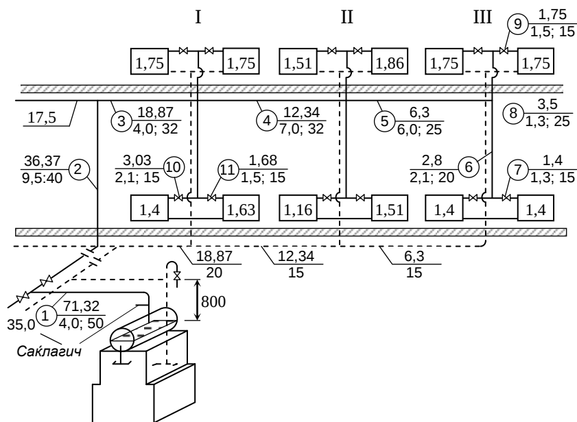
9.11–расм. Паст босимли буғ билан иситиш тизимининг ёпик системасининг ҳисобий схемаси.
