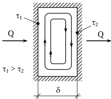
2.2-расм. Буш ҳаво қатламининг қалинлиги \delta бўлиб, икки ён сирт ҳарорати \tau_1 , \tau_2 , бунда \tau_1 > \tau_2 .
