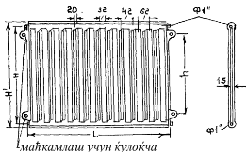
4.13.-расм. Қуй- ма пўлат туника- дан ясалган радиатор
