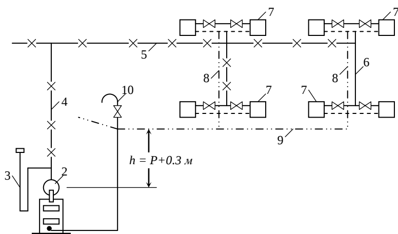
1.9-расм. Паст босимли ёпик ҳолатдаги буғли иситиш тизимининг принципаи схемаси.
