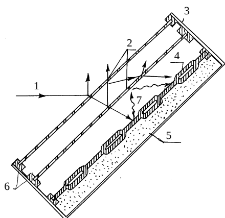
15.9-расм. Ясси қуёш коллектори. 1 – қуёш нурлари; 2 – шишали юза; 3 – коллектор қобиғи (корпуси); 4 – иссиқлик қабул қилувчи (пластина); 5 – иссиқликдан изоляцияловчи қатлам; 6 – шишани ўрнатиш учун мослама; 7 – иссиқлик қабул қилувчини узун тўлқинли нурланиши.
