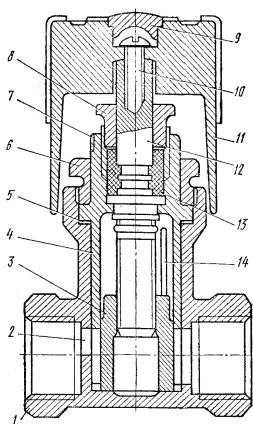
5.11-расм. Икки томонлама бошқарувчи жумрак – ИБЖ: 1 – корпус; 2 – бошқарувчи туйнук; 3 – шиббер; бурувчи втулка; 5 – прокладка; 6 – маҳкамловчи гайка; 7 – втулка рискаси; 8 – салник гайкаси; 9 – қопқоқ; 10 – винт; 11– даста; 12 – резбали шпиндел; 13 – санликли жипслагич; 14 – втулкадаги паз.
