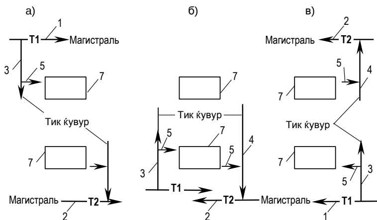
5.1-расм. Иситиш марказидан вертикал иссиқлик тарқатиш тизими: а – юқоридан тарқатувчи; б – пастдан узатувчи; в – «тунтарилган» вертикал қукурларда сув ҳаракати.
