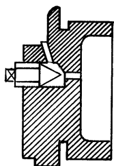
4.19-расм. Радиатор тикинига ўрнатиловчи ғаво чиқариш жумраги.
