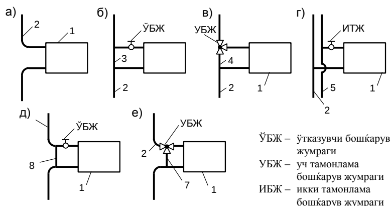
5.7-расм. Бир (а-в) ва икки (г) қувурли вертикал иситиш тизимида қувурларнинг иситиш асбобларига бир томонлама уланиши:
