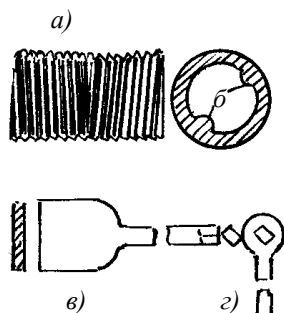
4.2-расм. Ниппель ва радиатор секцияларини бирлаштириш учун қўлланиладиган калит: а – ниппель; б – ниппелни бураб юргизувчи кўндаланг валик; в – радиатор учун калит; г – ёққалик калит.
