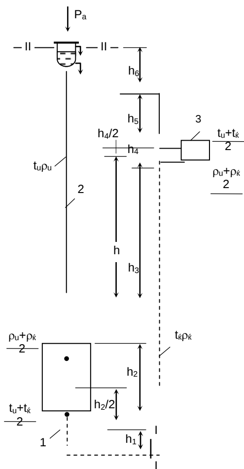
7.2-расм. Табиий босим
