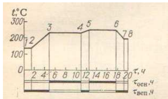
Расм – 2. Алкид синтезида фтал ангидридини қаттиқ ҳолда юклангандаги ва глицин билан ўсимлик мойларини олидндан иситиб олинмаган ҳолатидаги харорат-вақт режими:
